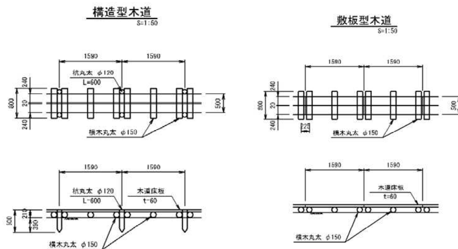
図-9.1 木道の構造図（サロベツ原生花園園地跡地の事例）
