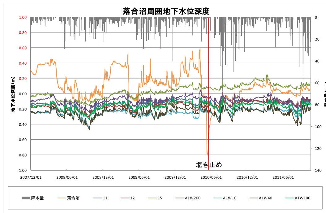
図Ⅲ. 6. 4 落合沼周囲の地下水位変動 (GL 以下深度)
