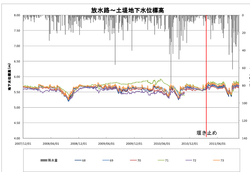
図Ⅲ. 6. 16 放水路～土堤の間の地下水位変動（標高）
