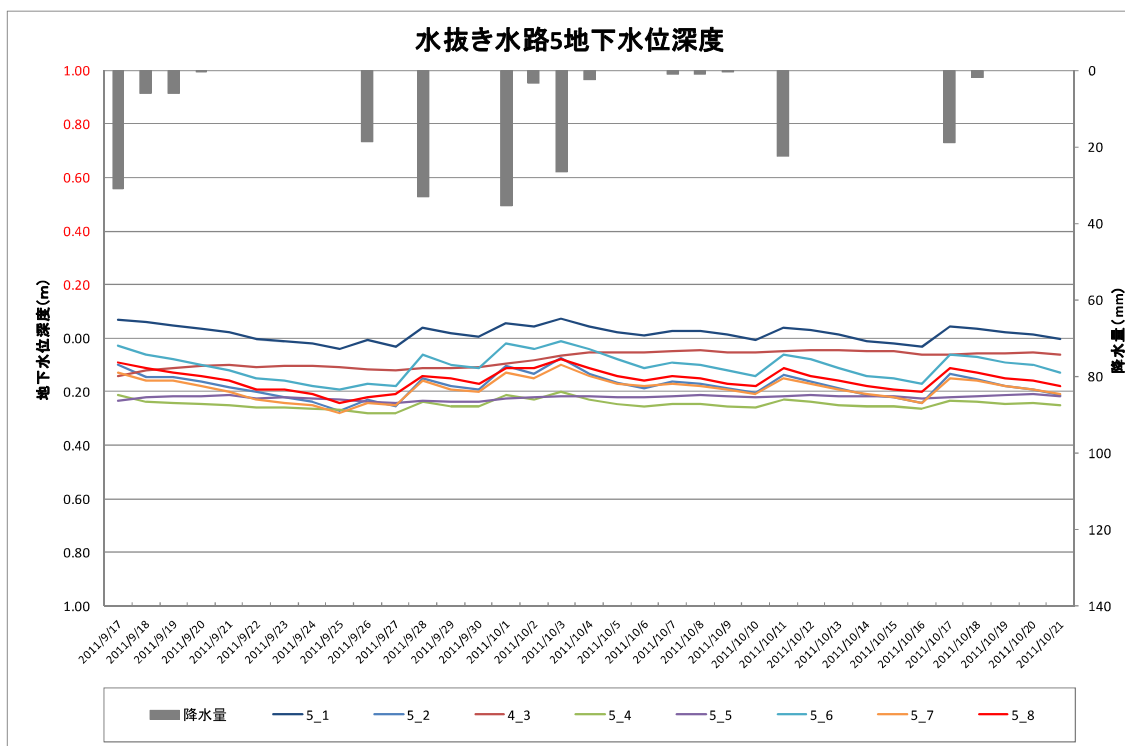
図Ⅱ. 6. 40 水抜き水路 5 の植物調査地点の水位変動
