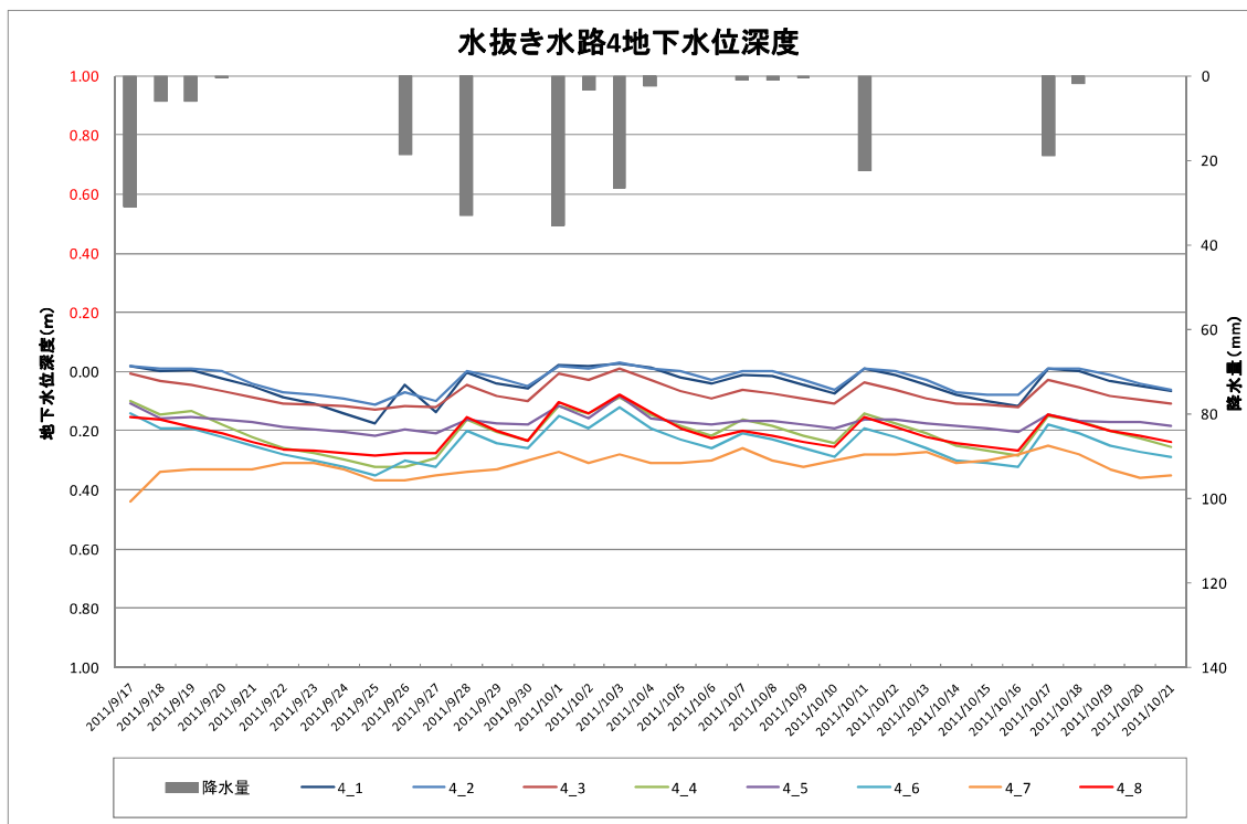
図Ⅱ. 6. 38 水抜き水路 4 の植物調査地点の水位変動
