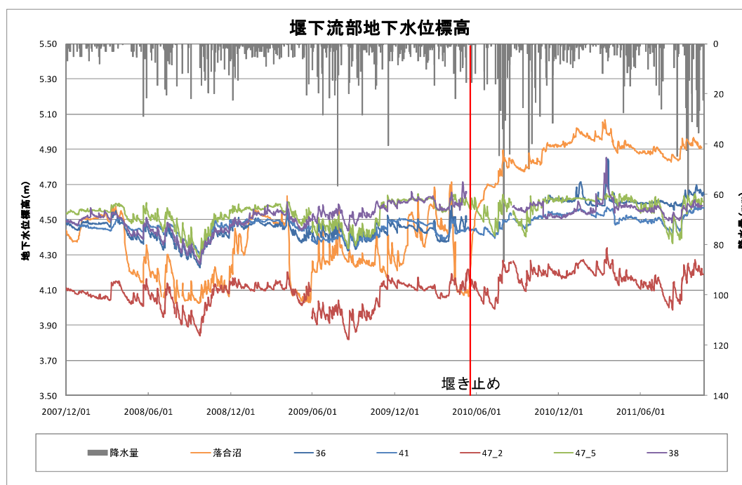
図Ⅲ. 6. 9 堰下流部の地下水位変動（標高）
