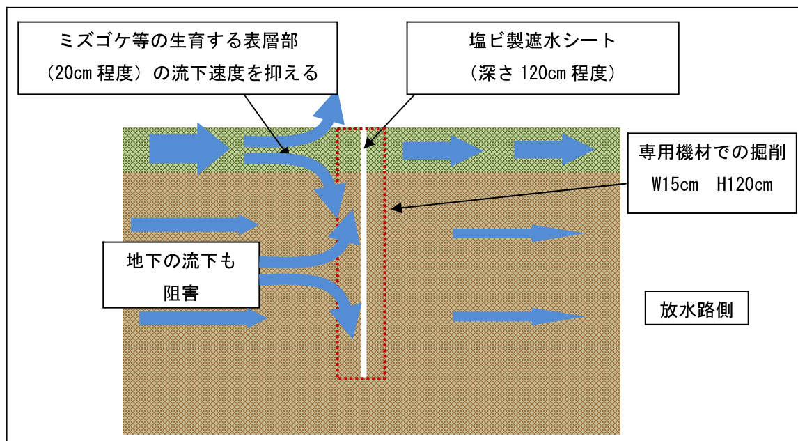
図Ⅱ.6.52 塩ビ遮水シート敷設模式断面
