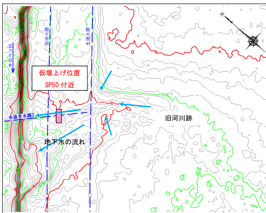
図Ⅱ.6.43 水抜き水路3の仮堰上げ位置（平面図）
