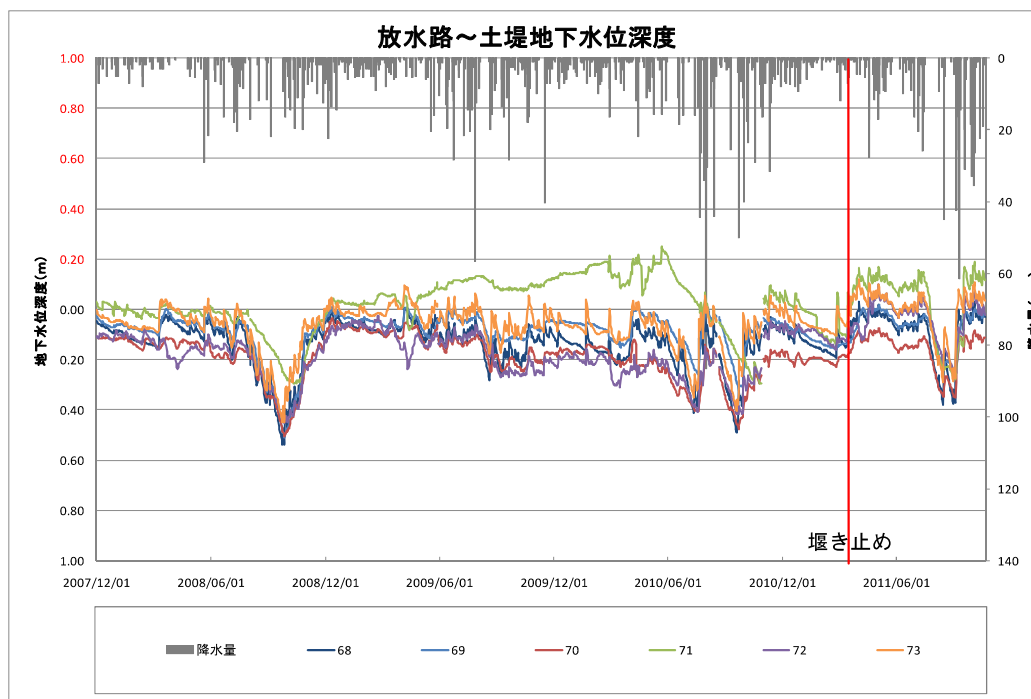
図Ⅲ. 6. 15 放水路～土堤の間の地下水位変動（GL 以下深度）
