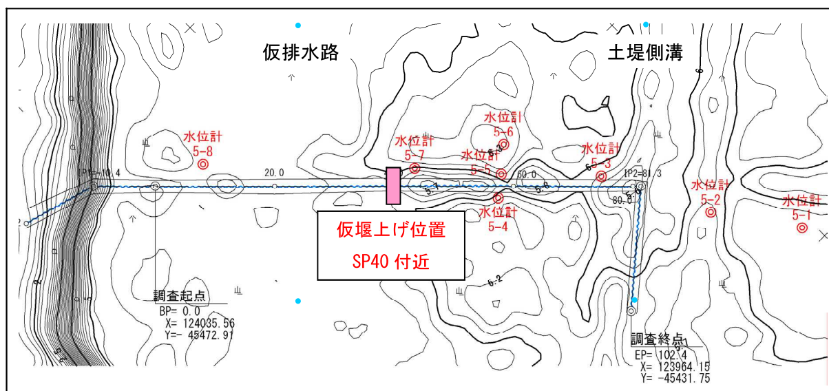
図 II. 6. 47 水抜き水路 5 の仮堰上げ位置 (平面図)
