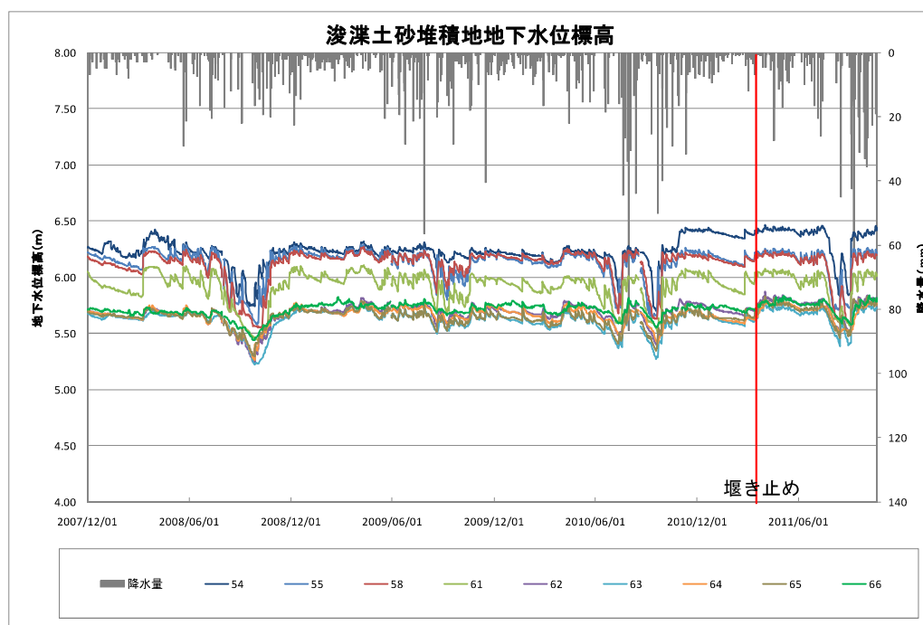
図Ⅲ. 6. 14 落合沼周囲の地下水位変動（標高）
