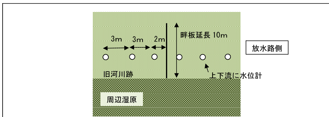
図 II. 6. 58 試験施工案 A 配置模式平面図
