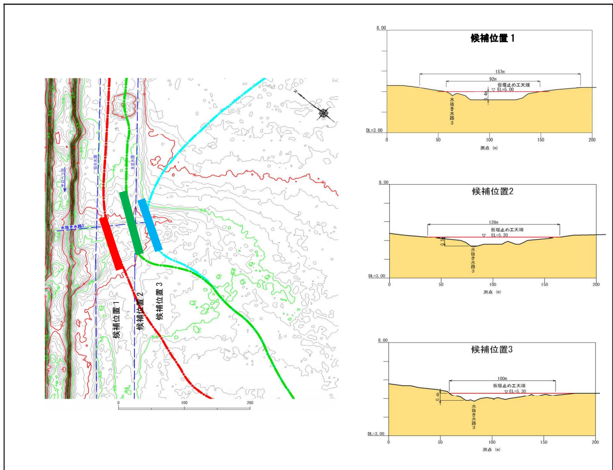
図Ⅱ. 6. 50 水抜き水路 3 および旧河川跡 堰き止め位置の比較
