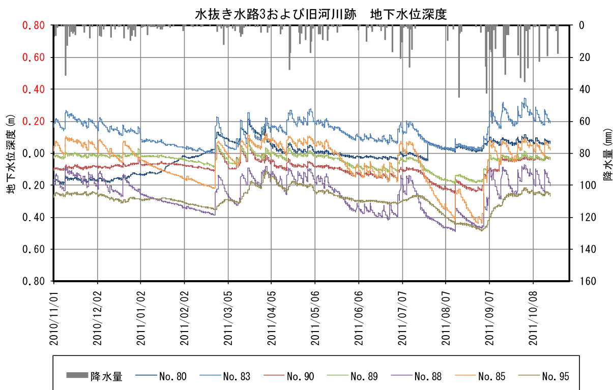
図Ⅱ. 6. 36 水抜き水路 3 の植物調査地点の水位変動
