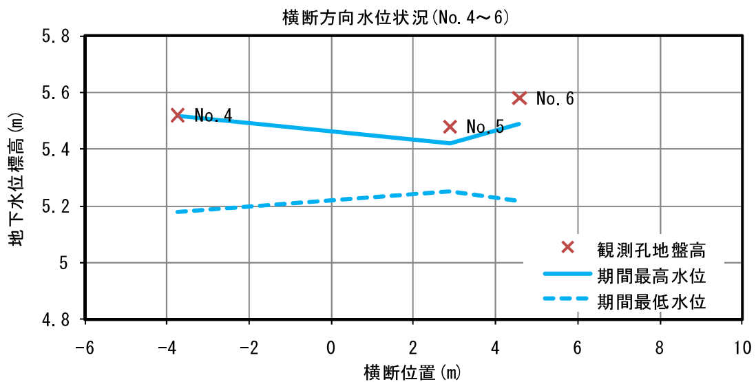
図Ⅱ. 6. 31 水抜き水路 4 の地下水位標高
