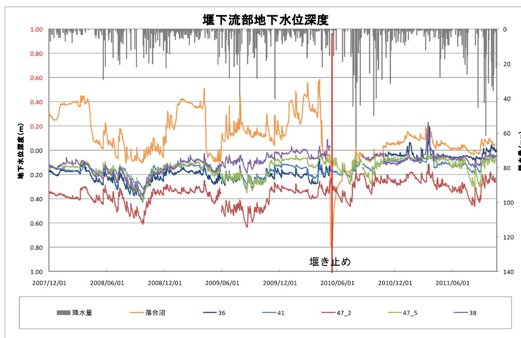
図Ⅲ. 6. 8 堰下流部の地下水位変動（GL 以下深度）
