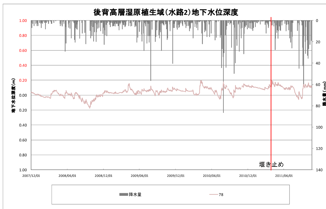
図Ⅲ. 6. 11 後背高層湿原植生域の地下水位変動（GL 以下深度）
