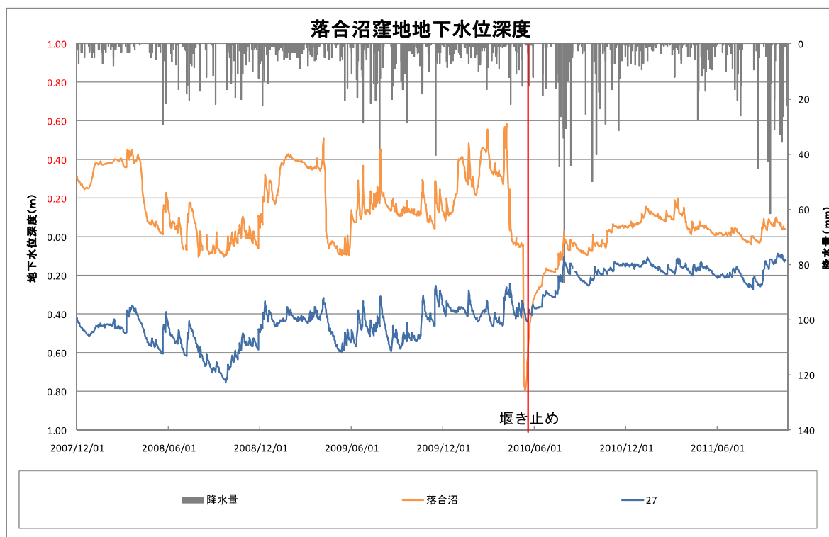
図Ⅲ. 6. 6 落合沼窪地の地下水位変動（GL 以下深度）
