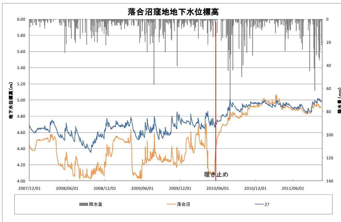
図Ⅲ. 6. 7 落合沼窪地の地下水位変動（標高）
