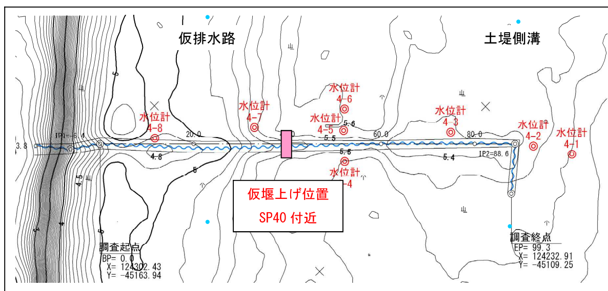
図Ⅱ.6.45 水抜き水路 4 の仮堰上げ位置（平面図）
