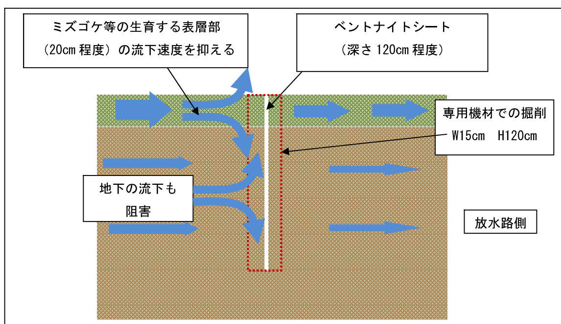
図 II. 6. 53 ベントナイト遮水シート敷設模式断面
