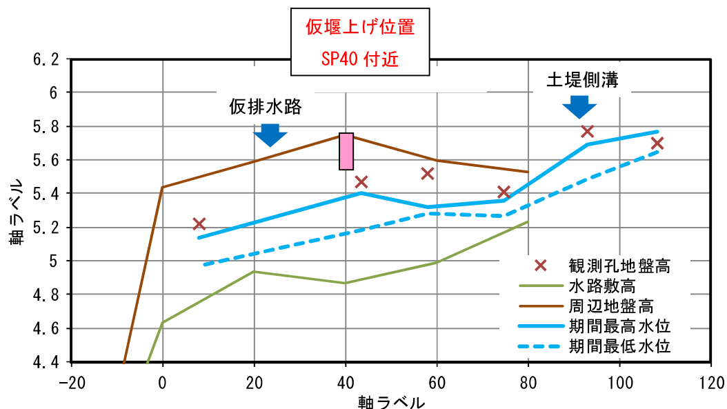
図 II. 6. 46 水抜き水路 5 の仮堰上げ位置 (縦断面図)
