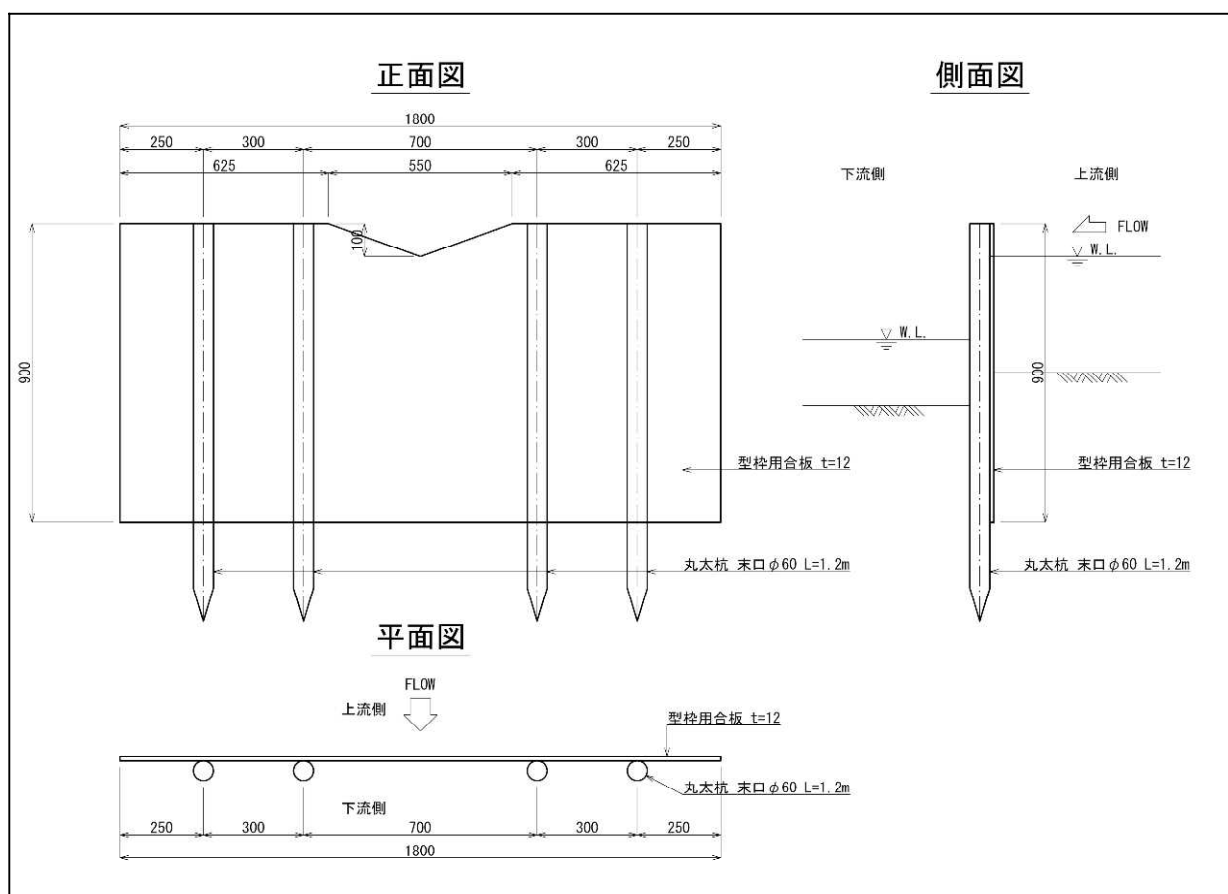
図 II.6.41 仮堰の構造
