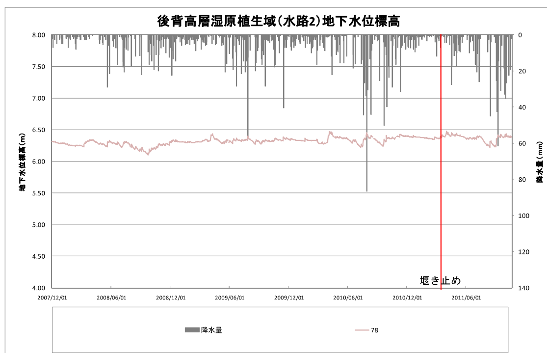
図Ⅲ. 6. 12 後背高層湿原植生域の地下水位変動（標高）
