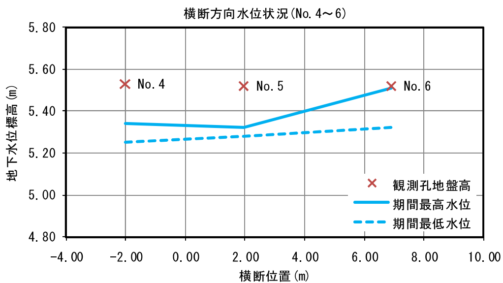
図Ⅱ. 6. 33 水抜き水路 5 の地下水位標高
