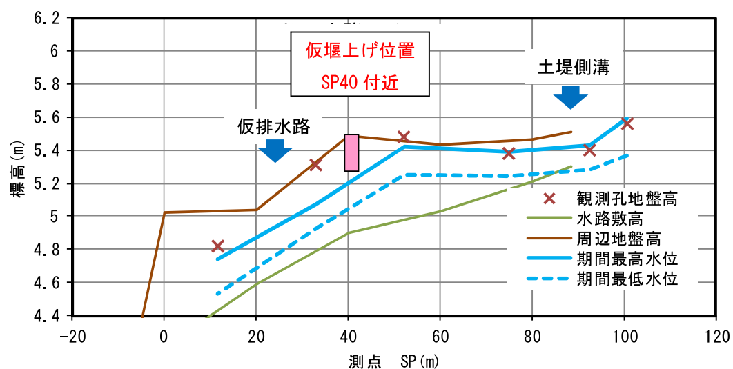
図Ⅱ.6.44 水抜き水路 4 の仮堰上げ位置（縦断図）
