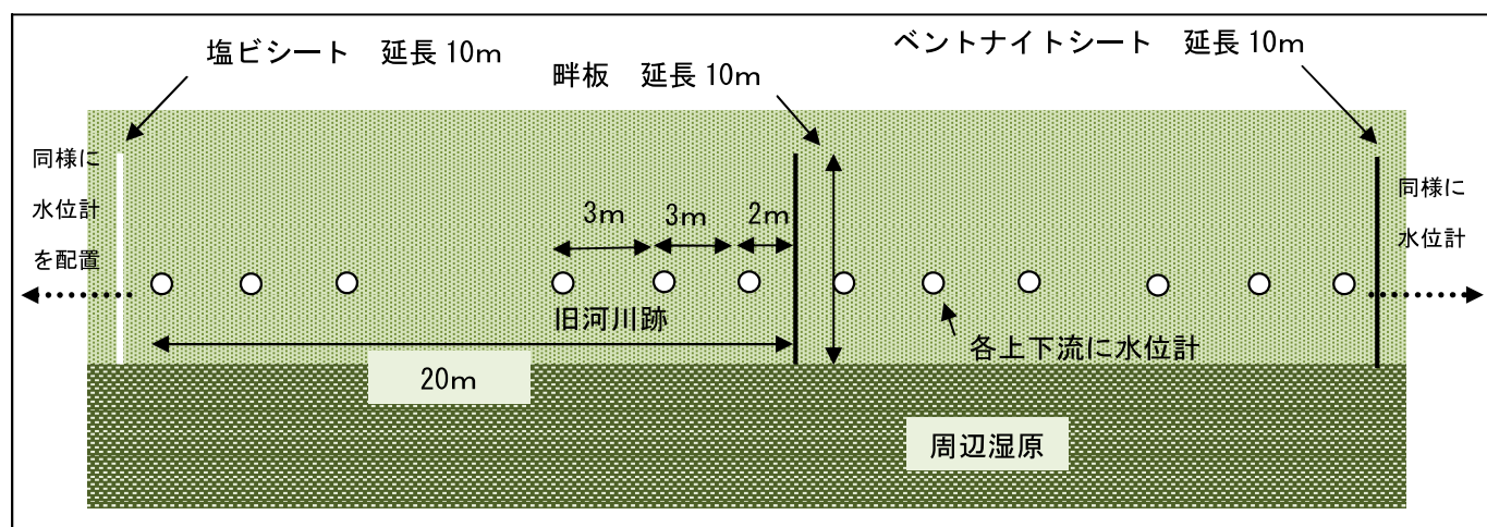
図 II. 6. 59 試験施工案 B 配置模式平面図
