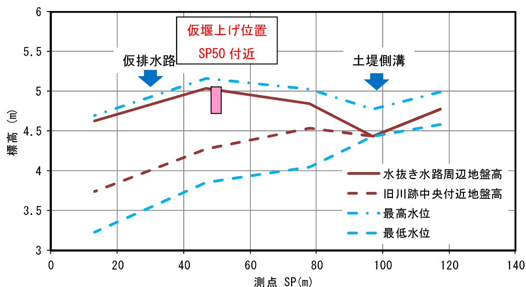
図Ⅱ.6.42 水抜き水路3の仮堰上げ位置（縦断図）
