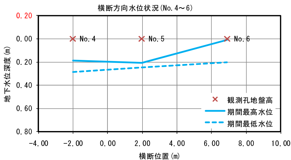
図Ⅱ. 6. 32 水抜き水路 5 の地下水位深度
