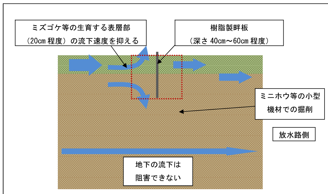
図 II.6.51 畔板敷設模式断面
