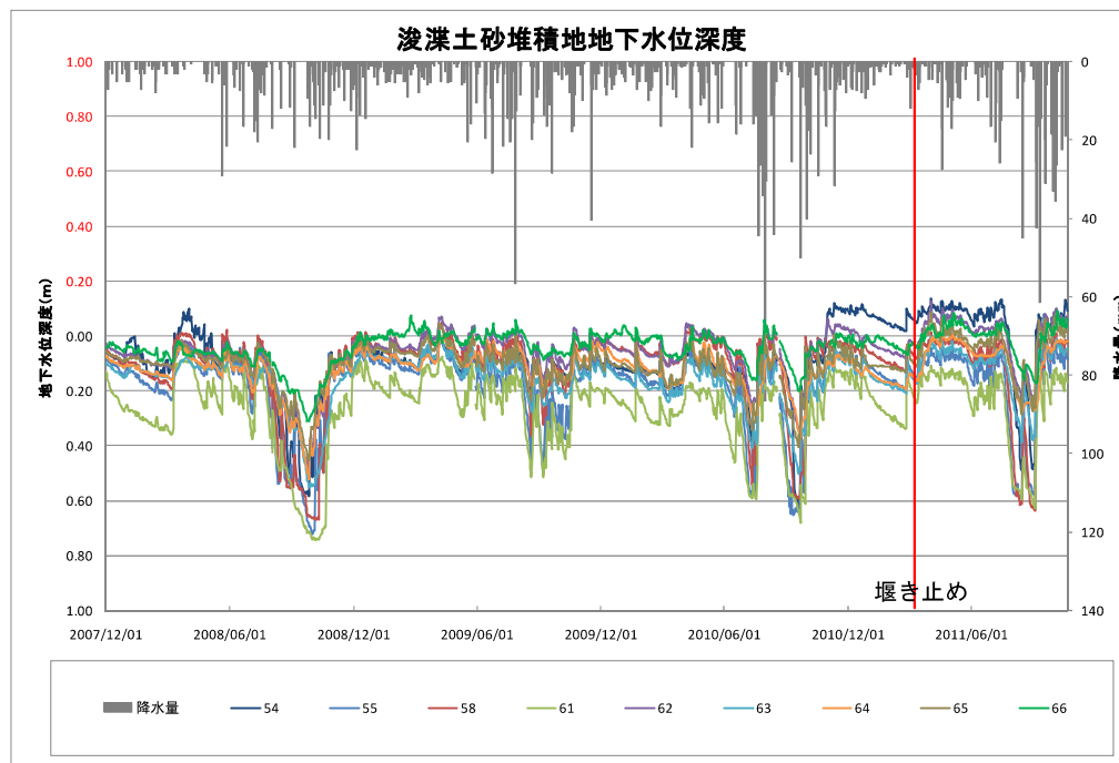
図Ⅲ. 6. 13 落合沼周囲の地下水位変動（GL 以下深度）
