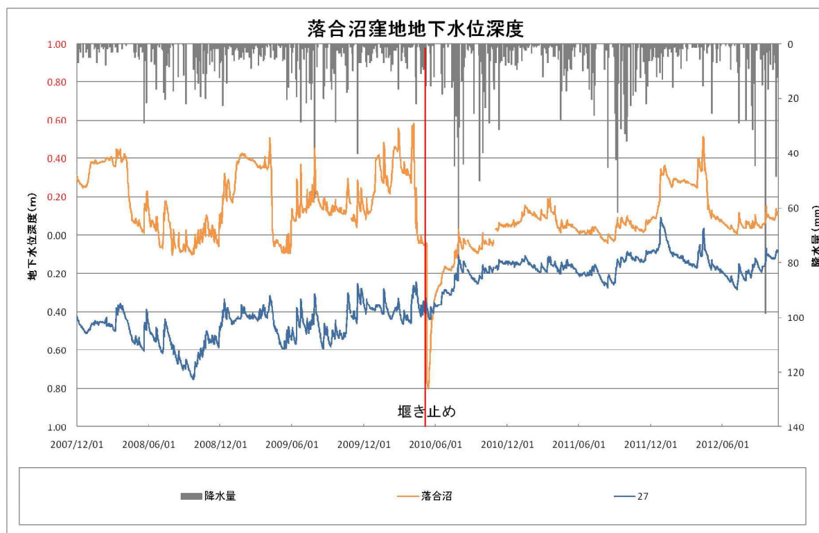
図Ⅲ. 6. 7 落合沼窪地の地下水位変動（GL 以下深度）
