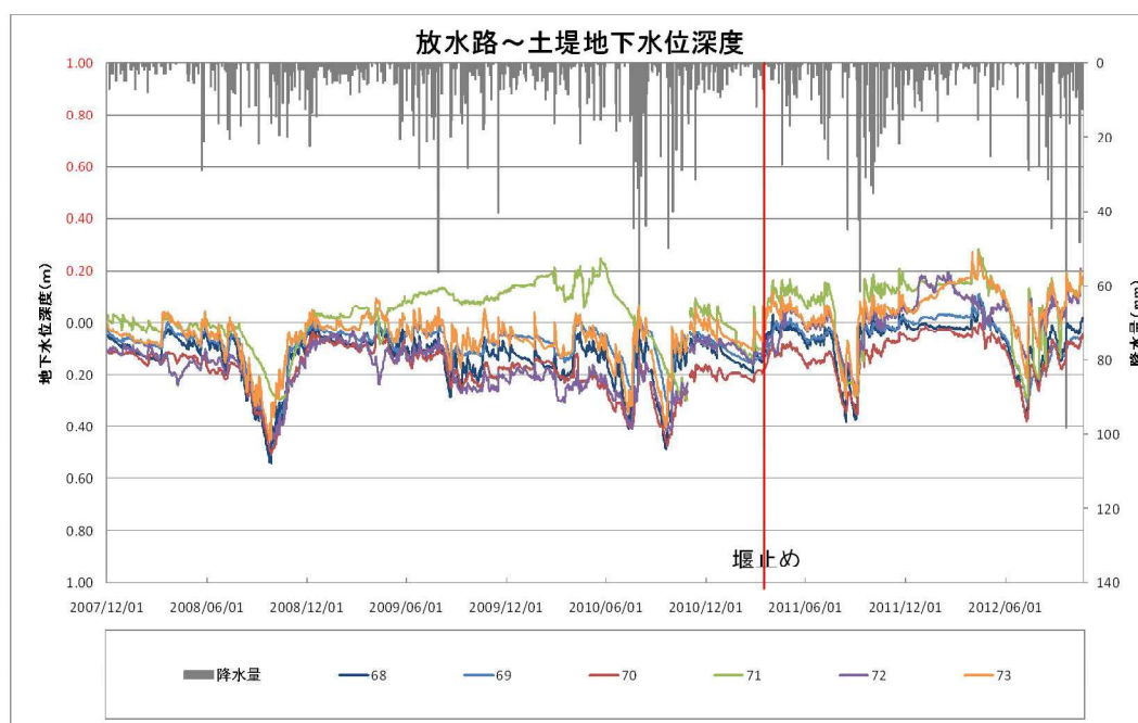
図Ⅲ. 6. 16 放水路～土堤の間の地下水位変動（GL 以下深度）
