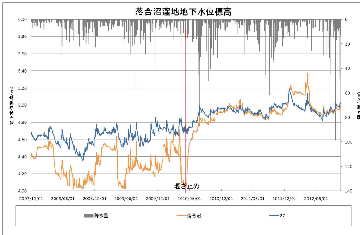
図Ⅲ. 6. 8 落合沼窪地の地下水位変動（標高）
