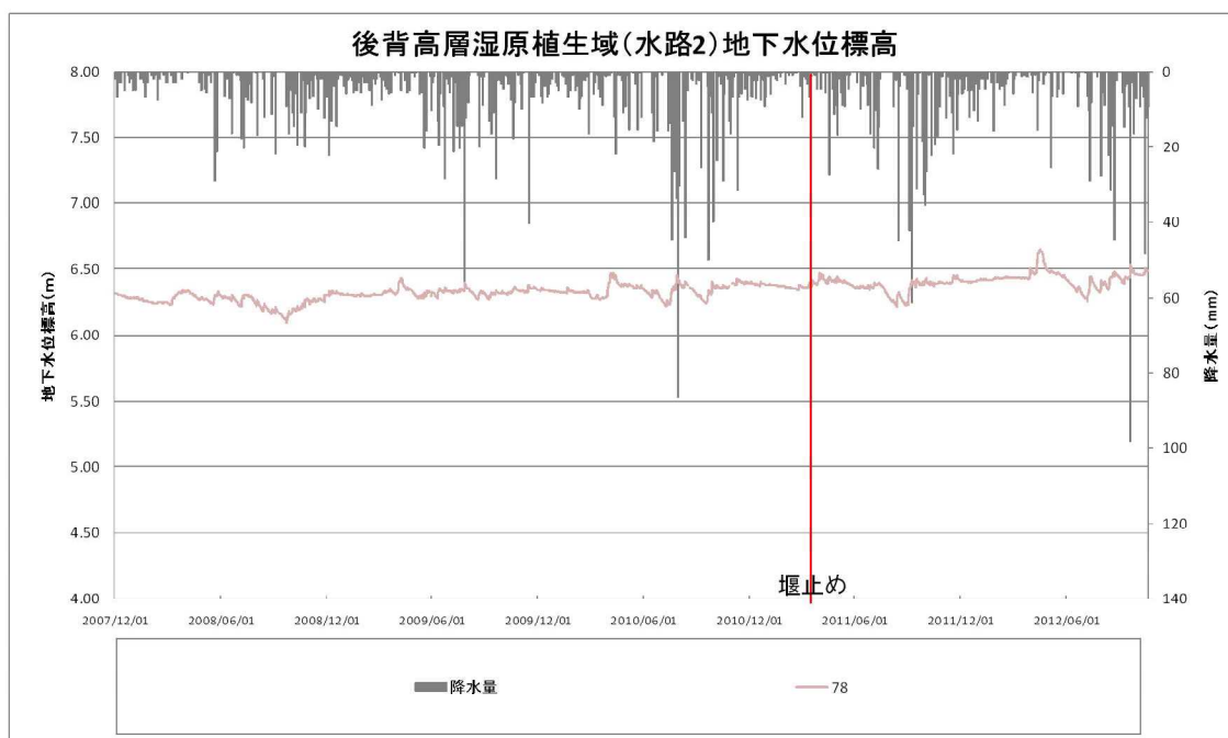
図Ⅲ. 6. 12 後背高層湿原植生域の地下水位変動（GL 以下深度）
