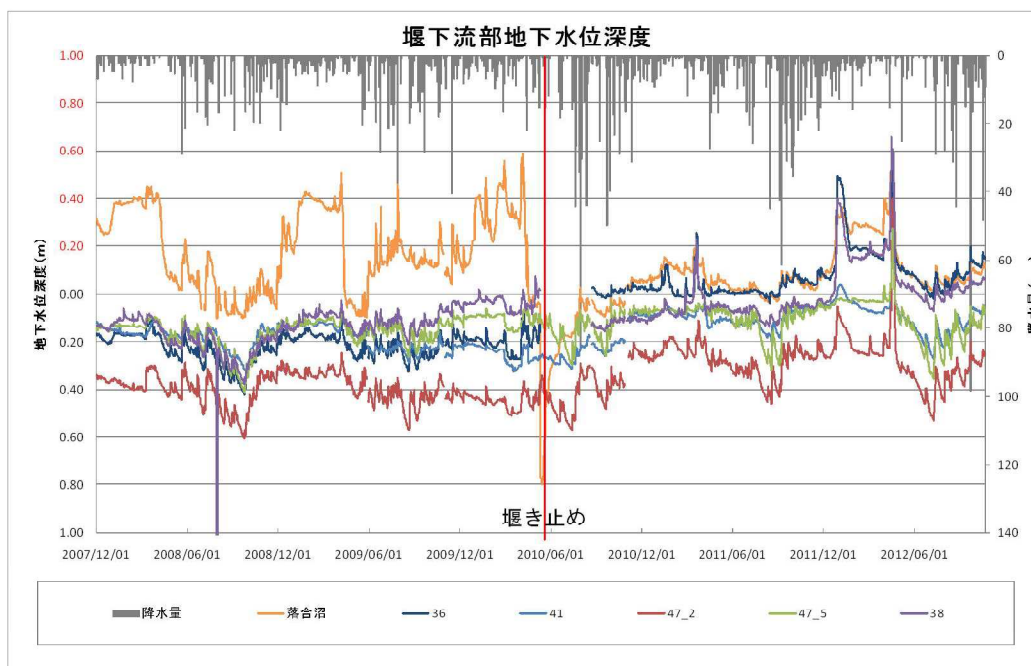
図Ⅲ. 6. 9 堰下流部の地下水位変動（GL 以下深度）
