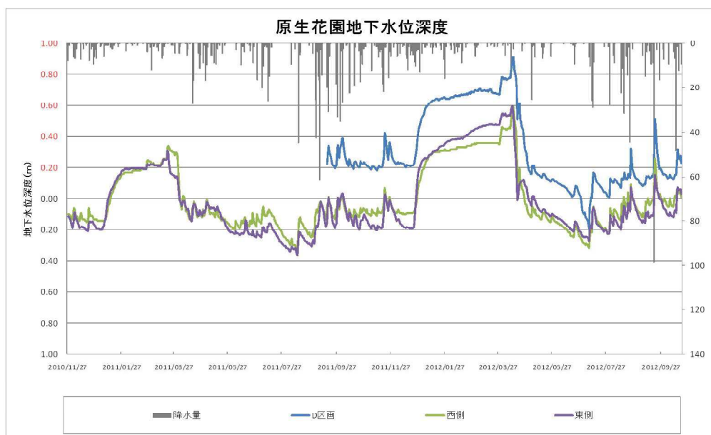
図IV. 6.2 原生花園園地跡地周辺の地下水位変動（GL 以下深度）
