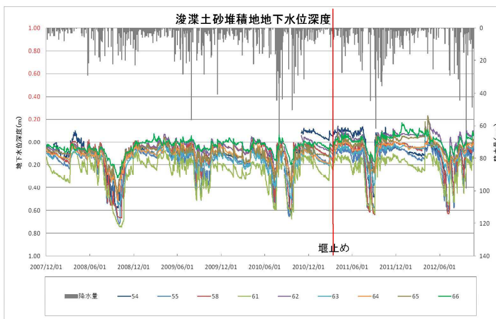
図Ⅲ. 6. 14 落合沼周囲の地下水位変動（GL 以下深度）
