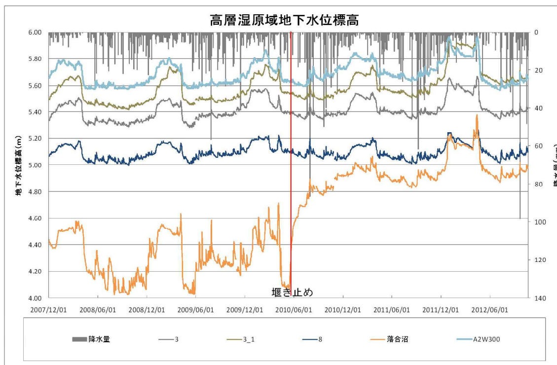
図Ⅲ. 6. 3 高層湿原植生域の地下水位変動（標高）
