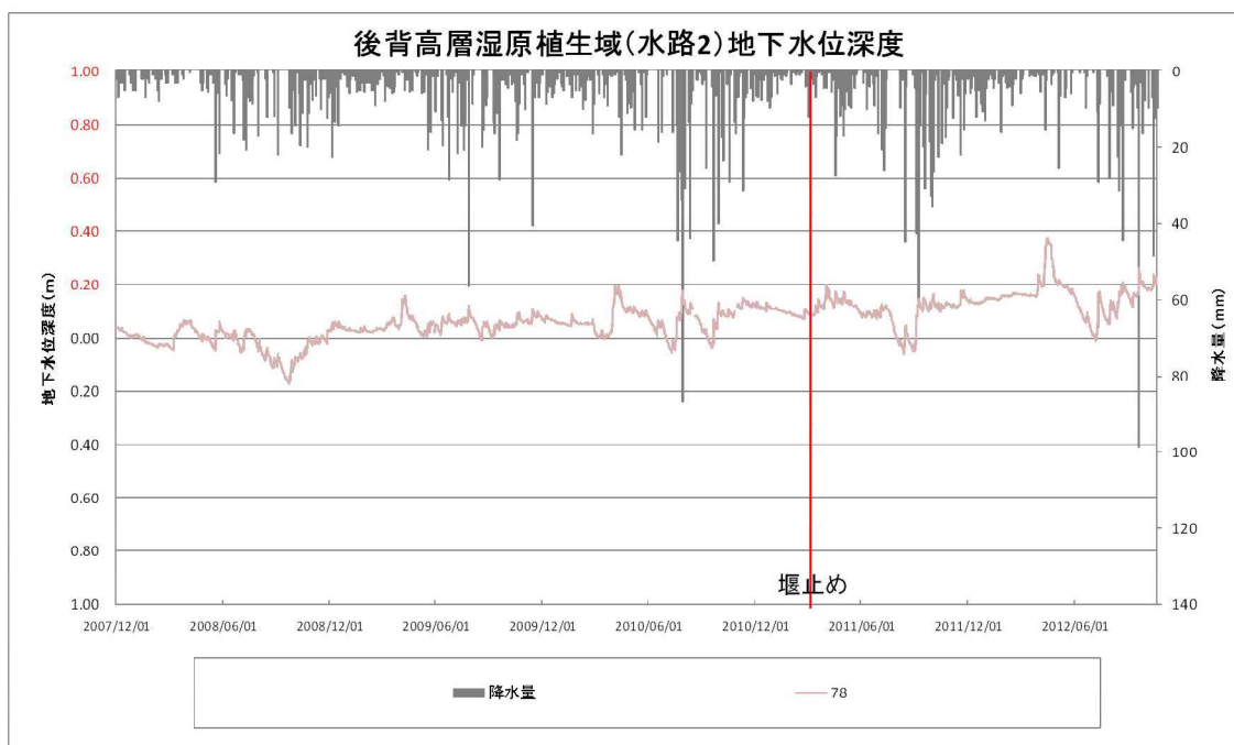
図Ⅲ. 6. 13 後背高層湿原植生域の地下水位変動（標高）
