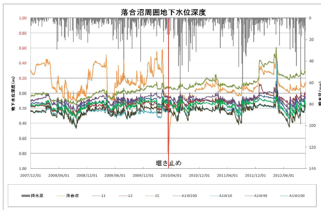
図Ⅲ. 6. 4 落合沼周囲の地下水位変動（GL 以下深度）
