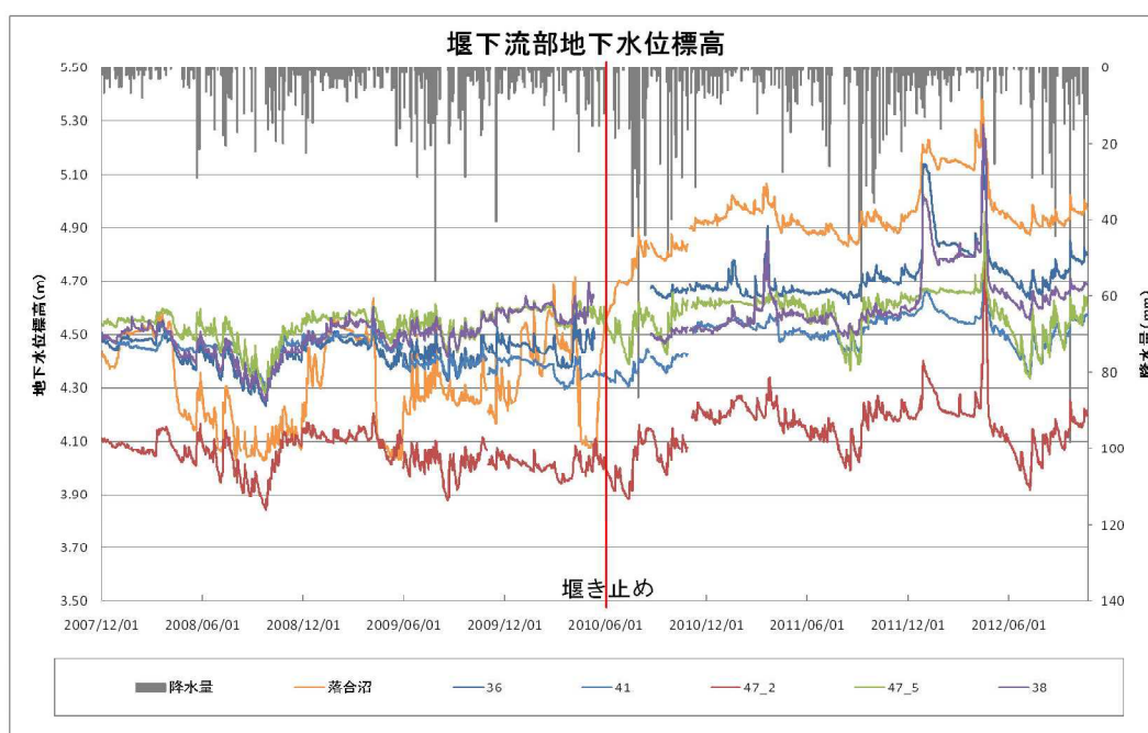
図Ⅲ. 6. 10 堰下流部の地下水位変動（標高）
