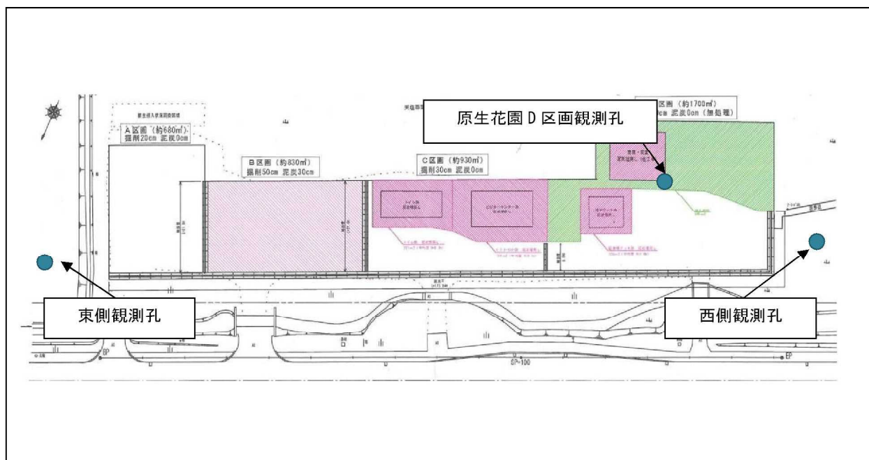
図IV. 6. 1 原生花園園地跡地地下水観測孔位置
