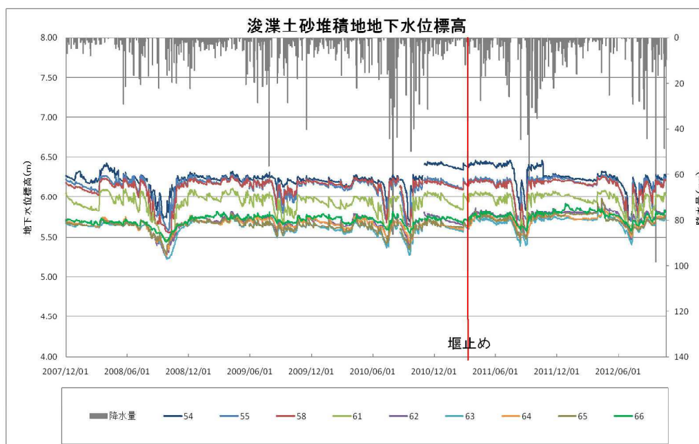
図Ⅲ. 6. 15 落合沼周囲の地下水位変動（標高）
