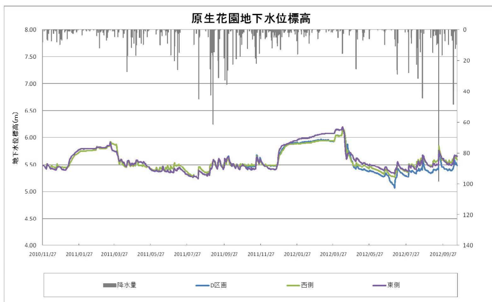
図IV. 6.3 原生花園園地跡地周辺の地下水位変動（標高）
