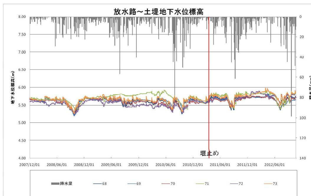
図Ⅲ. 6. 17 放水路～土堤の間の地下水位変動（標高）
