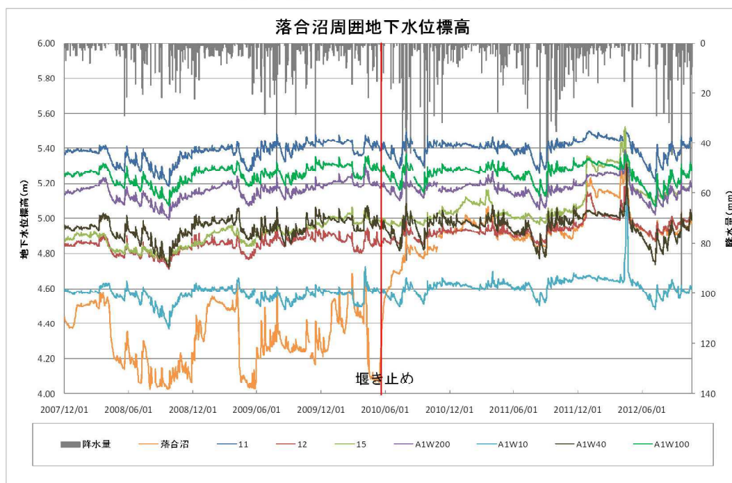
図Ⅲ. 6. 5 落合沼周囲の地下水位変動（標高）
