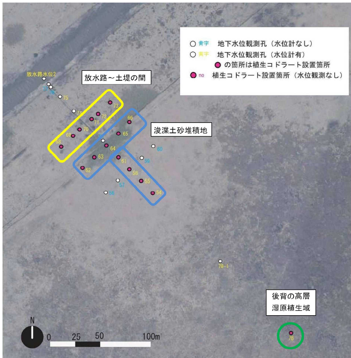
図Ⅲ. 6. 11 対象モニタリング地点
