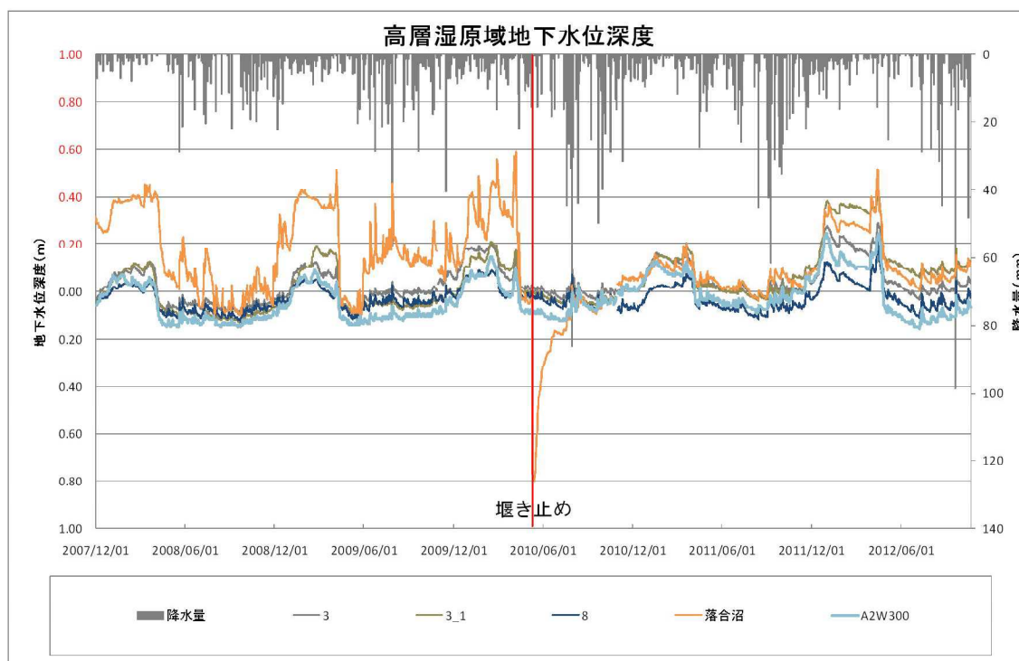
図Ⅲ. 6. 2 高層湿原植生域の地下水位変動（GL 以下深度）
