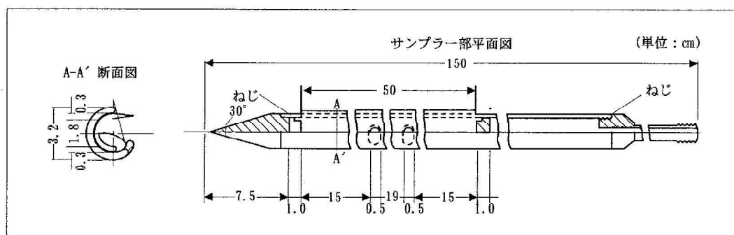
図Ⅱ.4.3 ピートサンプラーの概念図
