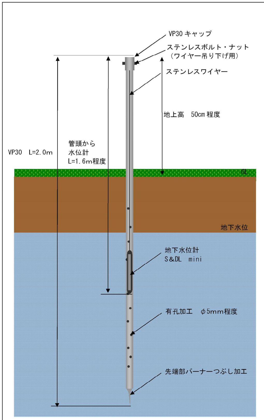
図Ⅱ.4.4 地下水位計の設置状況
