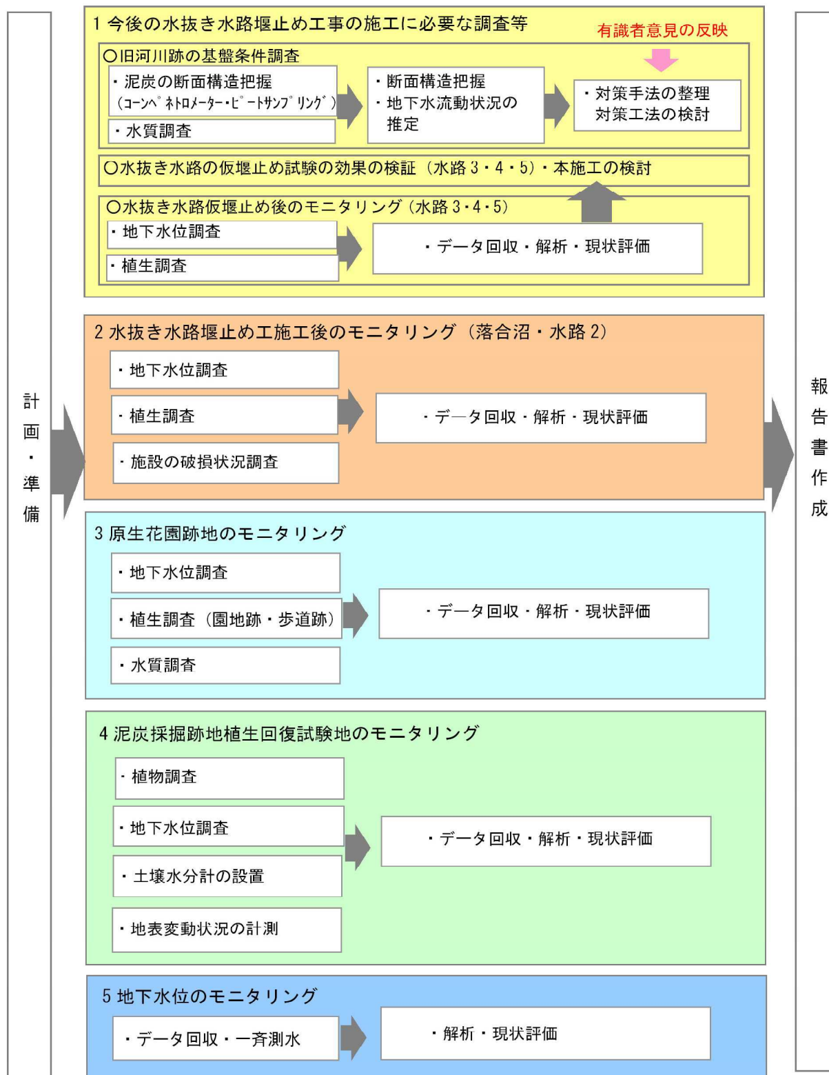
図 I.4.1 業務フロー
