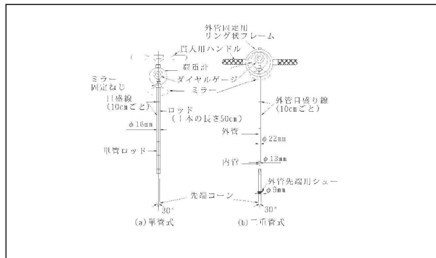
図 II. 4. 2 コーンペネトロメーター試験器具概要図
