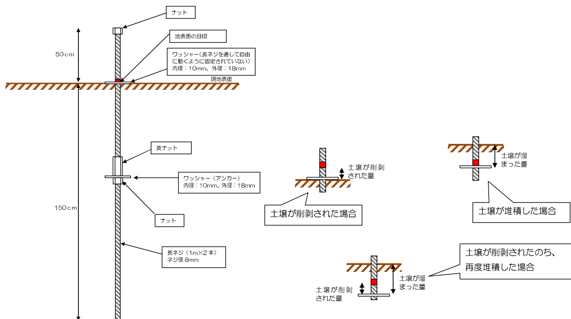
図 1.6.12 地表変動計測手法の概要
