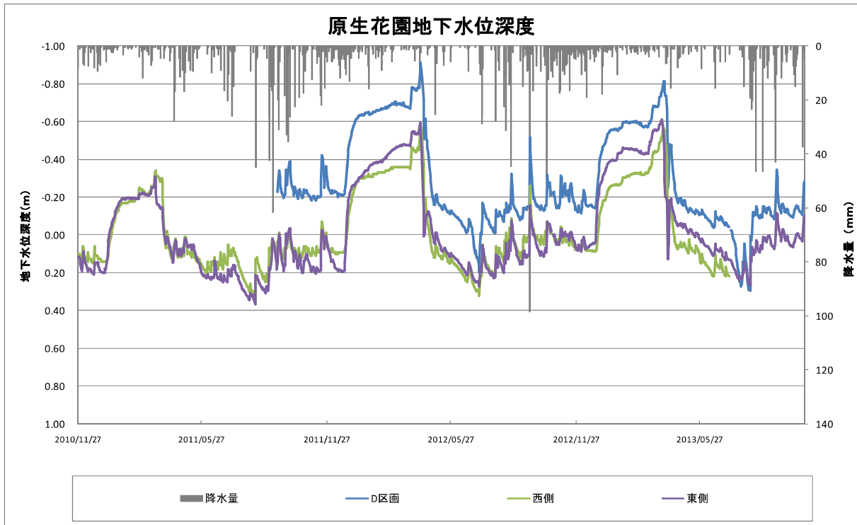
図2.5.39 原生花園園地跡地の地下水位深度
