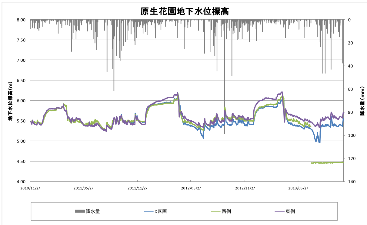
図2.5.38 原生花園園地跡地の地下水位標高
