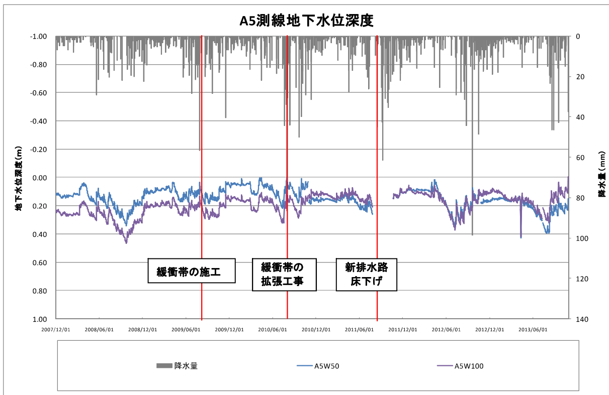
図2. 5. 28 A5 測線の地下水位深度
