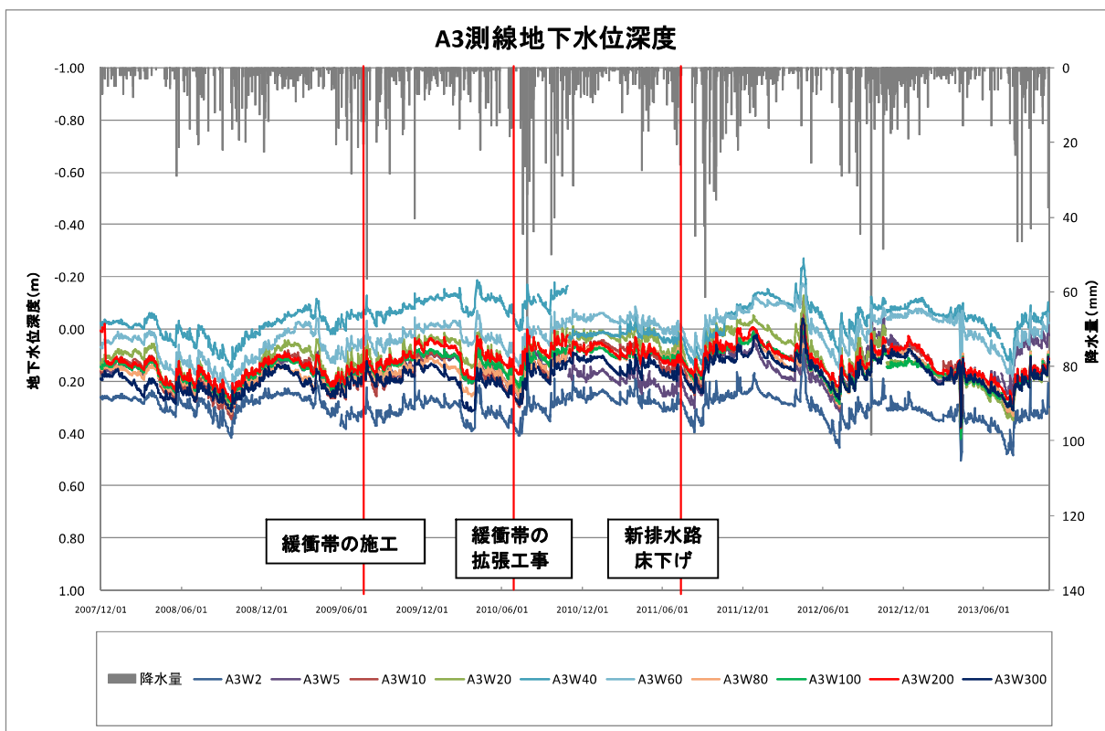
図2. 5. 24 A3 測線の地下水位深度
