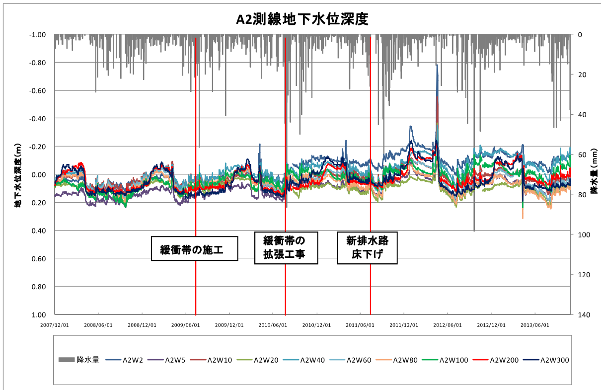
図2. 5. 22 A2 測線の地下水位深度
