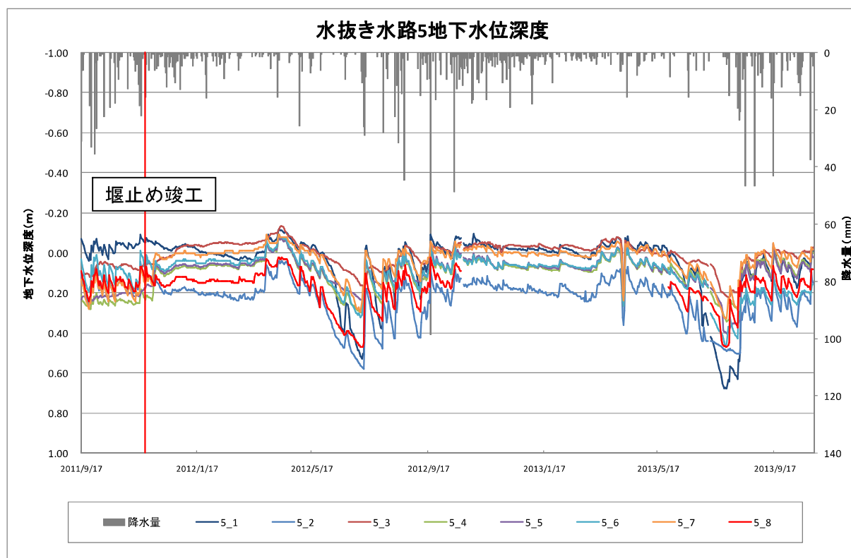
図2.5.17 水抜き水路5の地下水位深度
