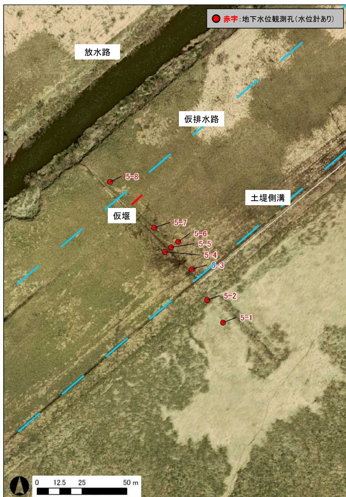
図2.5.15 水抜き水路 5 観測孔位置図
