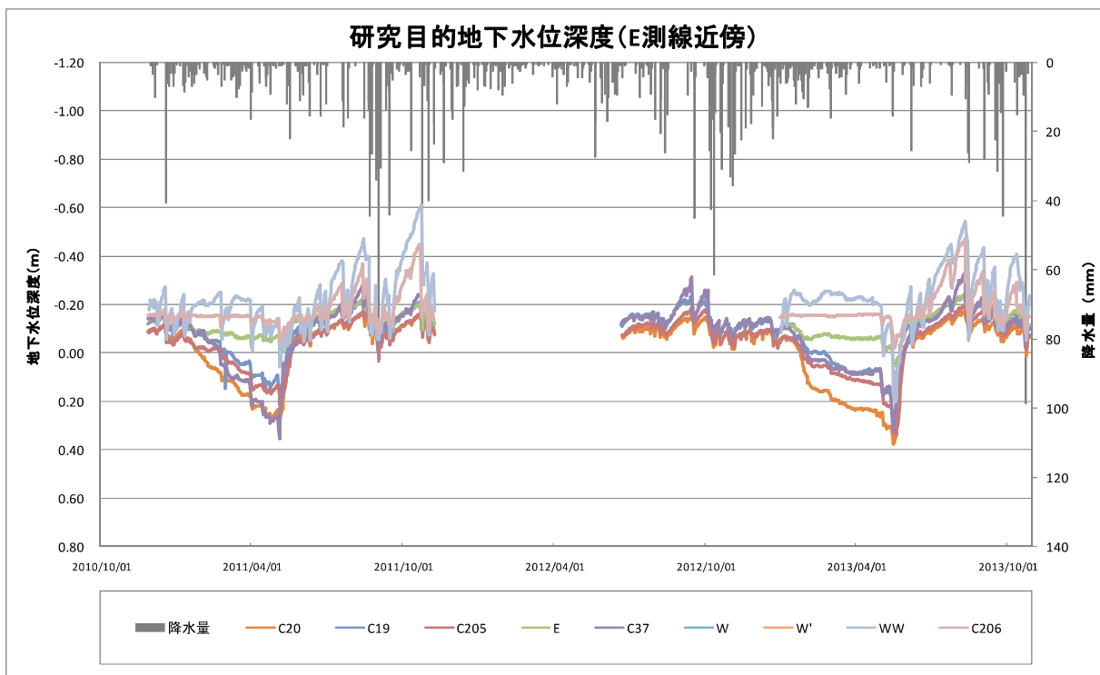
図2. 5. 45 研究目的用観測地点（E 測線近傍）の地下水位深度
