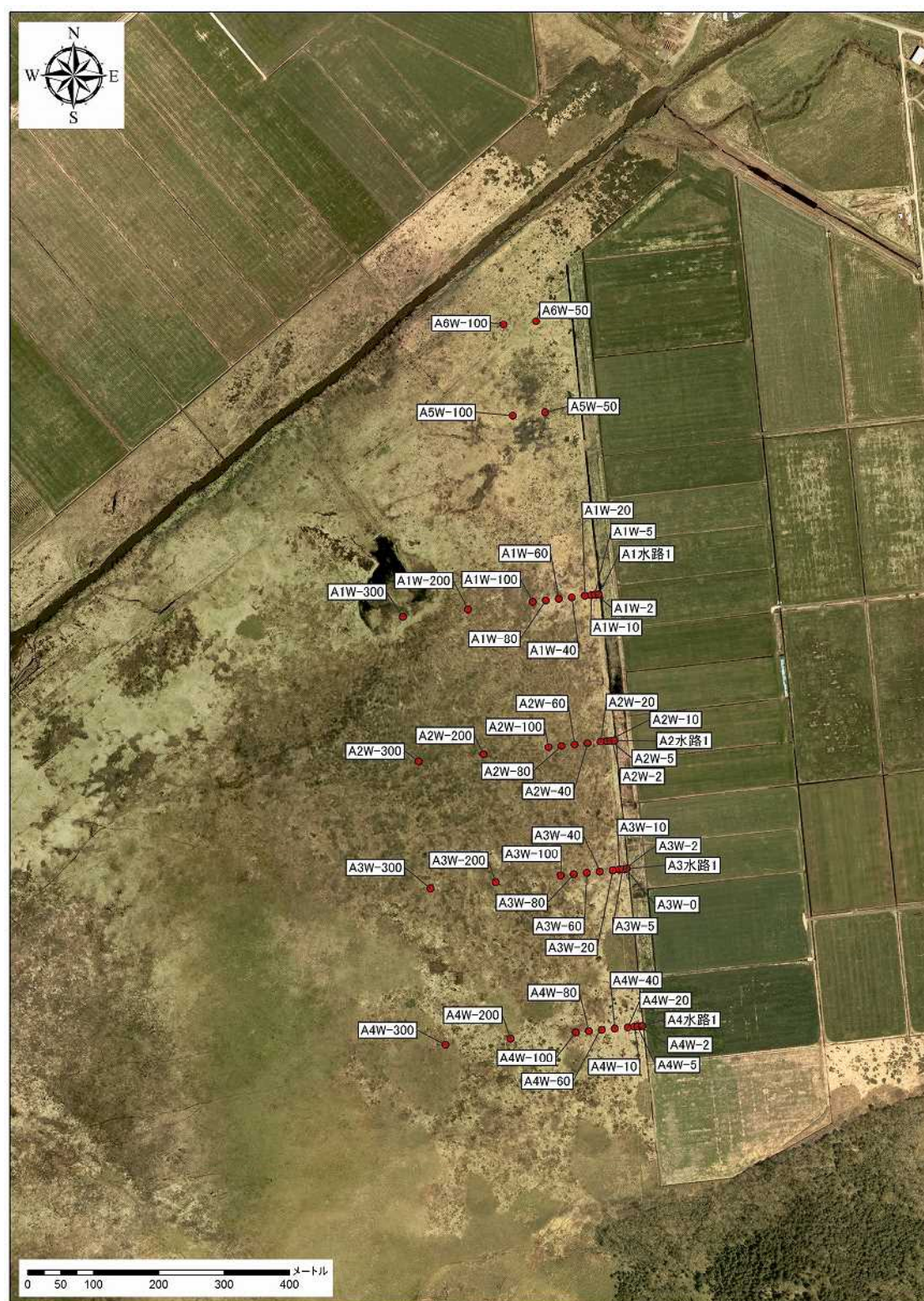
図2.5.18 A 測線観測孔位置図
