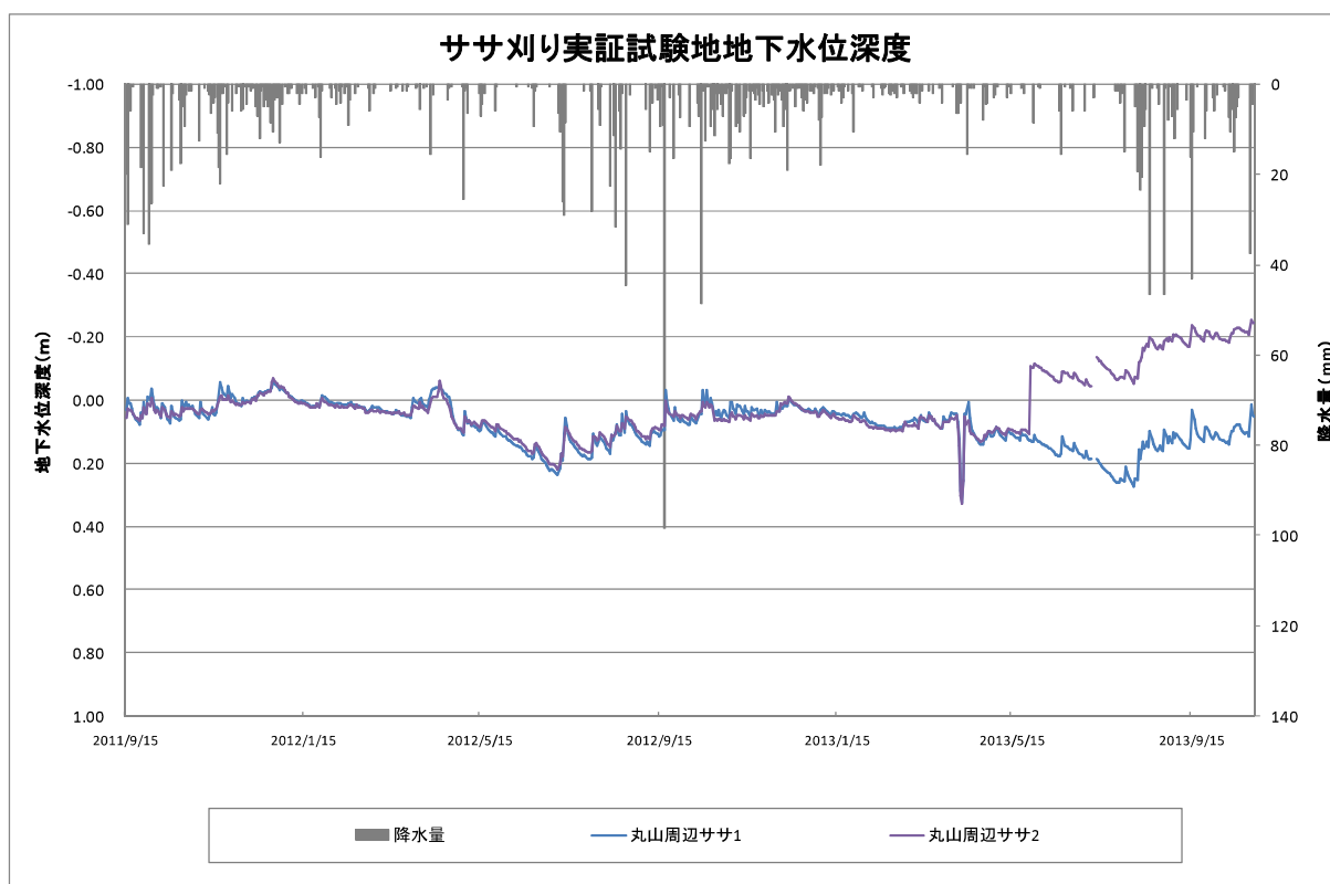
図2.5.33 ササ刈り実証試験地の地下水位深度
