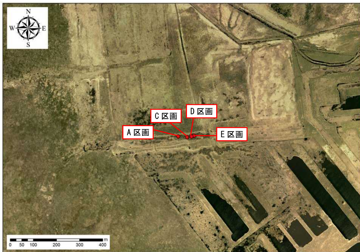
図2.5.34 泥炭採掘跡地観測孔位置図
