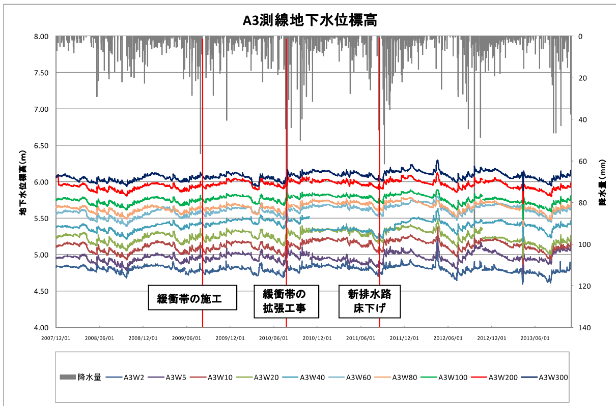
図2. 5. 23 A3 測線の地下水位標高
