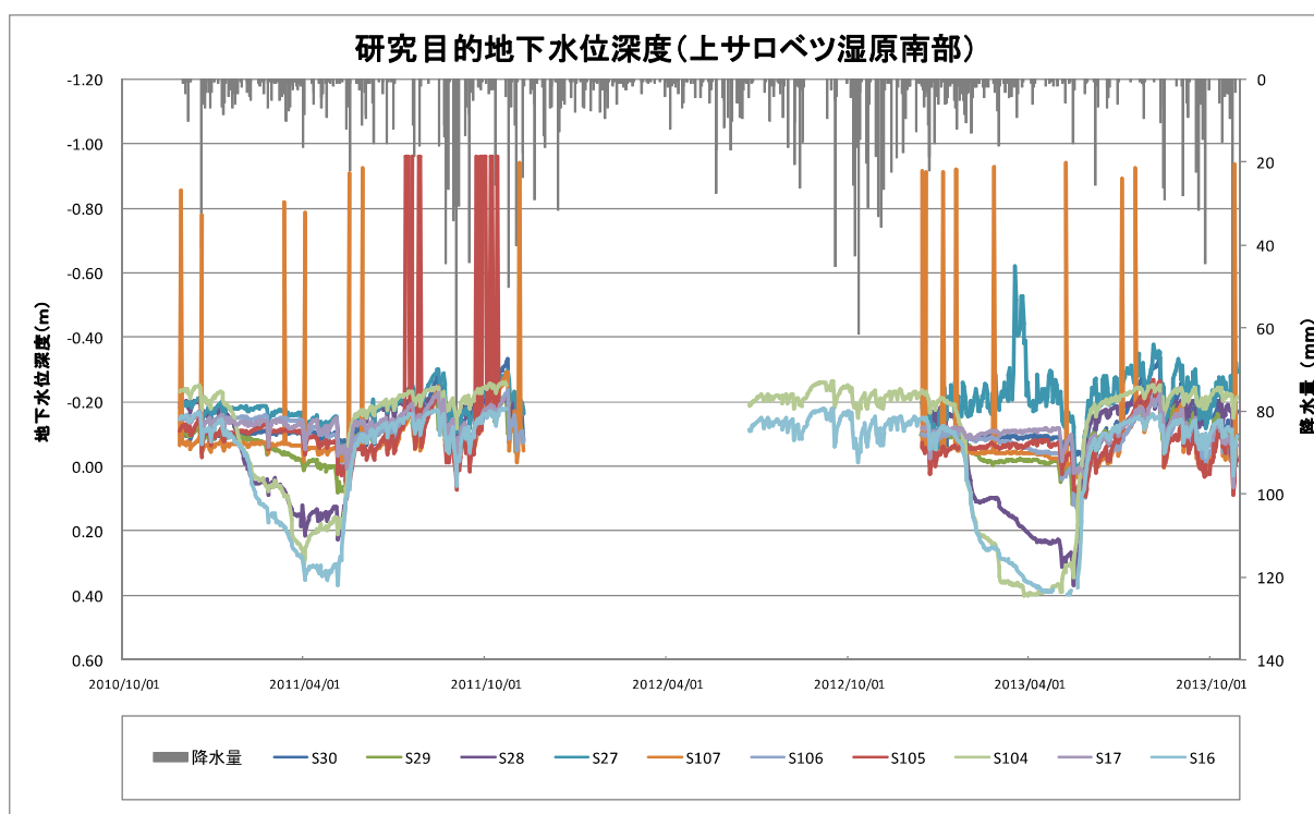
図2. 5. 46 研究目的用観測地点（上サロベツ湿原南部）の地下水位深度
