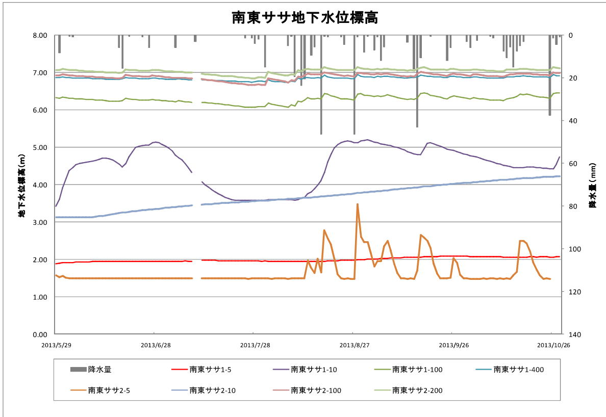
図2.5.41 南東側ササ拡大域の地下水位標高
