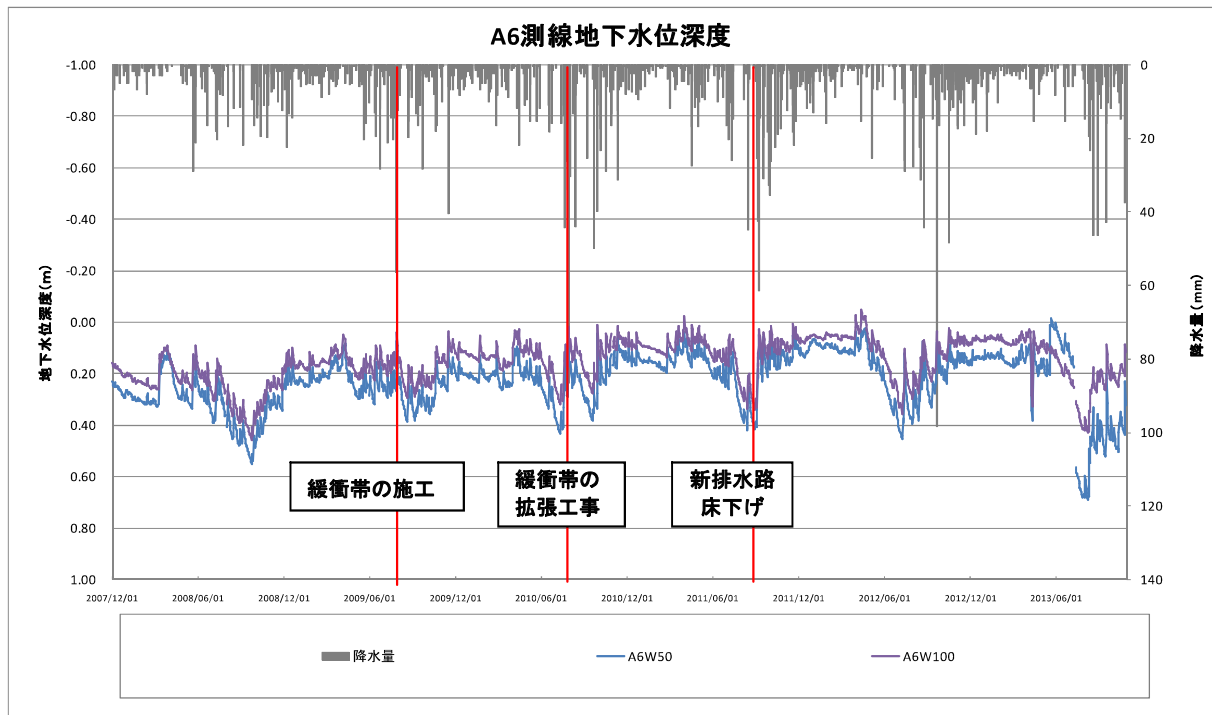
図2. 5. 30 A6 測線の地下水位深度
