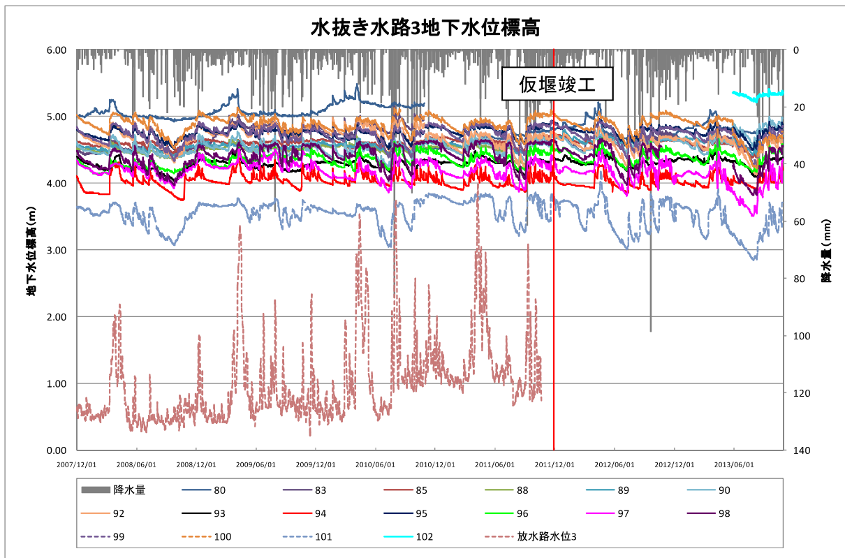
図2.5.10 水抜き水路3の地下水位標高
