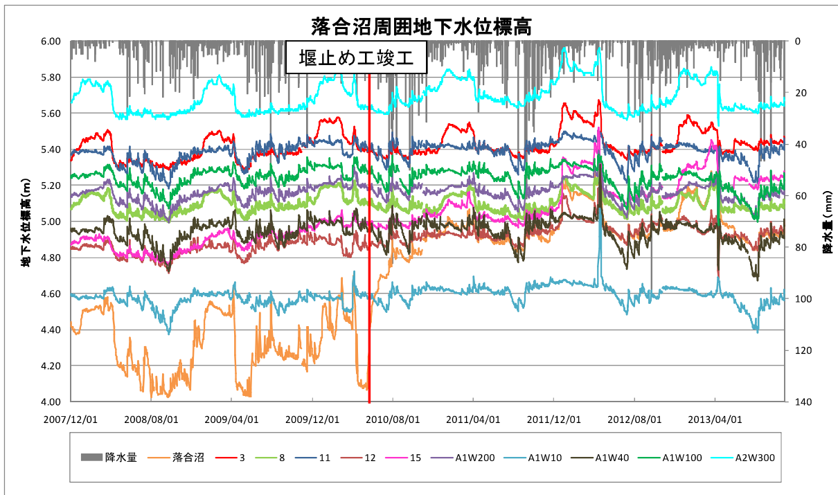
図2.5.2 落合沼周辺の地下水位標高
