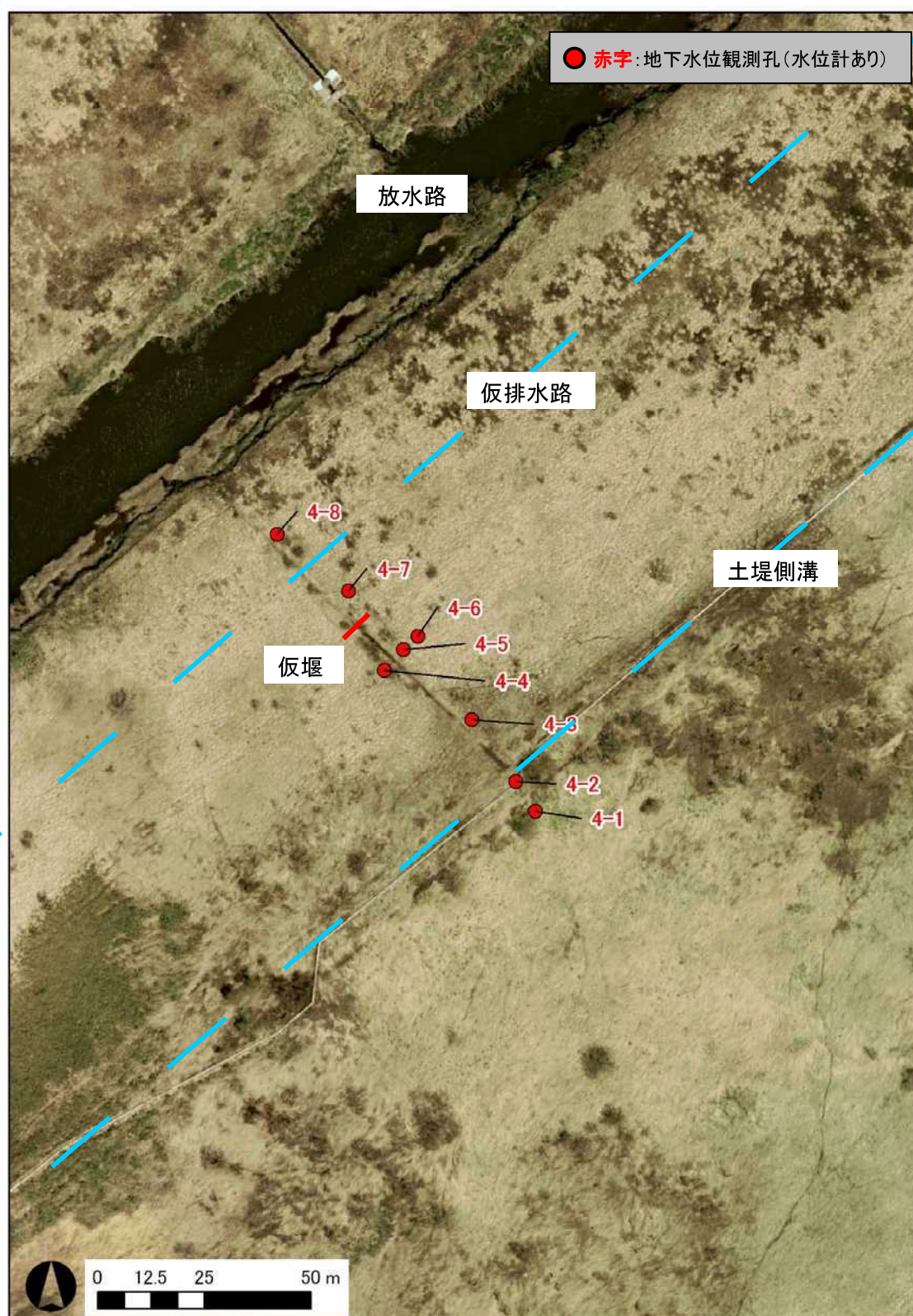
図2.5.12 水抜き水路 4 観測孔位置図
