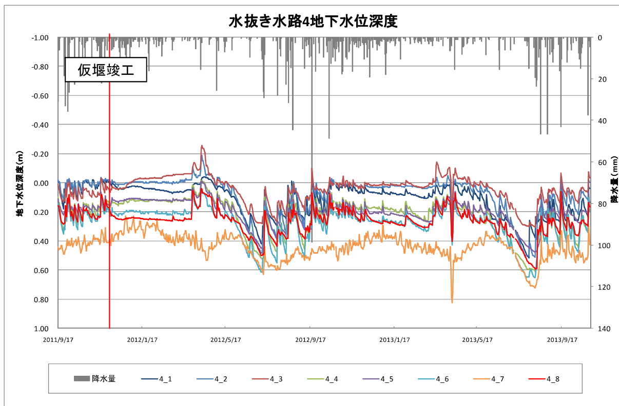
図2.5.14 水抜き水路4の地下水位深度
