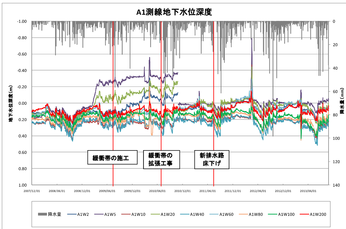
図2.5.20 A-1 測線の地下水位深度変動
