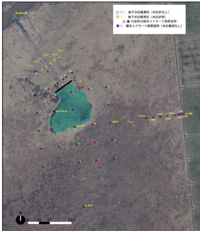
図 1.6.3 植物調査位置図（落合沼：45 地点）
