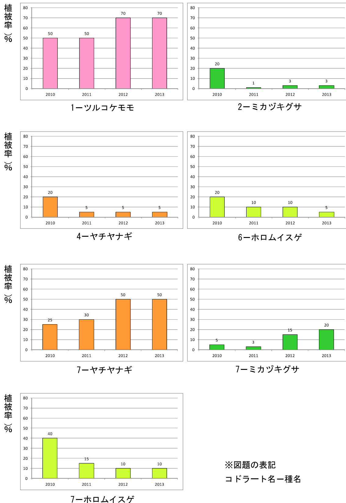
図 3.1.8 後背の高層湿原植生域における高層湿原評価指標種の植被率の変化 (15%以上の増減を確認した種を記載)
