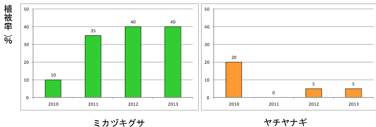
図 3.1.5 対照区における高層湿原評価指標種の植被率の変化 (15%以上の増減を確認した種を記載)
