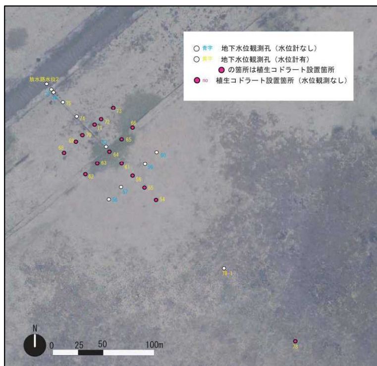
図 1.6.4 植物調査位置図（水抜き水路 2：16 地点）
