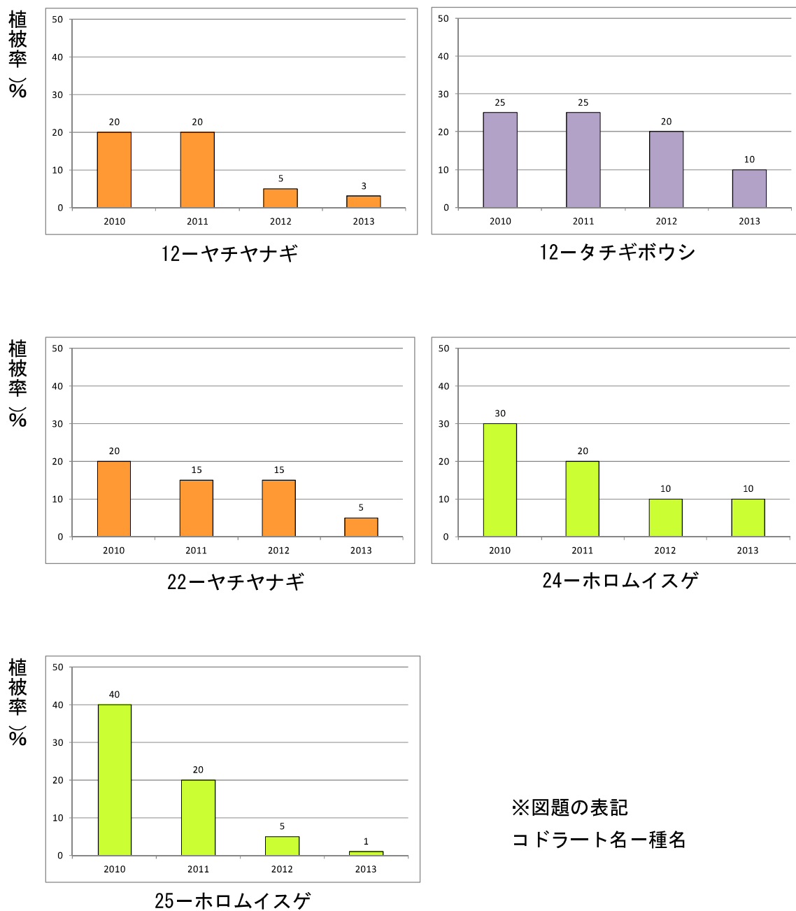
図 3.1.12 落合沼周辺における高層湿原評価指標種の植被率の変化 (15%以上の増減を確認した種を記載)
