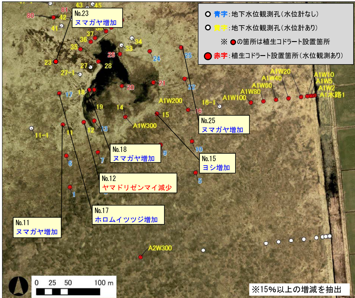
図 3.1.13 落合沼周辺におけるその他の種の主な変化 (2010 年と 2013 年を比較)
