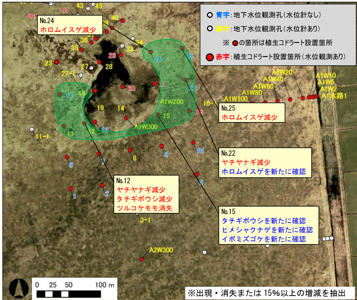
図 3.1.11 落合沼周辺における高層湿原評価指標種の主な変化 (2010 年と 2013 年を比較)
