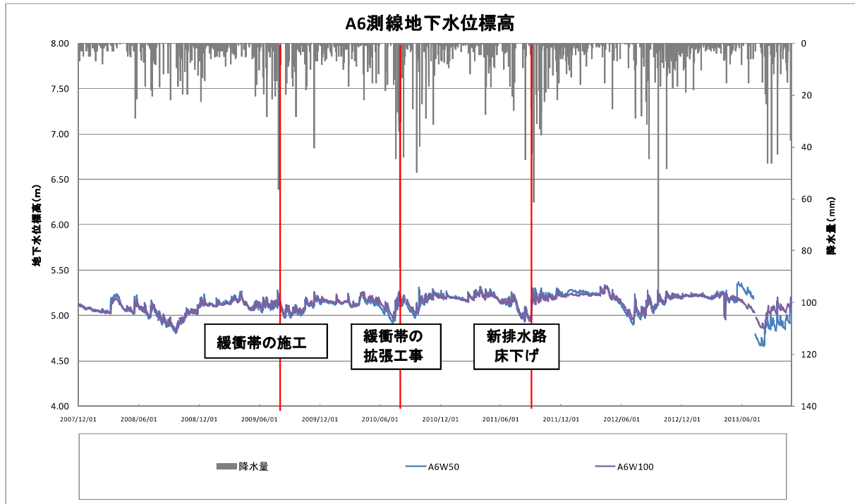
図2. 5. 29 A6 測線の地下水位標高
