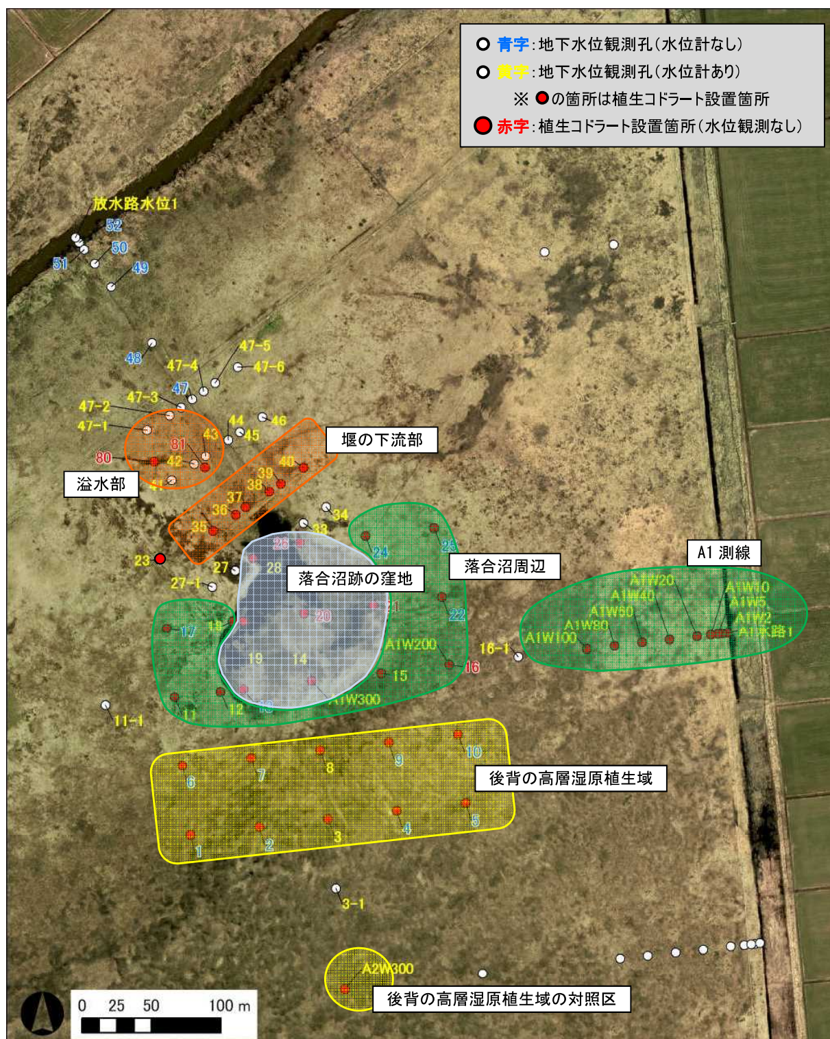
図 3.1.3 水抜き水路1（落合沼）の調査地点
