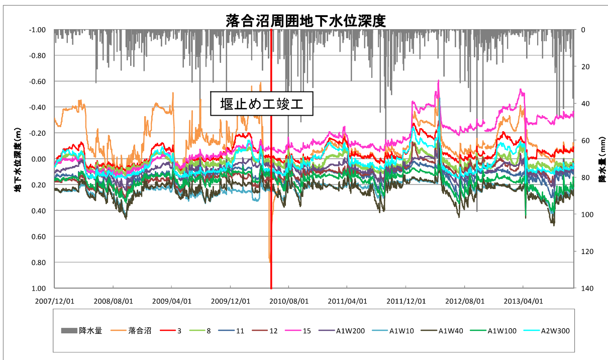
図2.5.3 落合沼周辺の地下水位深度
