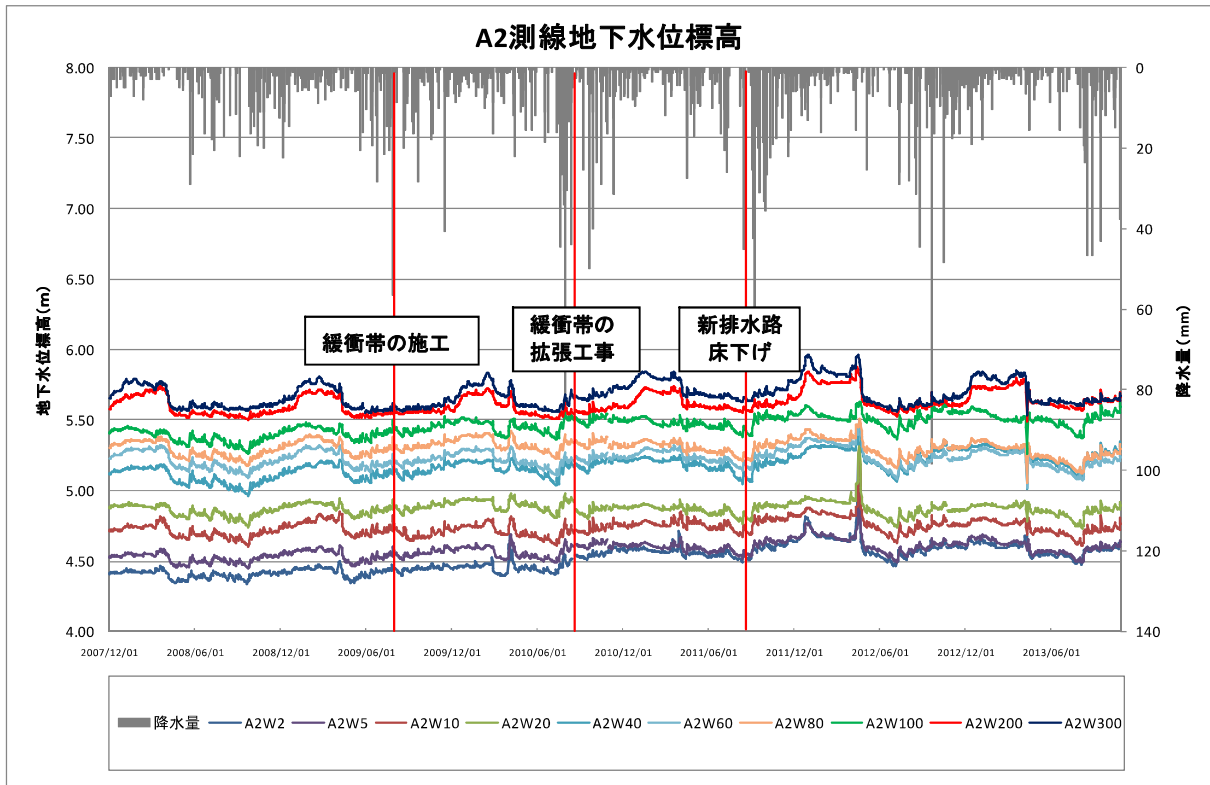
図2. 5. 21 A2 測線の地下水位標高
