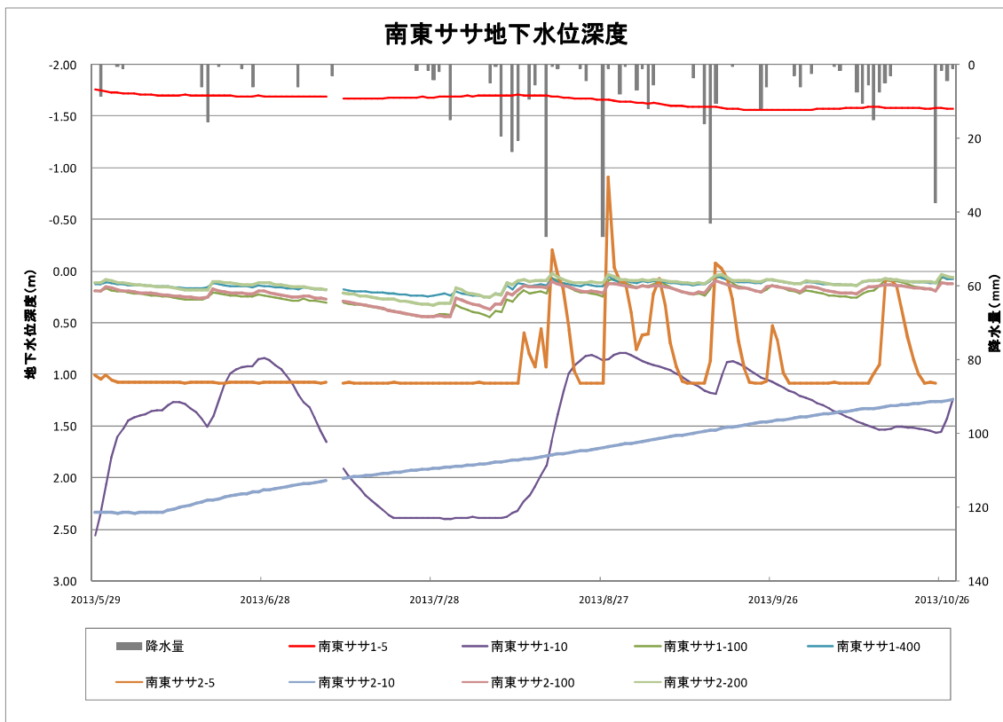
図2.5.42 南東側ササ拡大域の地下水位深度
