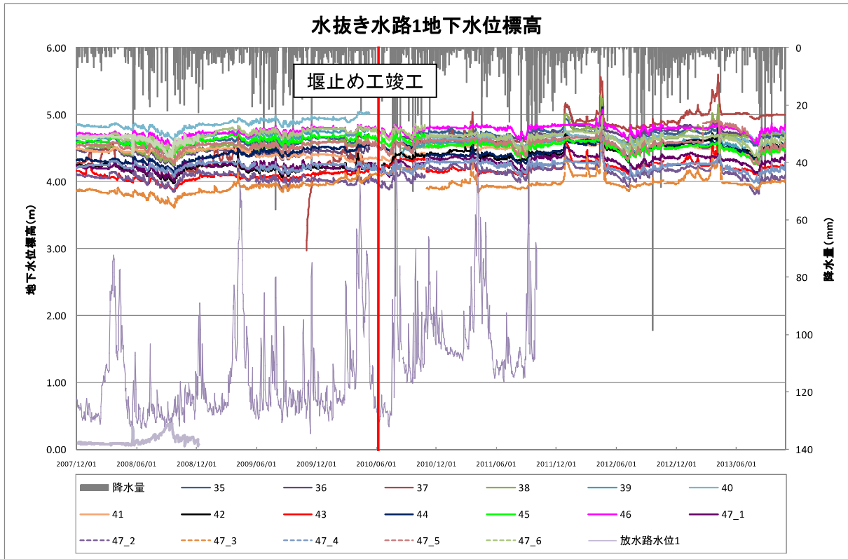
図2.5.4 水抜き水路1の地下水位標高
