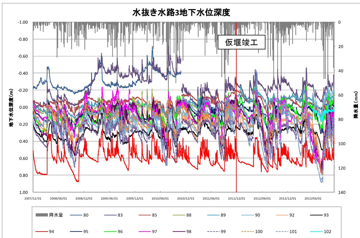
図2.5.11 水抜き水路3の地下水位深度
