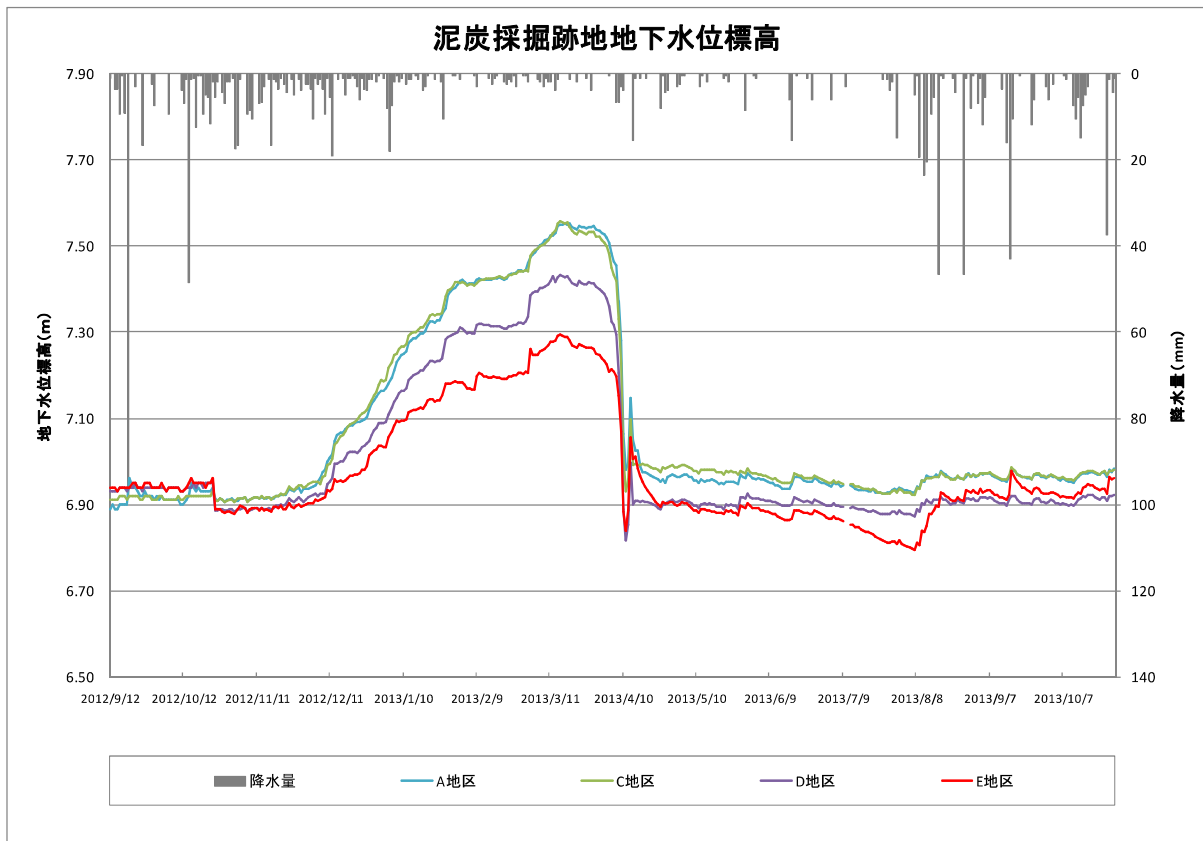
図2.5.35 泥炭採掘跡地の地下水位標高
