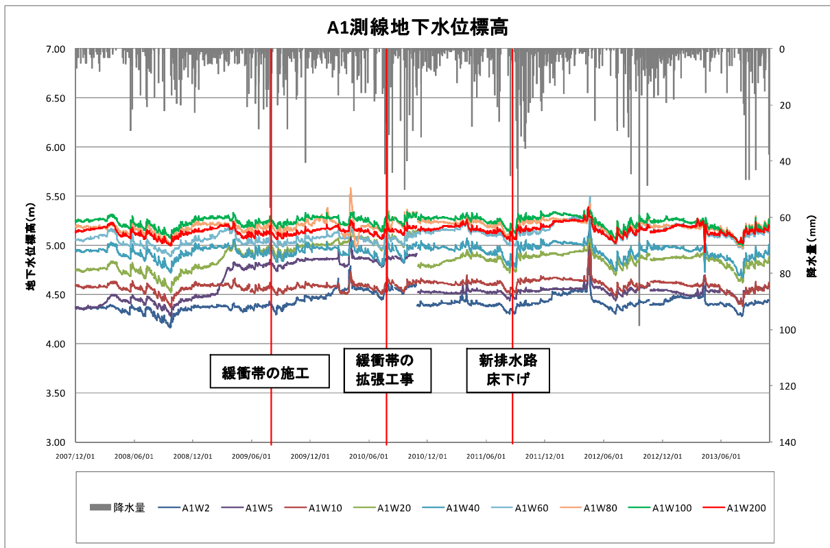
図2.5.19 A-1 測線の地下水位標高変動
