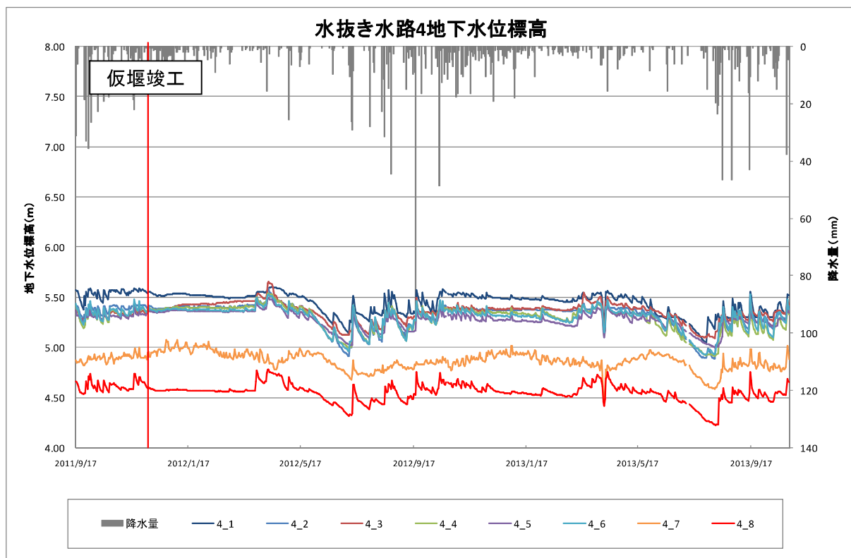
図2.5.13 水抜き水路4の地下水位標高
