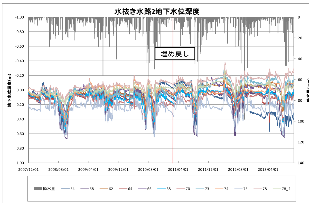
図2.5.8 水抜き水路 2 の地下水位深度
