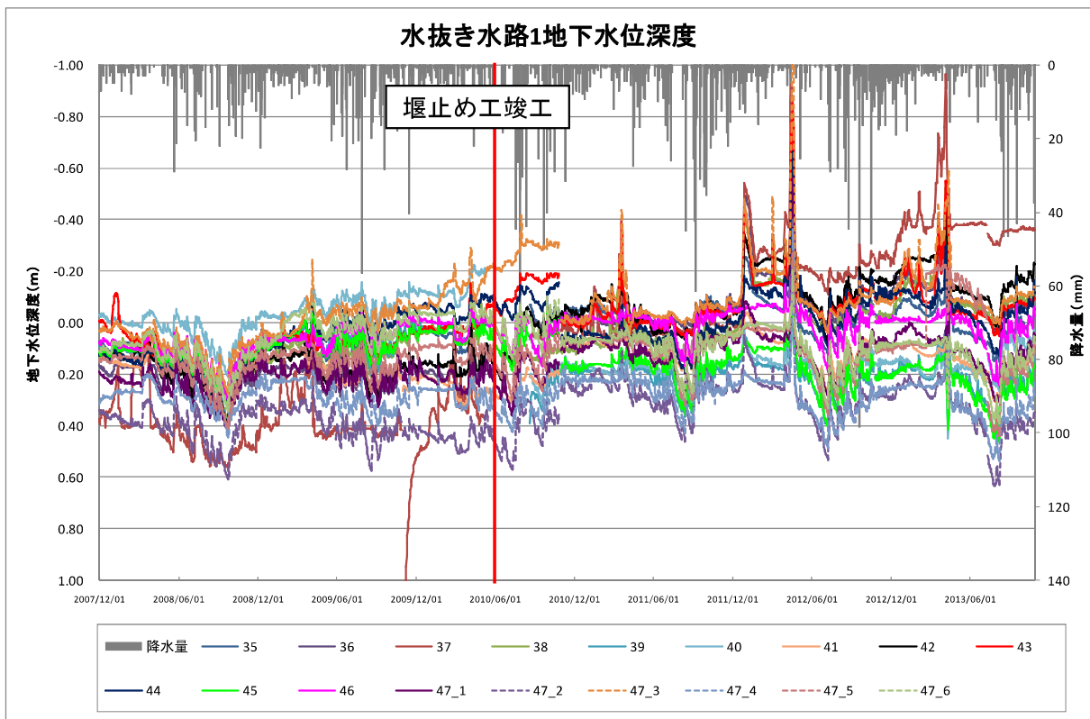
図2.5.5 水抜き水路1の地下水位深度
