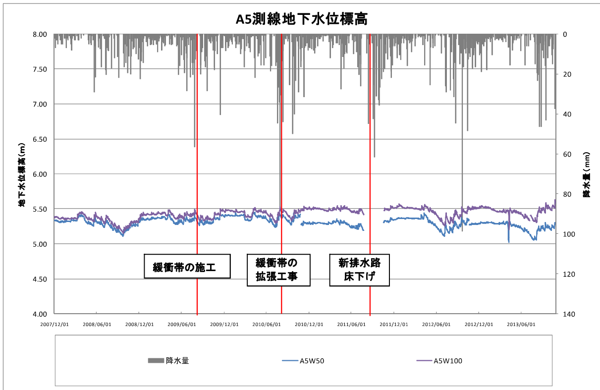
図2. 5. 27 A5 測線の地下水位標高
