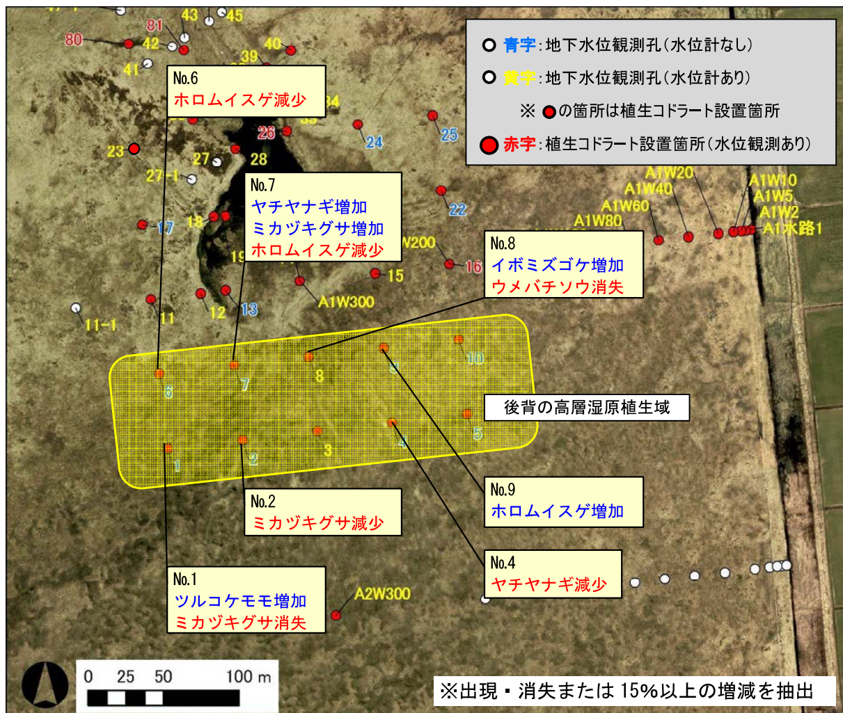
図 3.1.7 後背の高層湿原植生域における高層湿原評価指標種の主な変化 (2010 年と 2013 年を比較)
