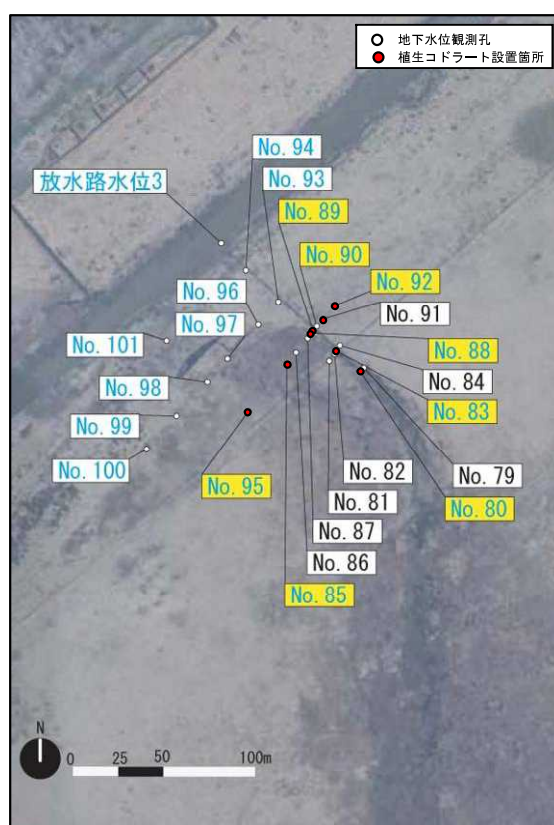
図 1.6.5 植物調査位置図（水抜き水路 3：8 地点）
