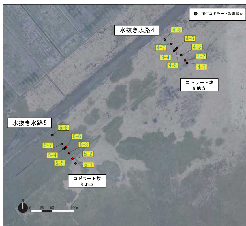
図 1.6.6 植物調査位置図（水抜き水路 4 および 5：16 地点）
