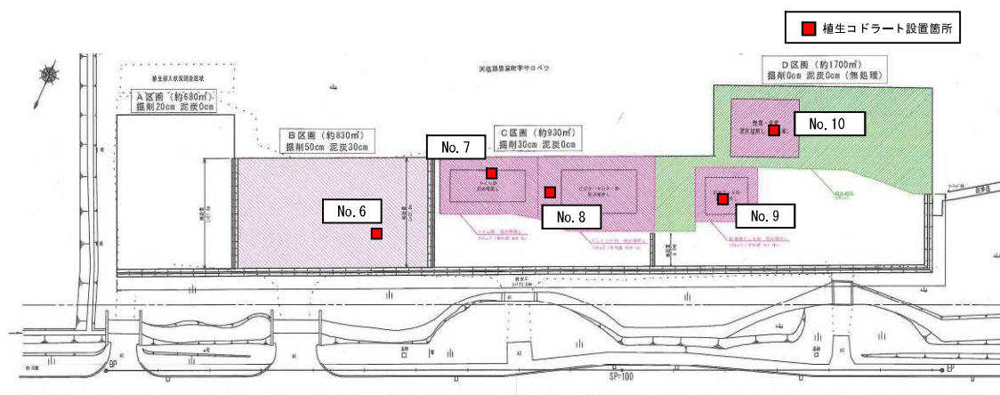
図 1.6.8 植物調査位置図（原生花園園地跡地（A～D 区画：5 地点）
