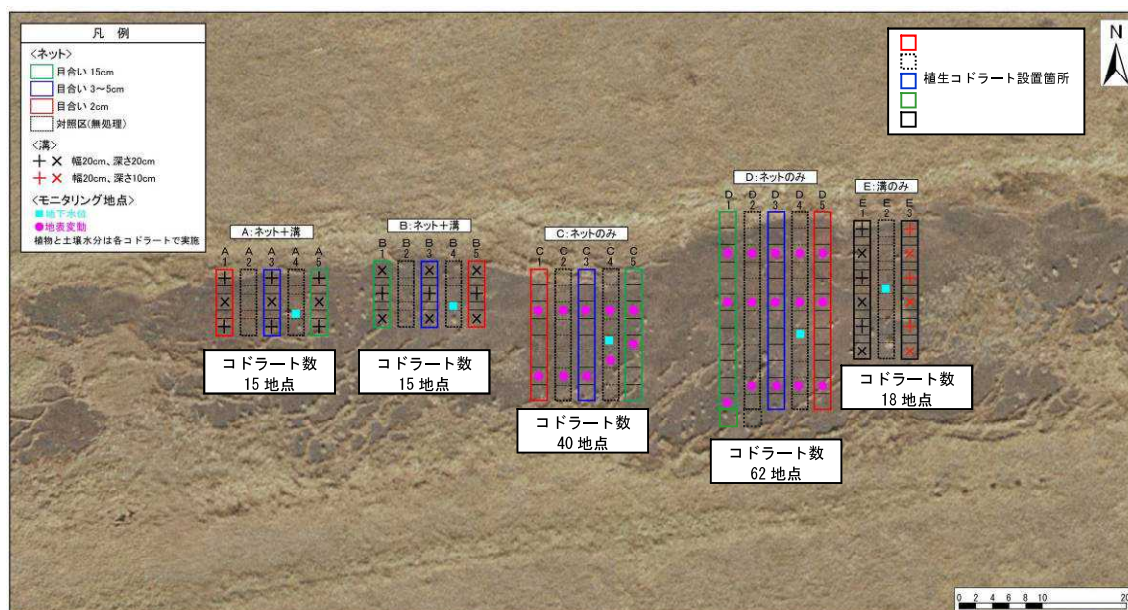
図 1.6.9 植物調査位置図（泥炭採掘跡地：150 地点）
