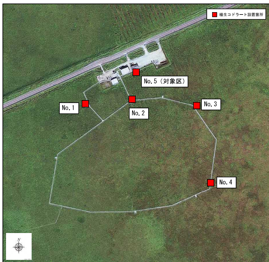
図 1.6.7 植物調査位置図（原生花園園地跡地（歩道設置跡：5 地点）
