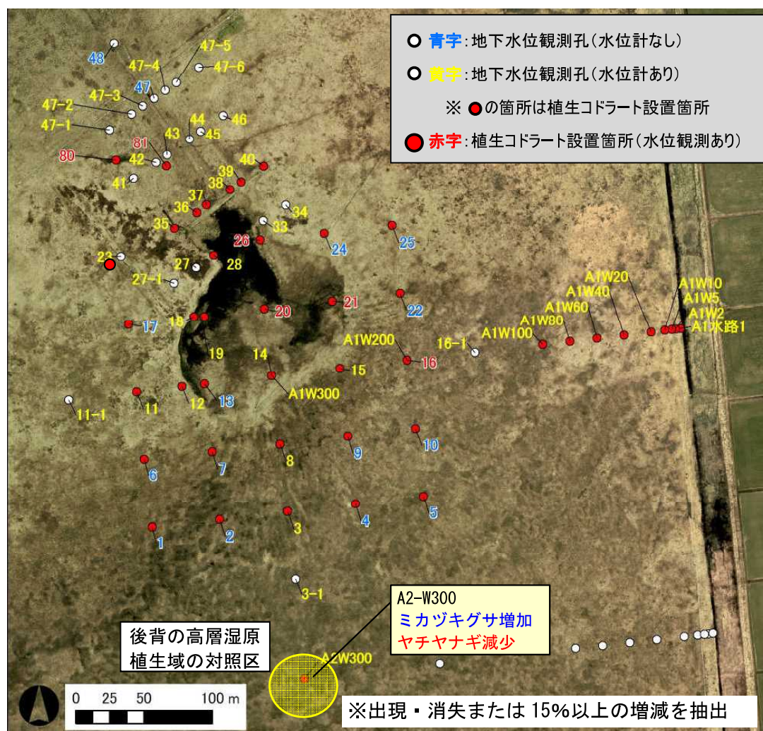
図 3.1.4 対照区における高層湿原評価指標種の主な変化 (2010 年と 2013 年を比較)
