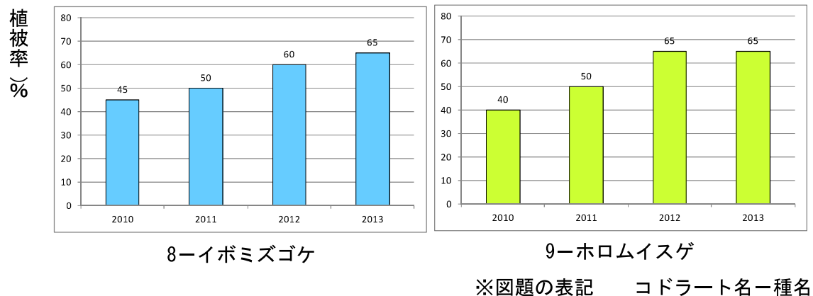
図 3.1.9 後背の高層湿原植生域における高層湿原評価指標種の植被率の変化 (15%以上の増減を確認した種を記載)
