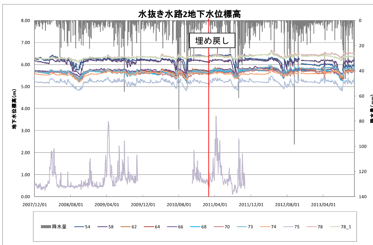
図2.5.7 水抜き水路 2 の地下水位標高
