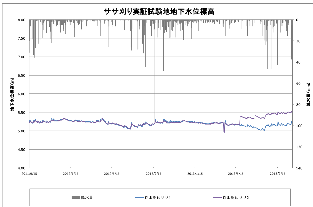
図2.5.32 ササ刈り実証試験地の地下水位標高
