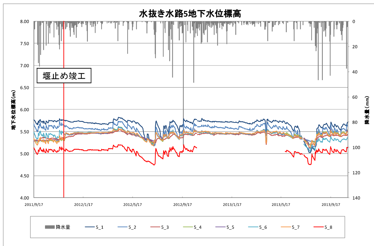
図2.5.16 水抜き水路5の地下水位標高
