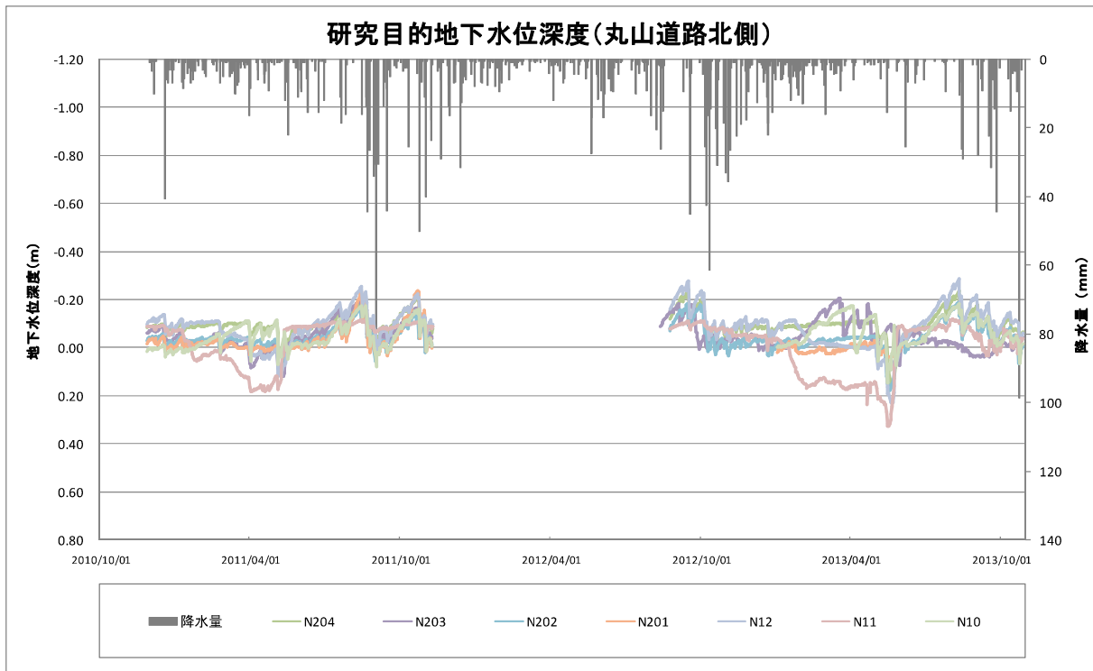
図2. 5. 44 研究目的用観測地点（丸山道路北側）の地下水位深度
