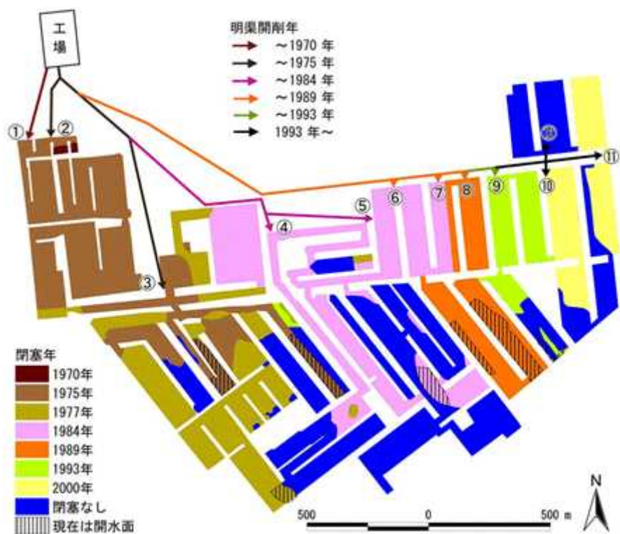
図 5-5 排水明渠の軌跡と水面閉塞年代
