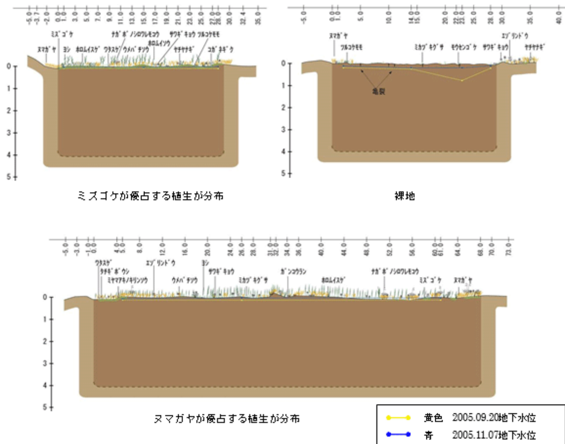
図 5-11 基盤構造と植生断面模式(ペースト状泥炭が厚く堆積した採掘跡地)
