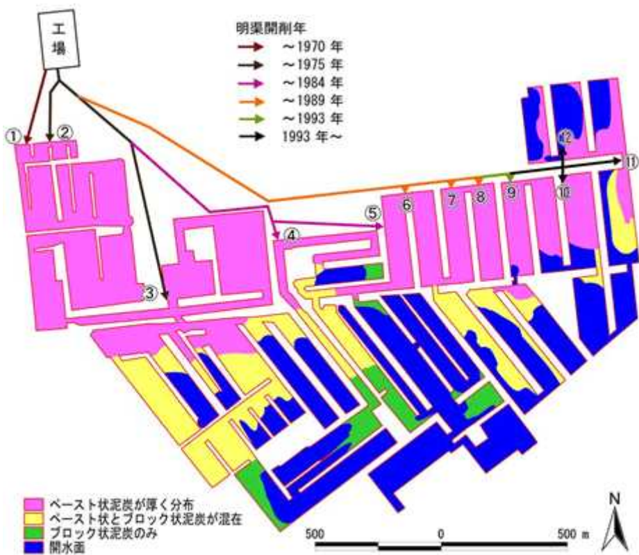
図 5-6 泥炭の性状分布
