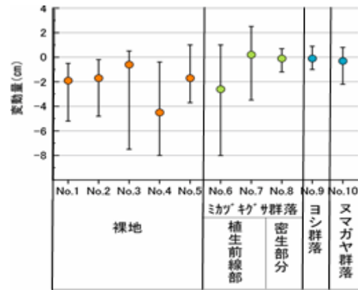
図 5-17 表層変動量計測結果
