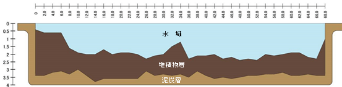
図 5-24 基盤構造の断面模式(開水面)
