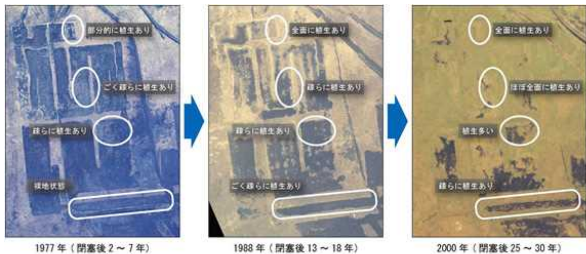
図5-10 泥炭採掘跡地における植生の遷移
