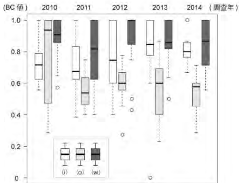
図Ⅱ 1－3. 長尾峠における BC 値の箱ひげ図
