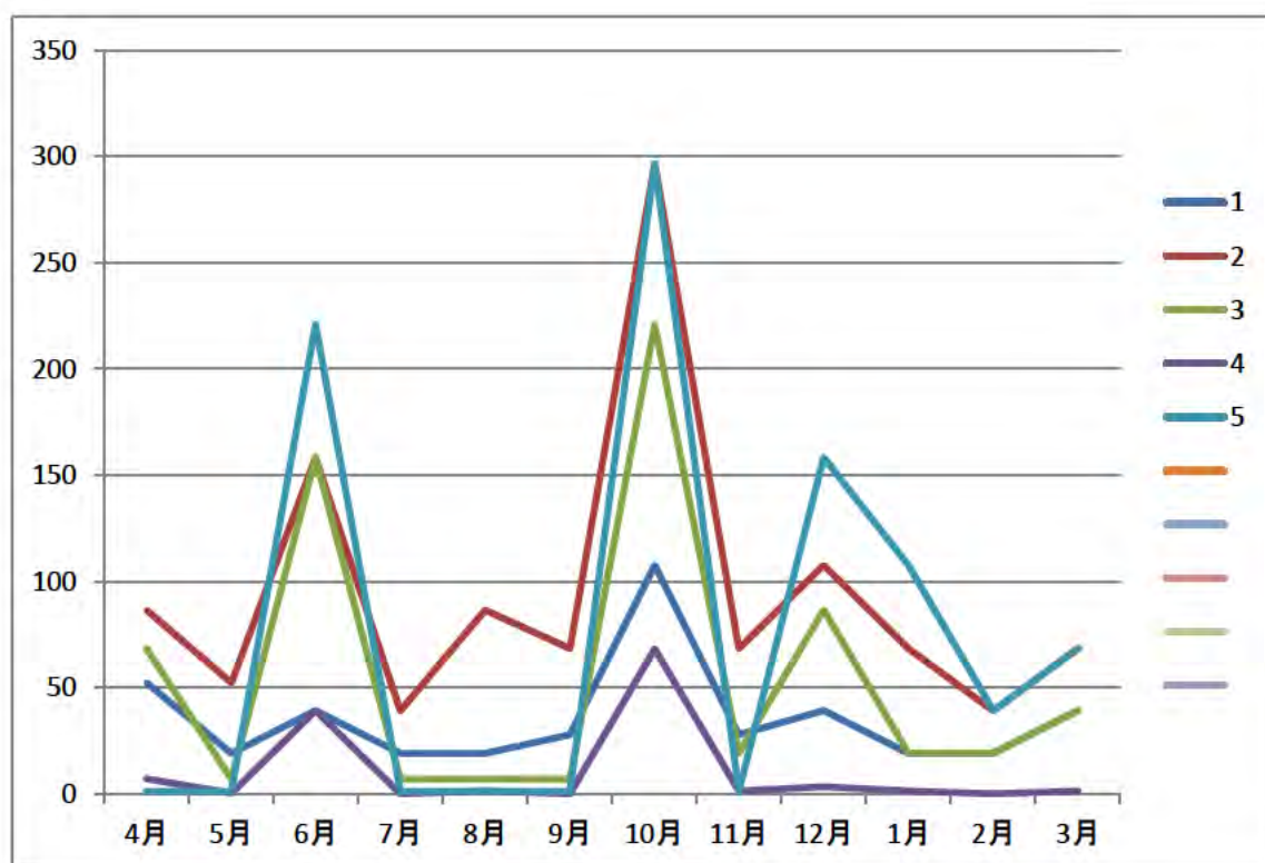
図IV 2－2 平成26年度の湧水量の月別変化
