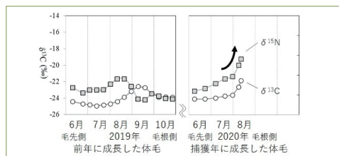
図. 2020年8月に上高地で捕獲されたツキノワグマ体毛の炭素・窒素安定同位体比（中下ほか2021より引用）
