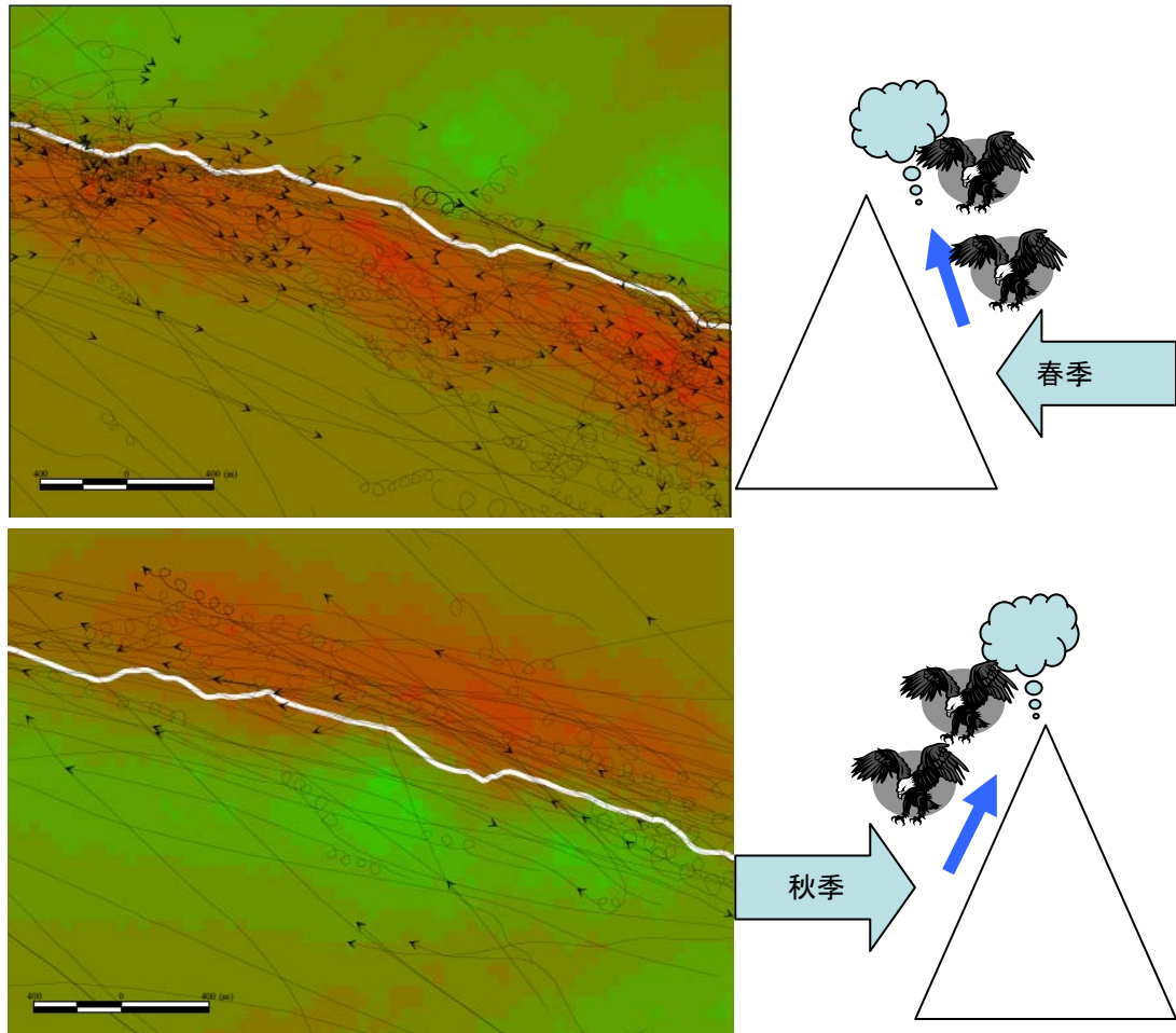
図 3-26 山陵線における猛禽類の渡りと気流シミュレーション結果
