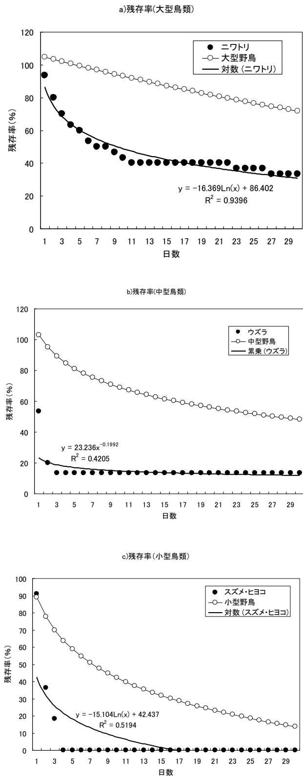
図 3-57 鳥類死骸を用いた残存率曲線
