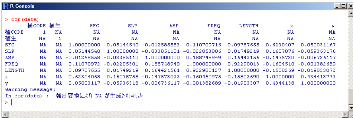
図 3-37 相関行列の例
