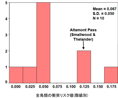
図 3- 19 Smallwood et al (2004)による飛翔頻度と衝突リスク
