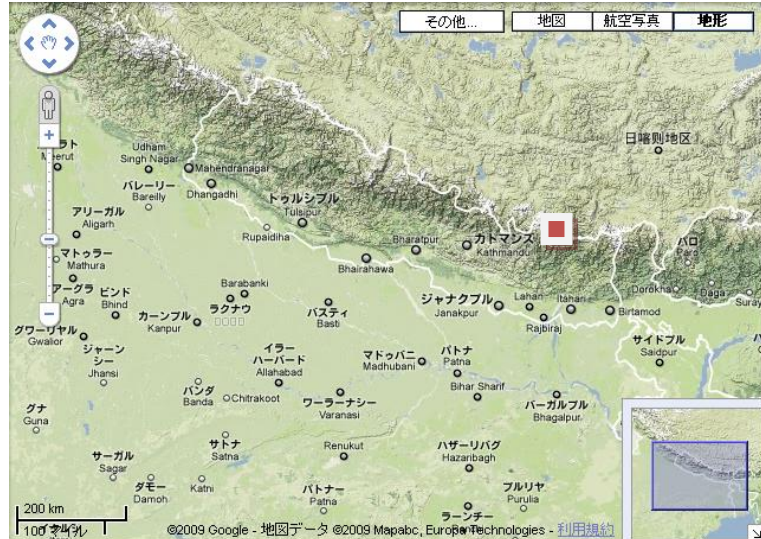
図 ネパール東北部ソル・クンブ郡 出所: Google マップ. http://maps.google.co.jp/maps?hl=ja&tab=w1
