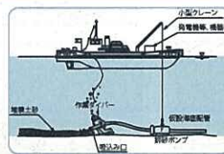
作業船の仕組み
