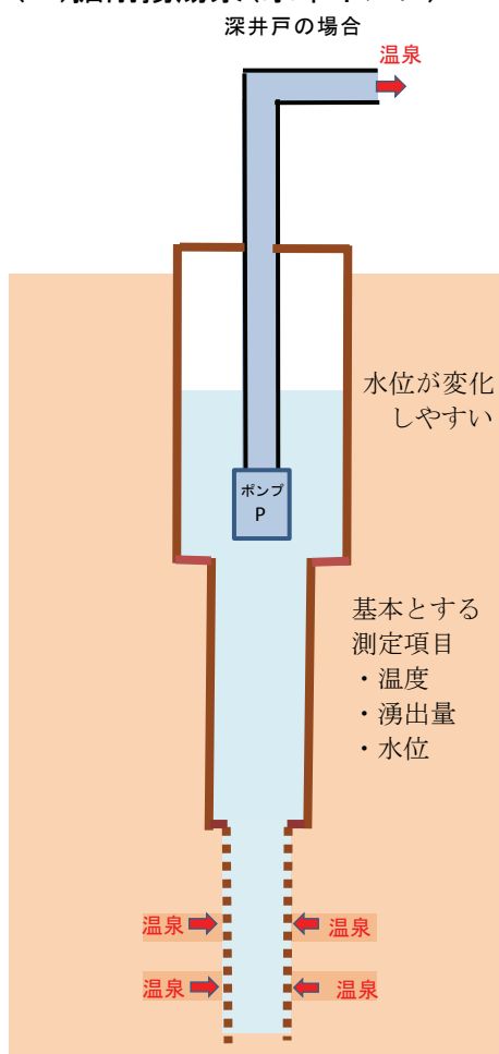
(c2)掘削揚湯泉(水中ポンプ)
