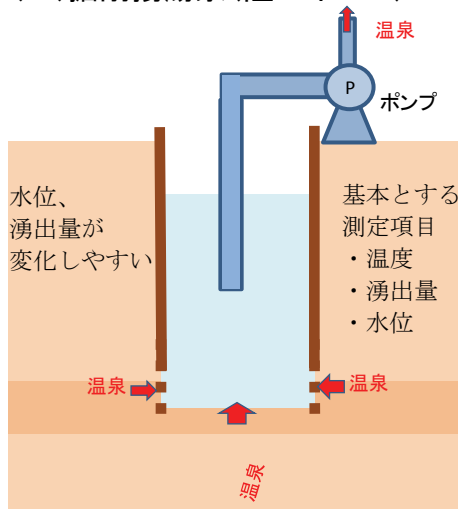
(c1)掘削揚湯泉(陸上ポンプ)
