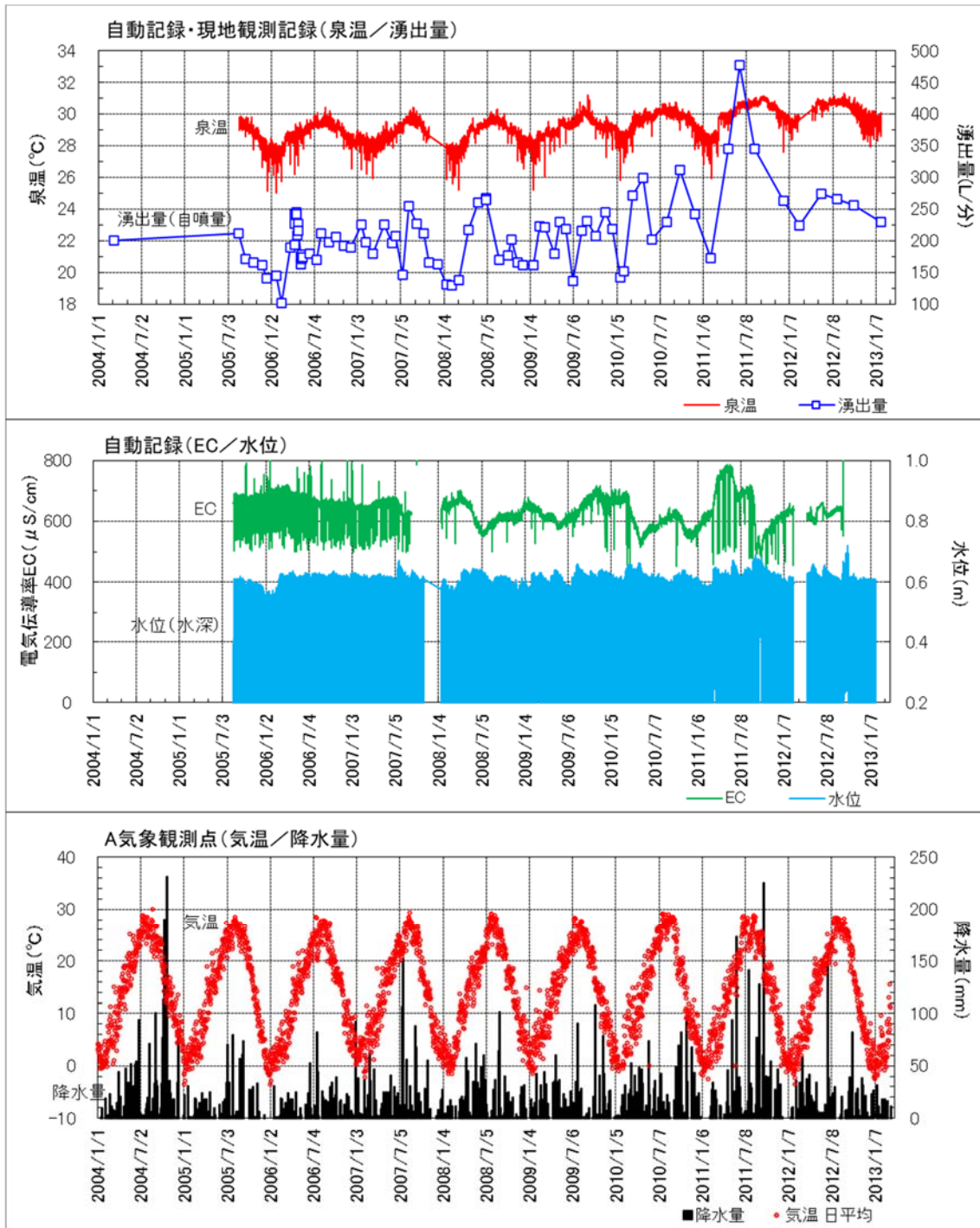
図4 深度の浅い源泉の長期モニタリング結果（自然湧出泉）
