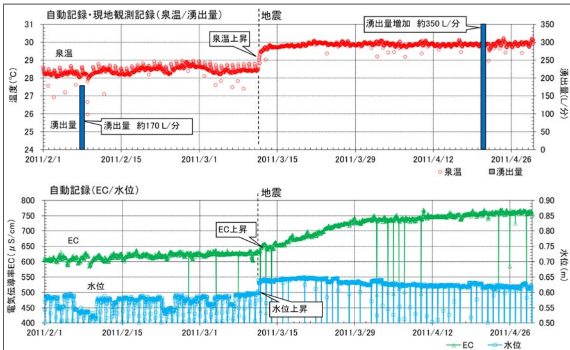
図5 深度の浅い源泉の地震発生前後の湧出状況変化
