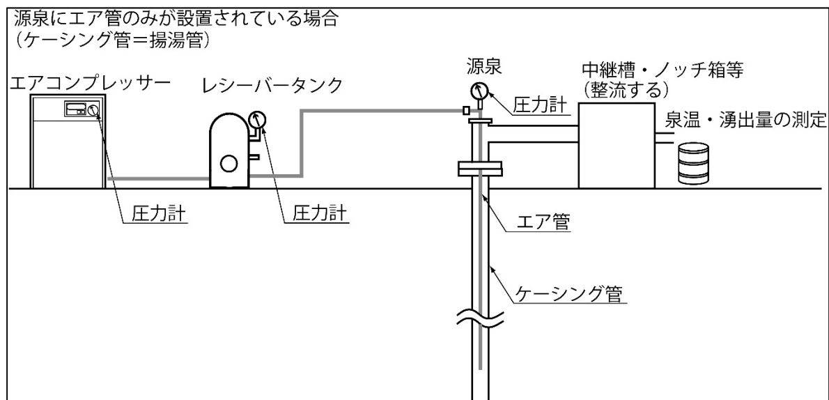
図9 エアリフト揚湯源泉の概略図（揚湯管設置なし）
