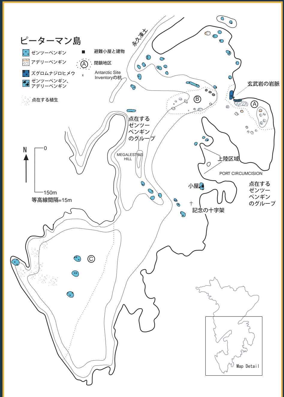
玄武岩岩脈付近のズグロムナジロヒメウ (ピーターマン島北東)
