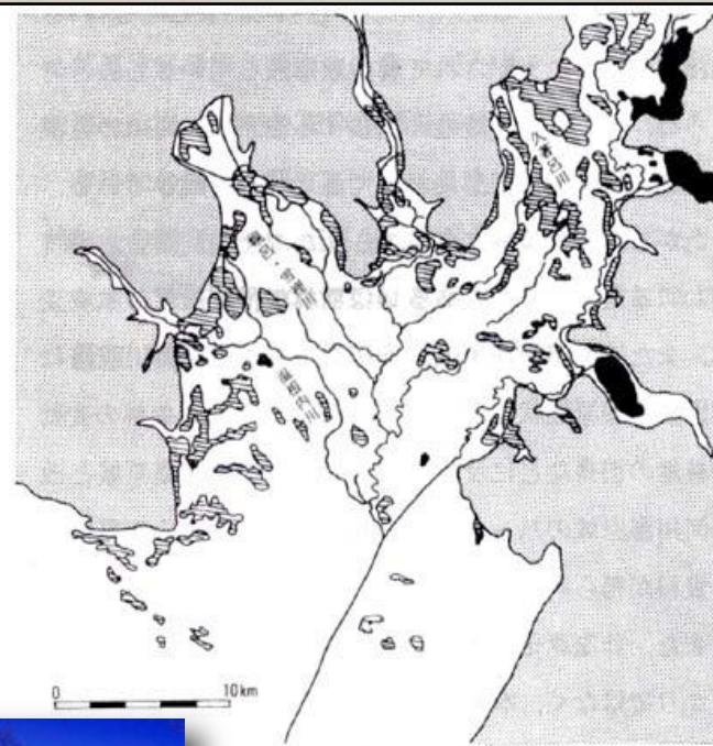
図5. ハンノキ林 (1977年)
