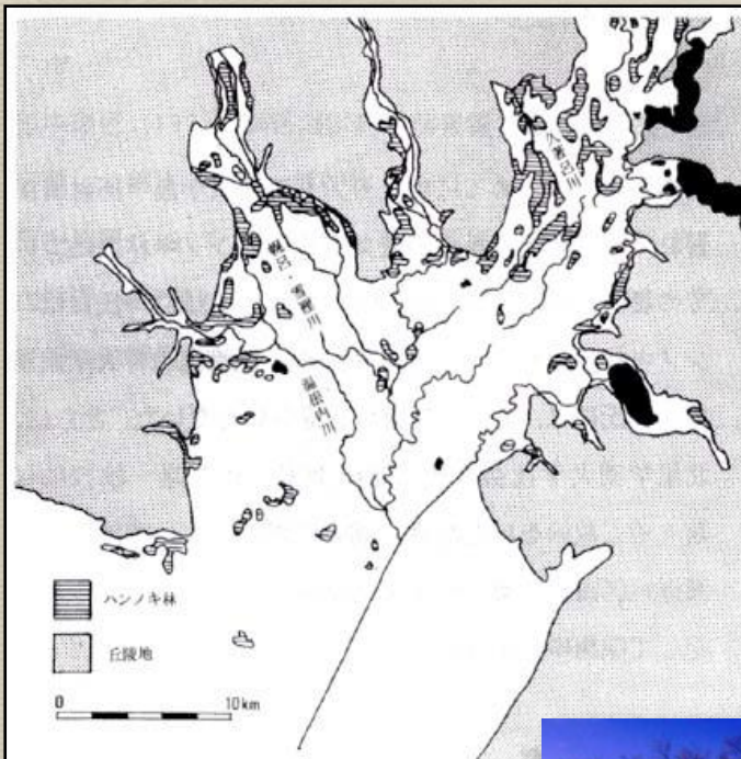
図4. ハンノキ林 (1947年)
