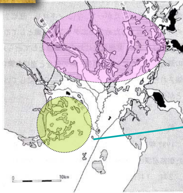
図7. ハンノキ林 (1992年)
