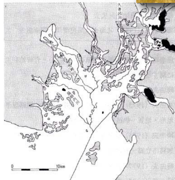
図6. ハンノキ林 (1984年)
