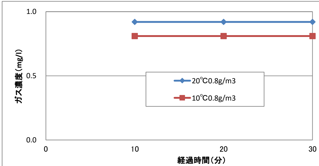
図3 アルゼンチンアリ(働きアリ成虫)を青酸ガスくん蒸したときの 温度・薬量別ガス濃度の経時変化
