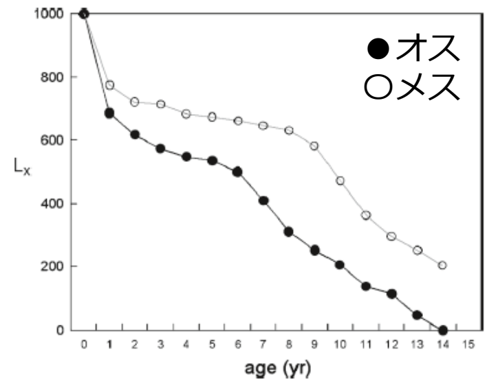
金華山における生存曲線
