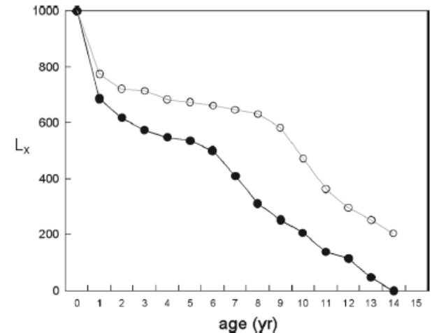
金華山におけるシカの年齢ごとの生存率 (●オス、○メス) Minami et al 2009
