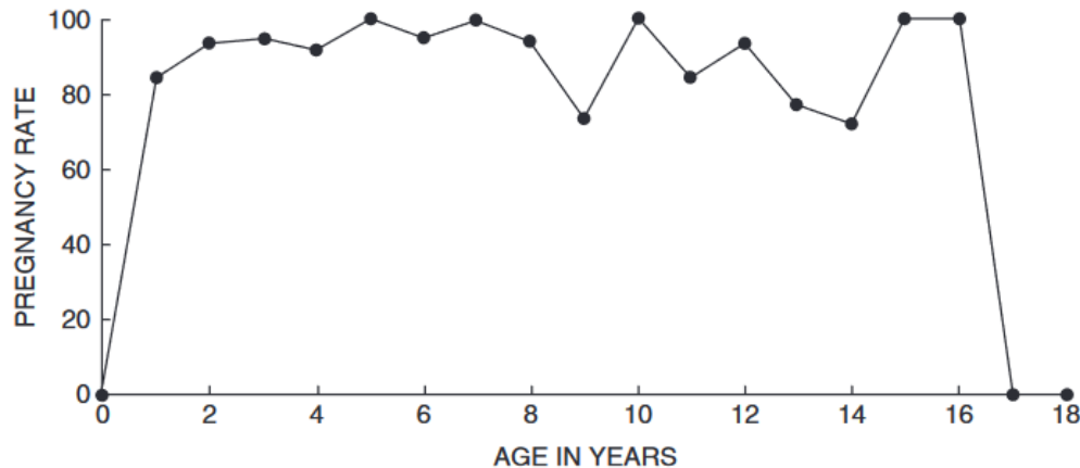
二ホンジカの年齢ごとの妊娠率 (Koizumi et al 2009)
