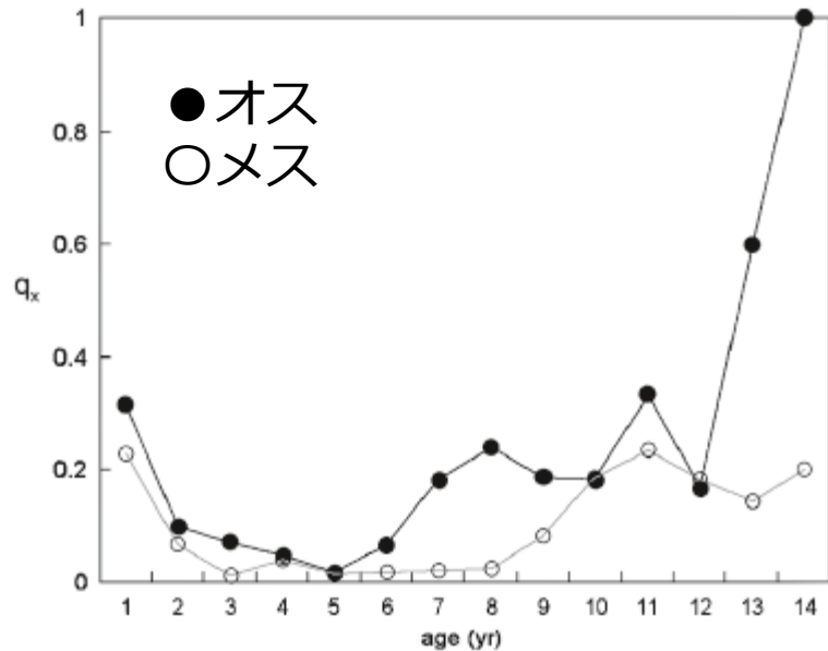
金華山における年齢ごとの死亡率
