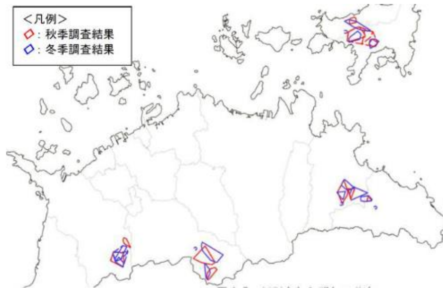
図Ⅲ-1-3 出没カレンダー調査により推定された群れの分布 (野生動物保護管理事務所, 2013)
