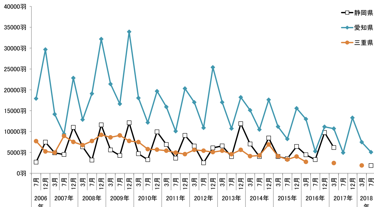
図7. 静岡県、愛知県、三重県のカワウ個体数の推移
