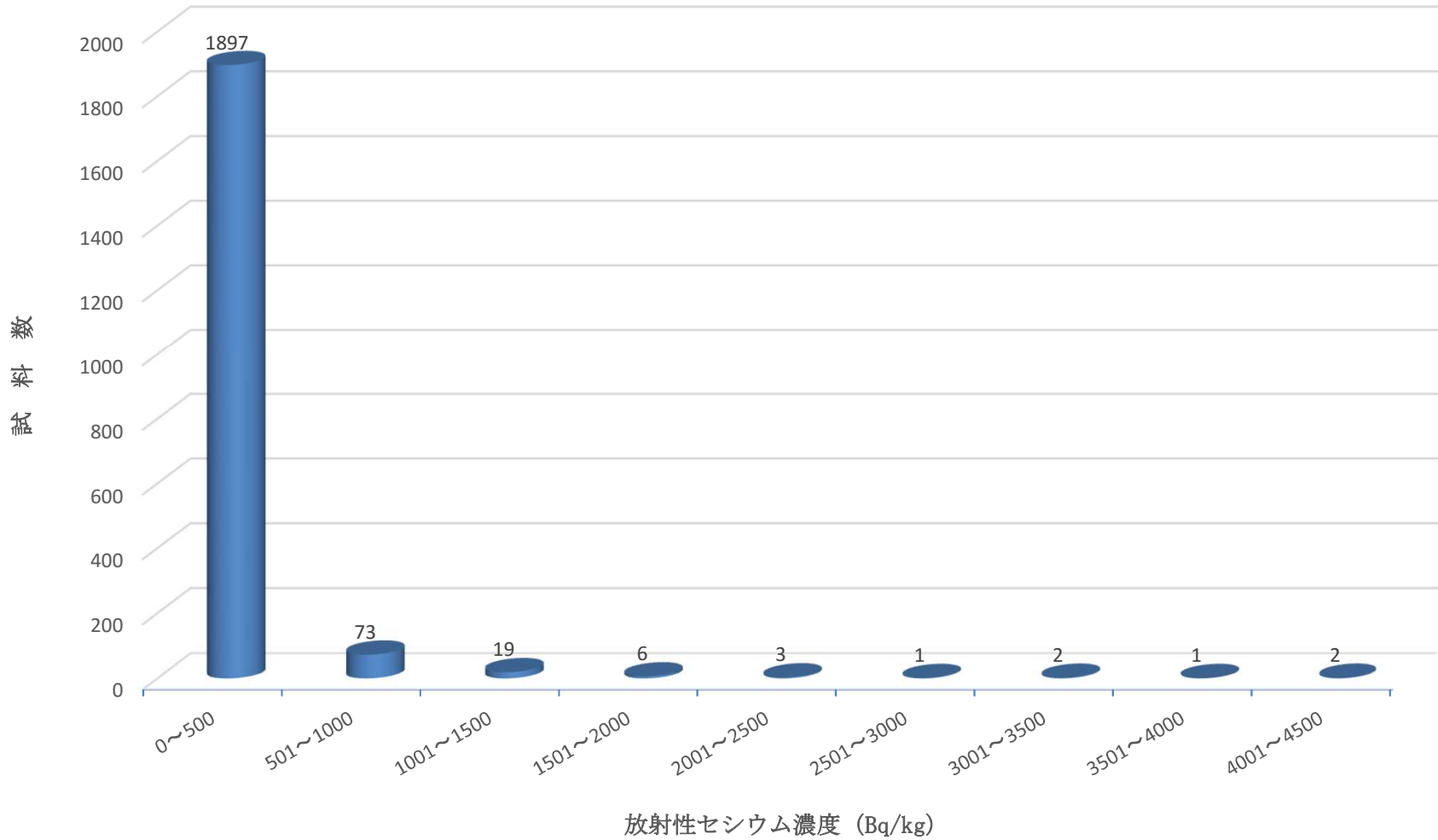
河川（底質）の放射性セシウム濃度（500Bq/kg）ごとの頻度（令和元年度）
