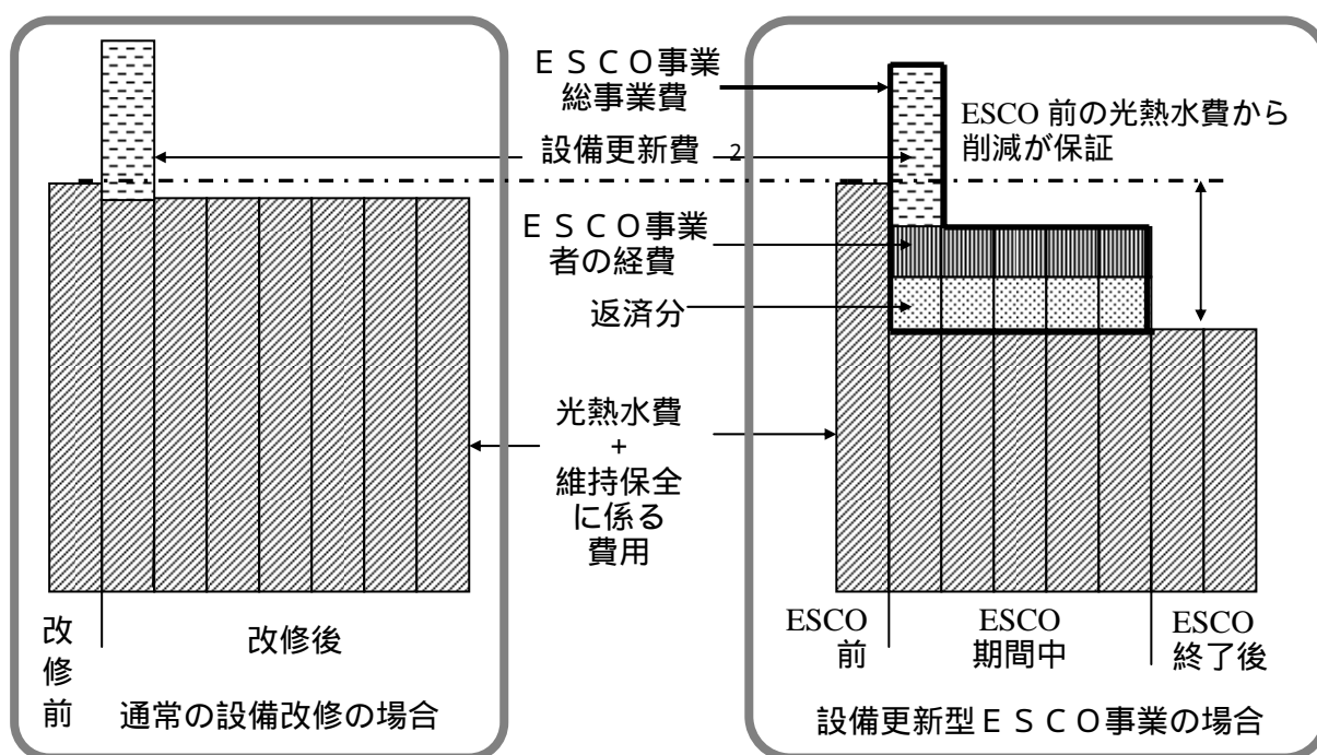
図 1 - 1 通常の設備改修と設備更新型E S C O事業についての概念図
