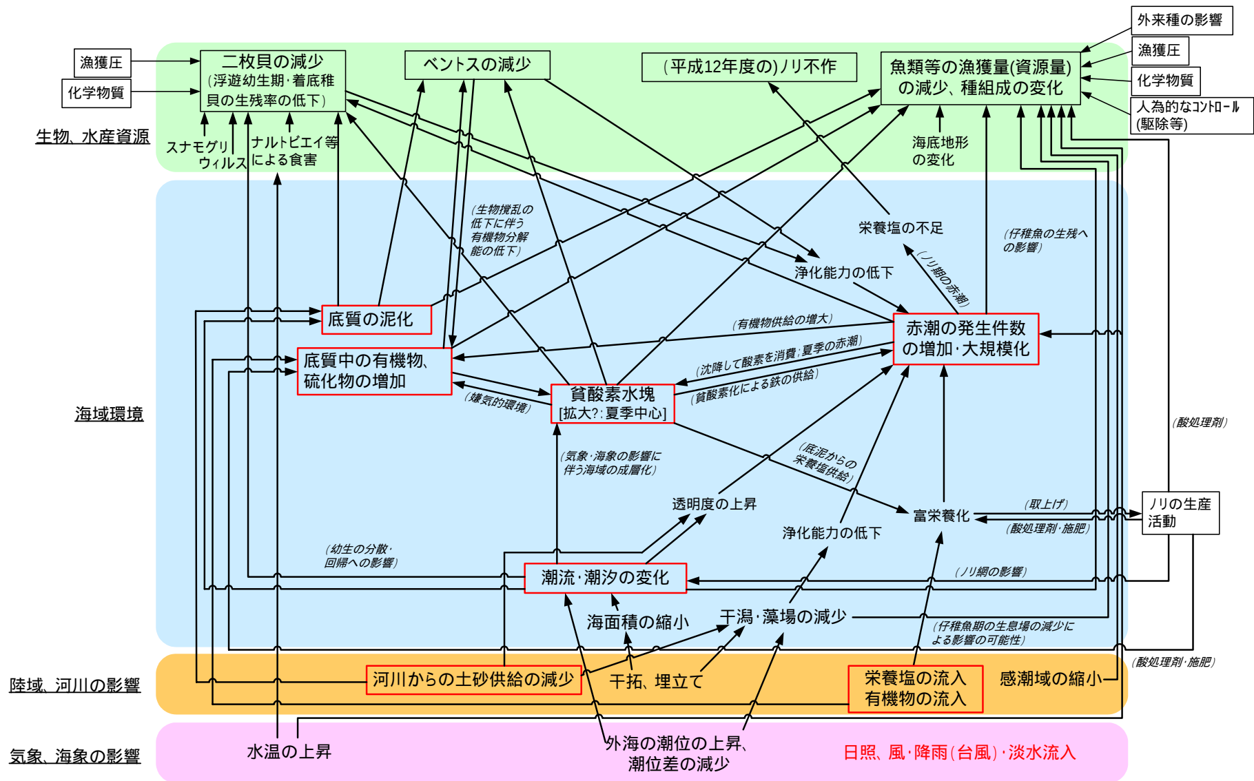
図 4.1.1 問題点と原因・要因との関連の可能性(検討中): 有明海
