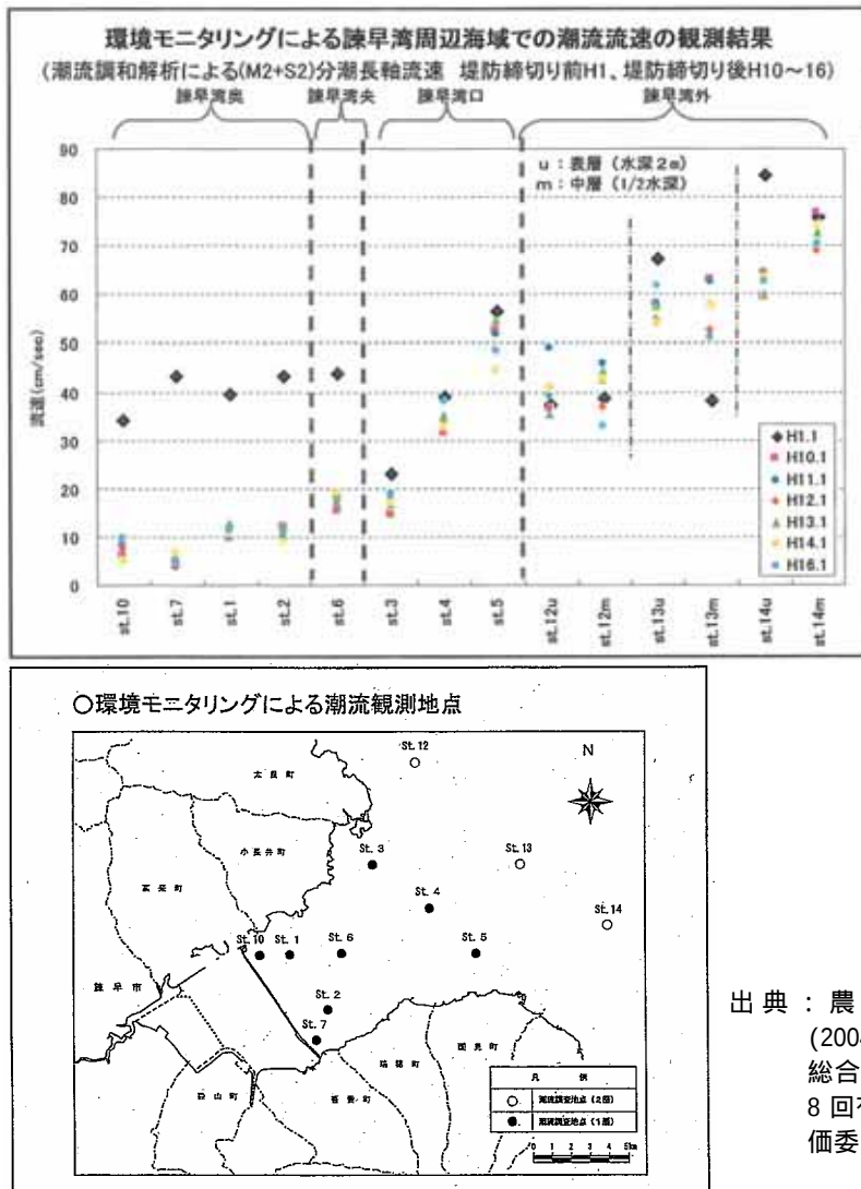
図 3.6.12 環境モニタリングによる諫早湾周辺海域での潮流流速の観測結果
