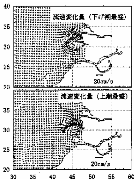
図 3.6.18 熊本新港設置前後の流速変化量
