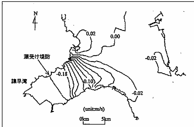
図 3.6.13 下げ潮時の流速強度に関する締め切り前後の差
