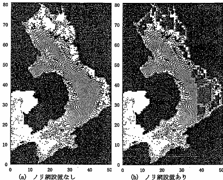
図 3.6.16 ノリ網設置の有無による流況変化（粒子追跡開始 3 潮汐後）
