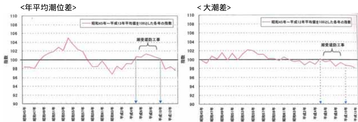
図 3.6.3 大浦検潮所における年平均潮位差と大潮差の推移
