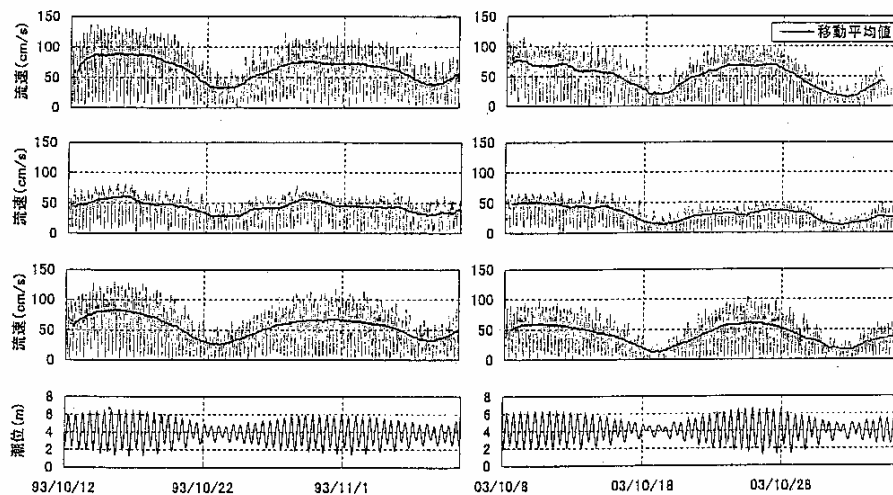
図 3.6.13 下げ潮時の流速強度に関する締め切り前後の差
