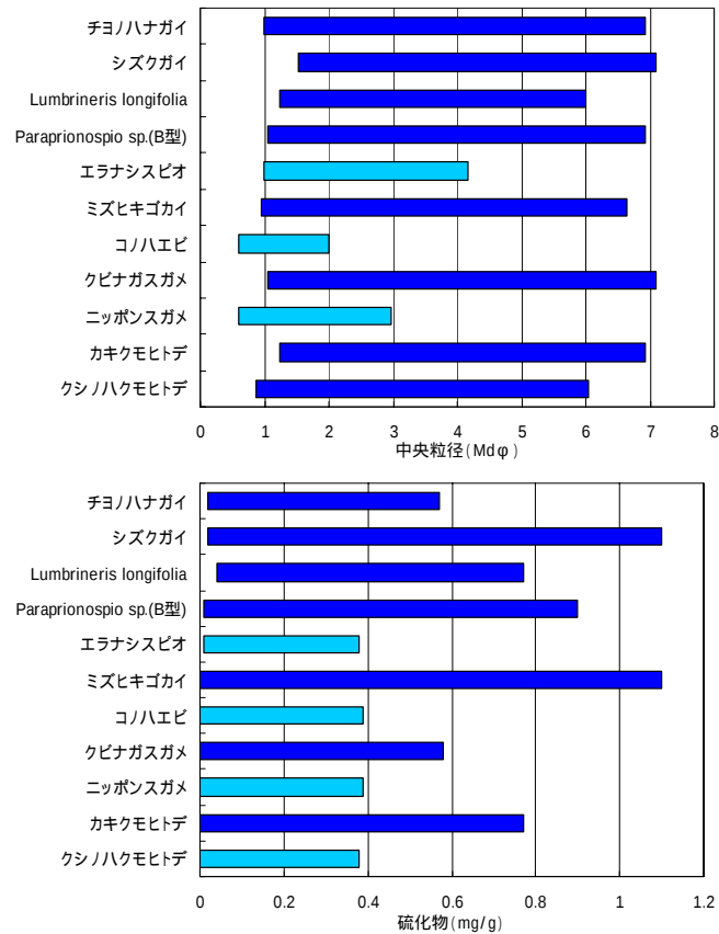
図 3.10.5 指標種の生息域における粒度組成(Md φ)と硫化物の範囲
