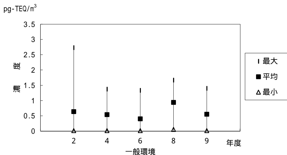
図1 ダイオキシン類の大気環境中濃度（一般環境）の経年変化
