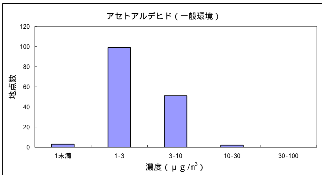
図7 アセトアルデヒドの大気環境中濃度分布
