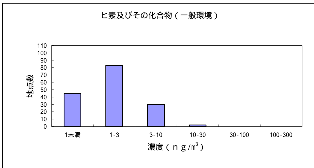
図 17 ヒ素及びその化合物の大気環境中濃度分布
