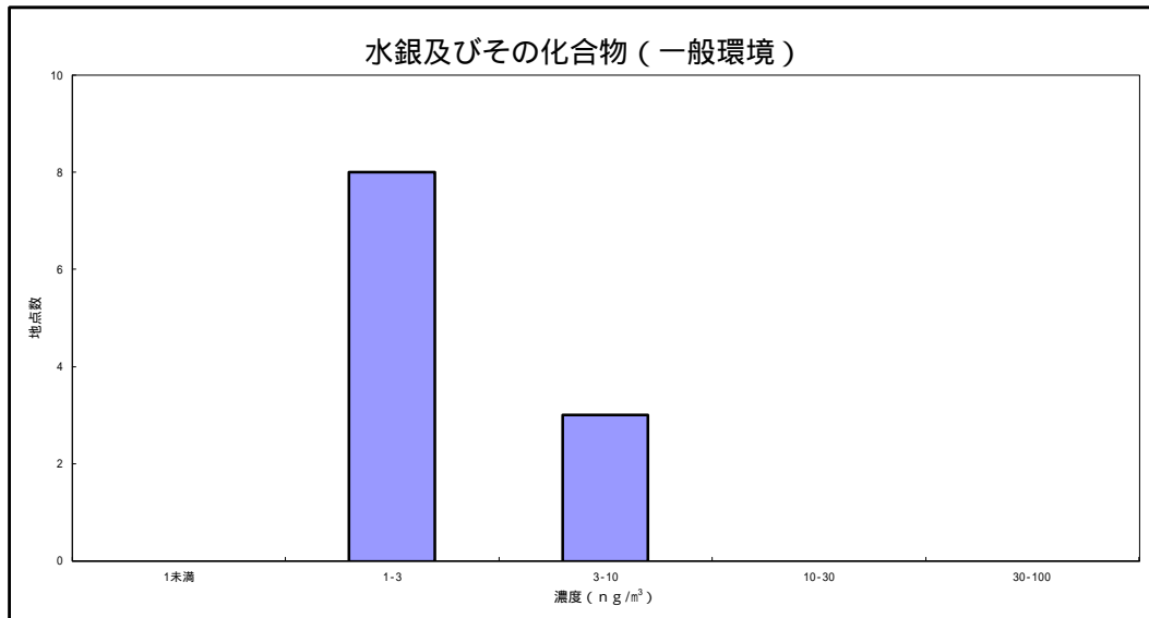
図 1 5 水銀及びその化合物の大気環境中濃度分布
