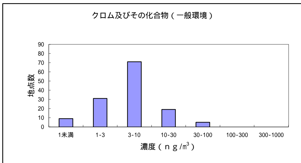
図 2 0 クロム及びその化合物の大気環境中濃度分布
