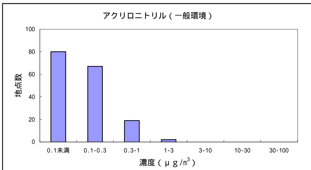
図6 アクリロニトリルの大気環境中濃度分布
