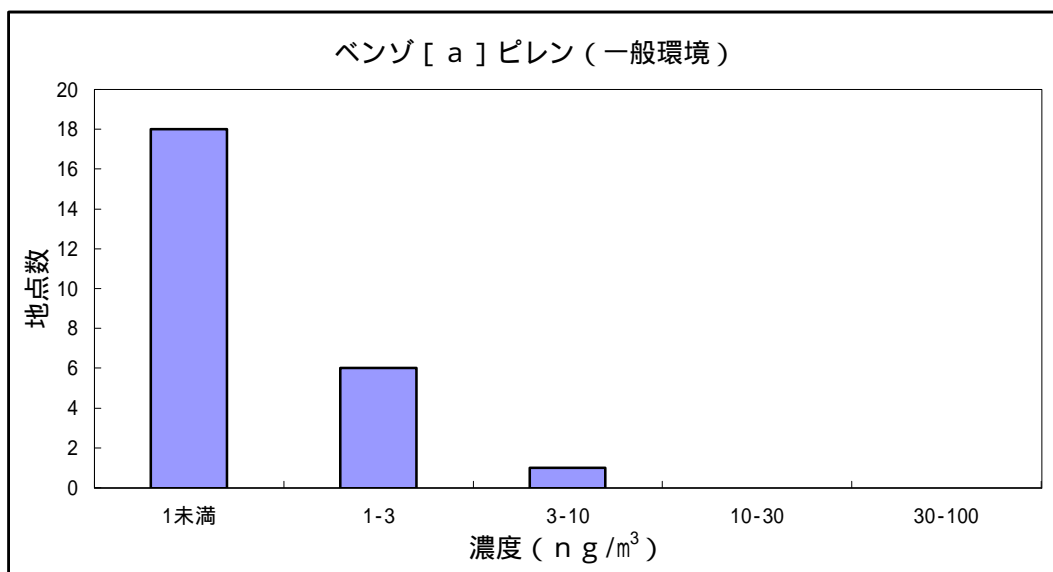
図 13 ベンゾ[ a ]ピレンの大气環境中濃度分布
