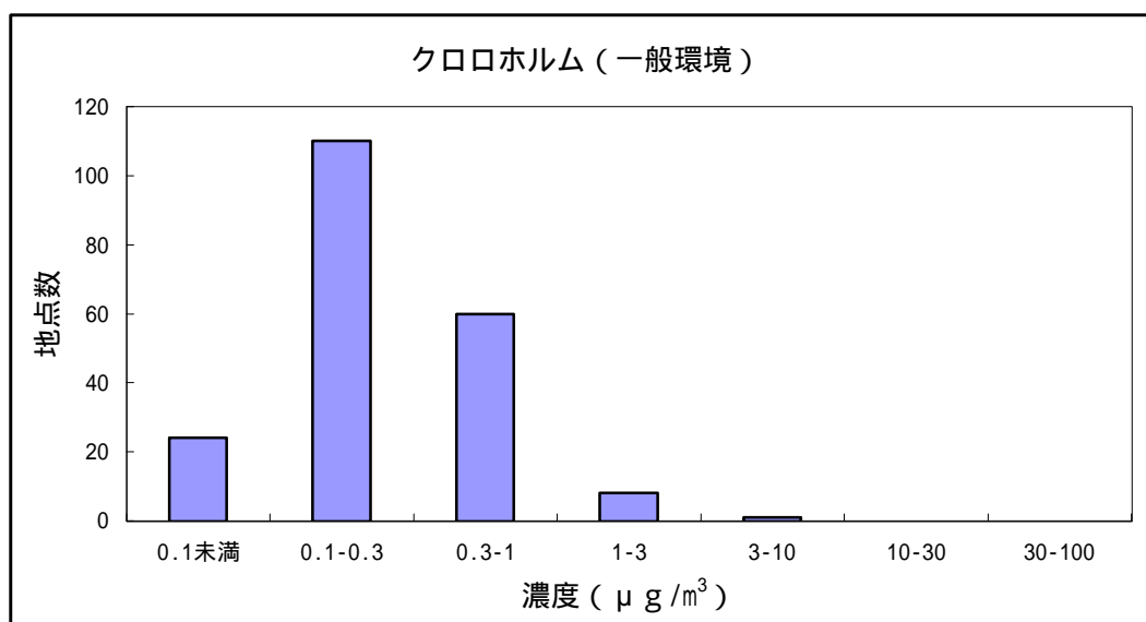
図9 クロロホルムの大気環境中濃度分布
