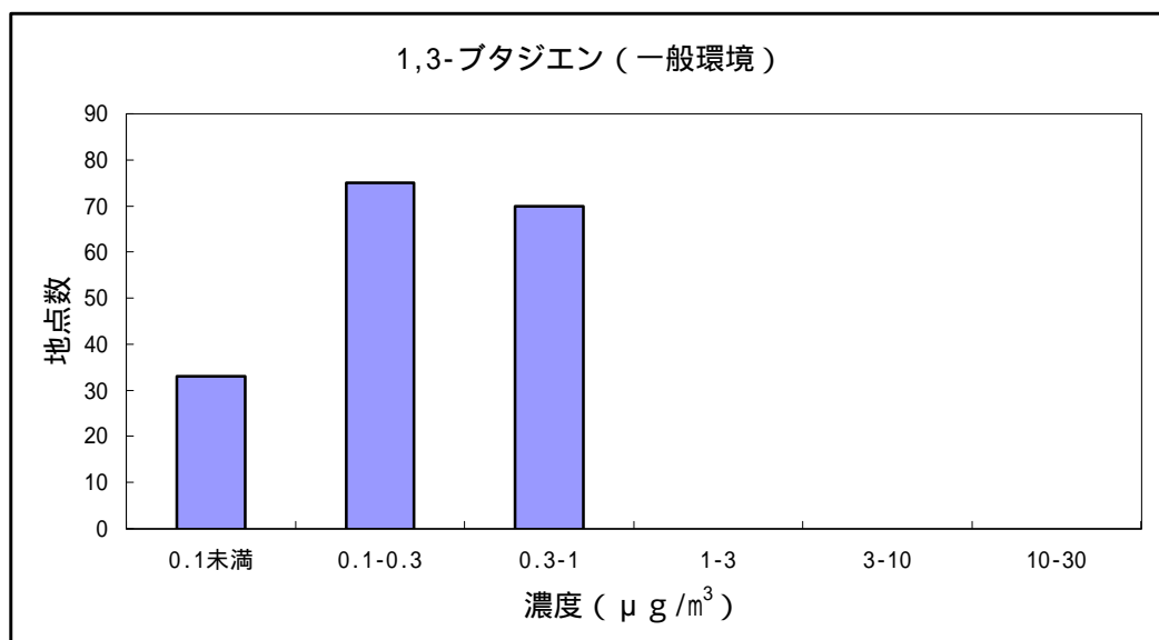
図 1 2 1,3-ブタジエンの大気環境中濃度分布
