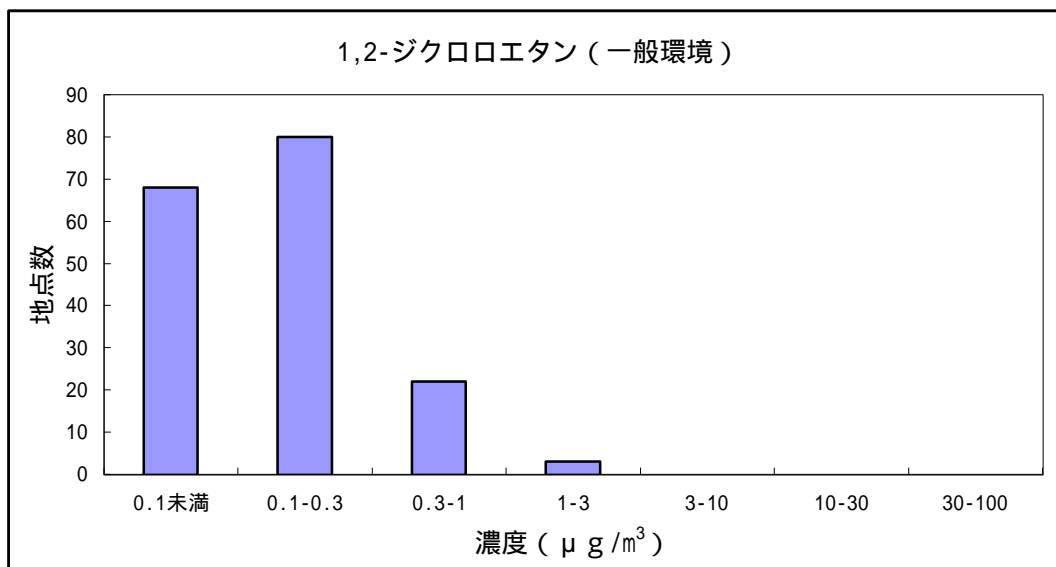
図10 1,2-ジクロロエタンの大気環境中濃度分布
