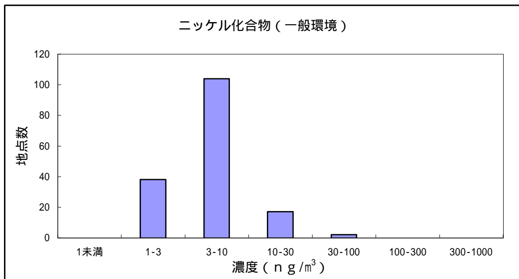
図 1 6 ニッケル化合物の大気環境中濃度分布
