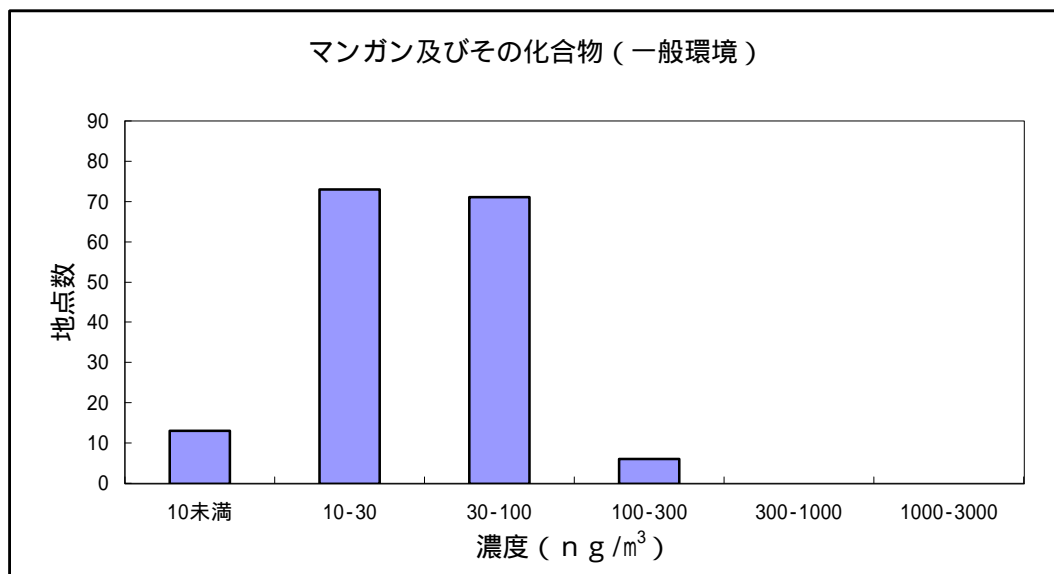
図 19 マンガン及びその化合物の大気環境中濃度分布
