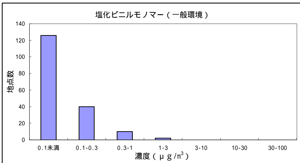
図8 塩化ビニルモノマーの大気環境中濃度分布
