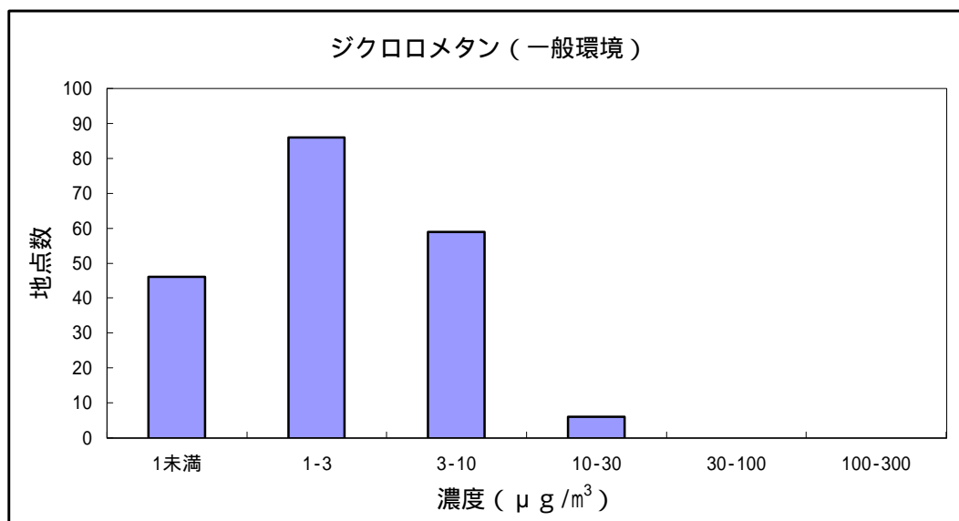
図 1 1 ジクロロメタンの大気環境中濃度分布
