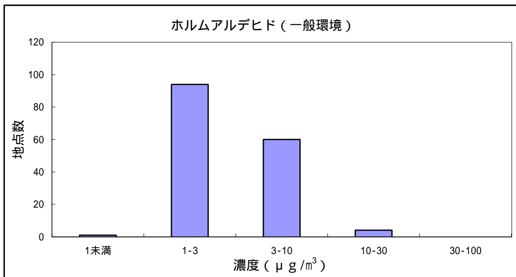
図 1 4 ホルムアルデヒドの大気環境中濃度分布
