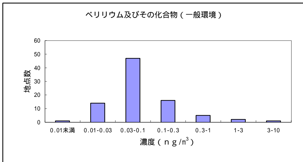
図 1 8 ベリリウム及びその化合物の大気環境中濃度分布
