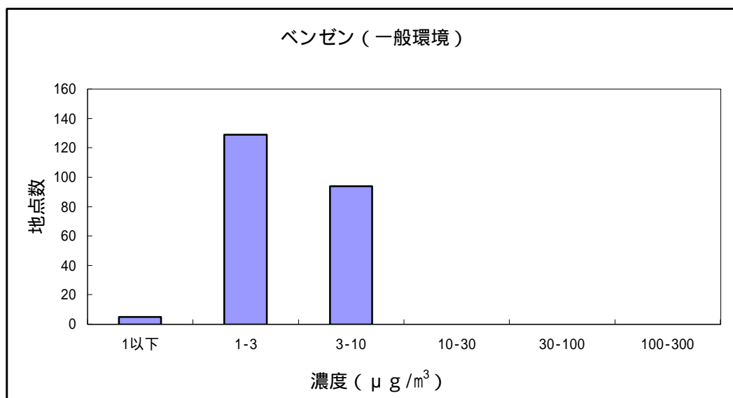
図3 ベンゼンの大気環境中濃度分布
