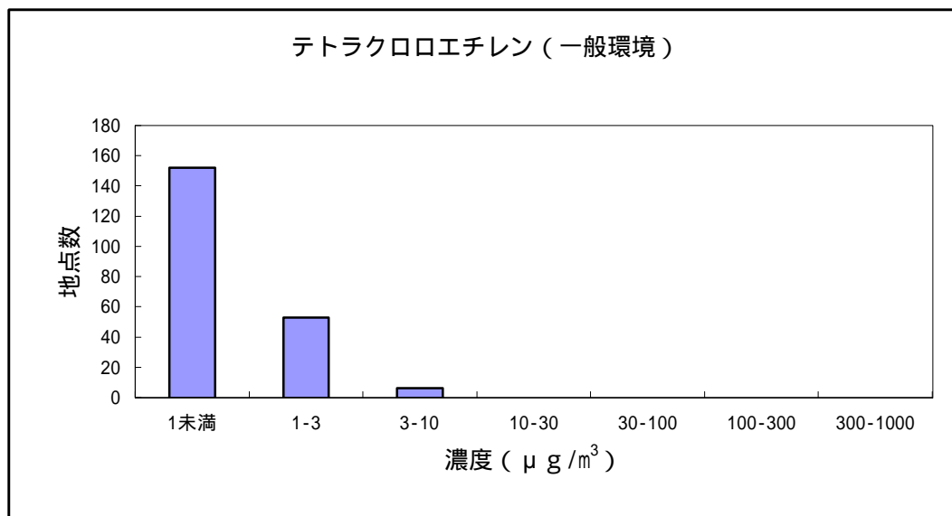
図5 テトラクロロエチレンの大気環境中濃度分布
