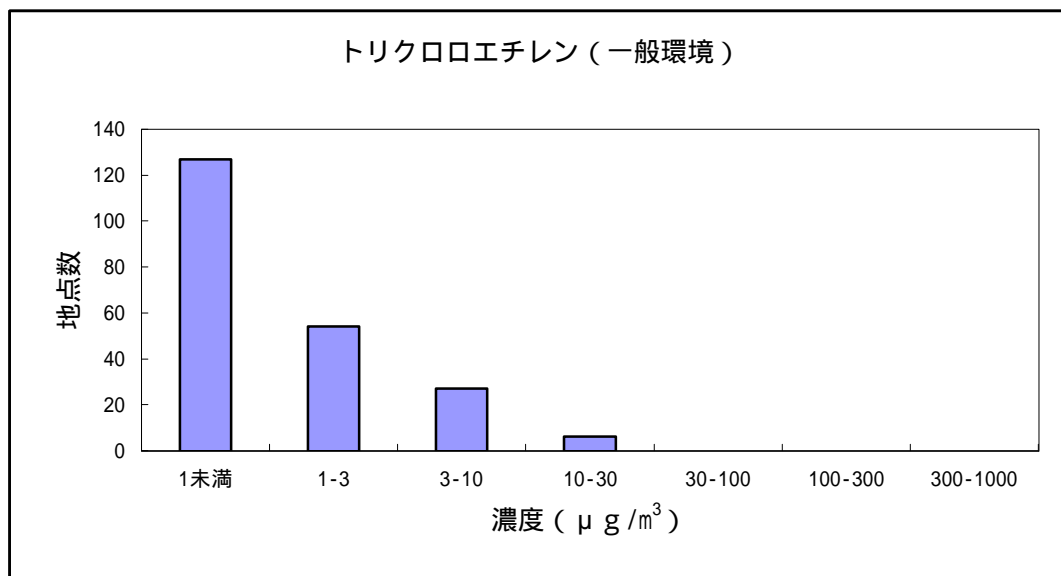
図4 トリクロロエチレンの大気環境中濃度分布
