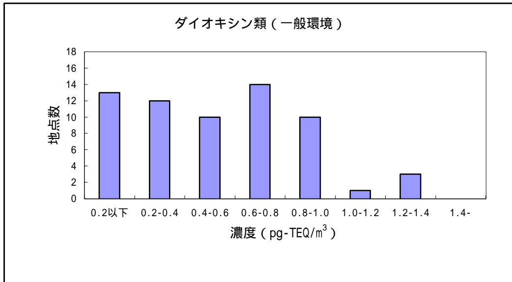
図2 ダイオキシン類の大気環境中濃度分布 (夏冬を含む年2回以上の測定)
