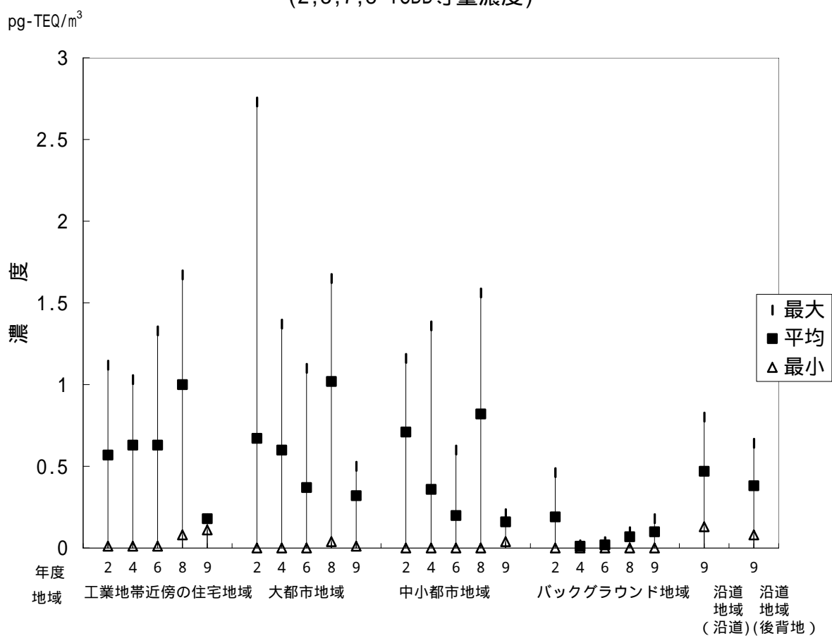
図 ダイオキシン類大気環境濃度調査結果の経年変化 (2,3,7,8-TCDD等量濃度)
