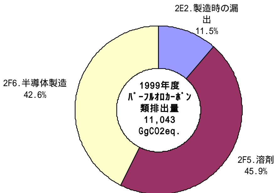
図 2.7 ハイドロフルオロカーボン類の実排出量内訳 (1999 年度)
