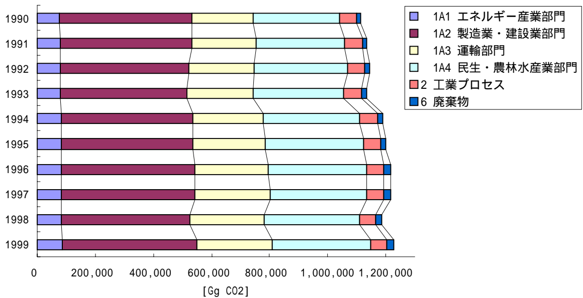
図 2.3 二酸化炭素の部門別排出量 (1990 - 1999 年度)
