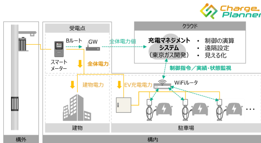
EV充電マネジメントシステム イメージ
