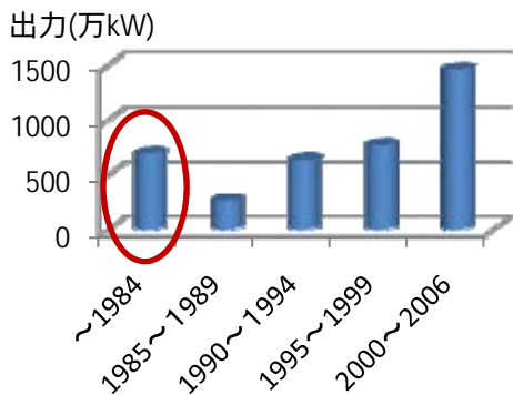
石炭火力発電所の設置年別出力
