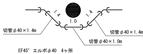
f 部詳細図 1ヶ所
