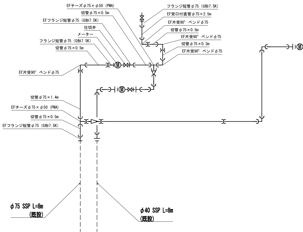
d 部詳細図
