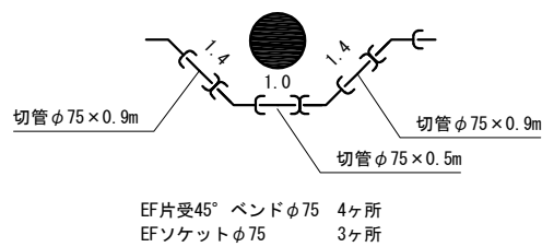
a 部詳細図 10ヶ所
