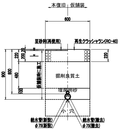
砂利舗装22型
