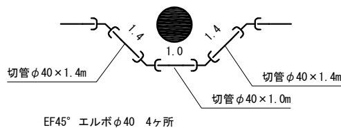
e 部詳細図 5ヶ所
