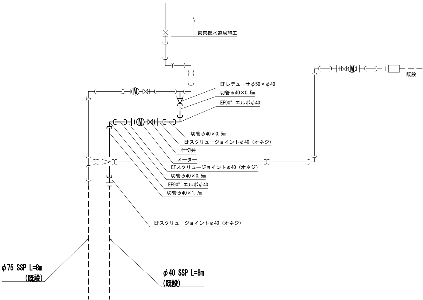
d 部詳細図
