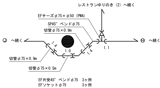
c 部詳細図
