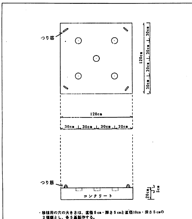
図 6-16. 人工基盤図
