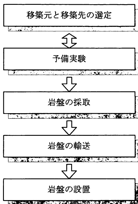
図 5・1. サンゴ群集の移築工程(港湾空間高度化センター 1999 より)
