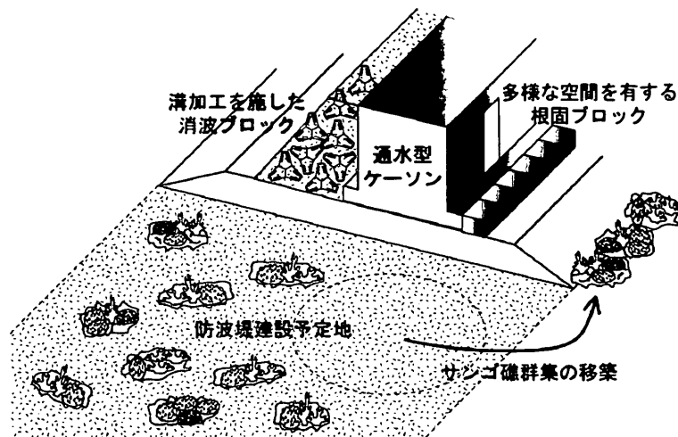
図 5-6. 平良港における環境共生型防波堤の概要（石井ほか 2001 より）
