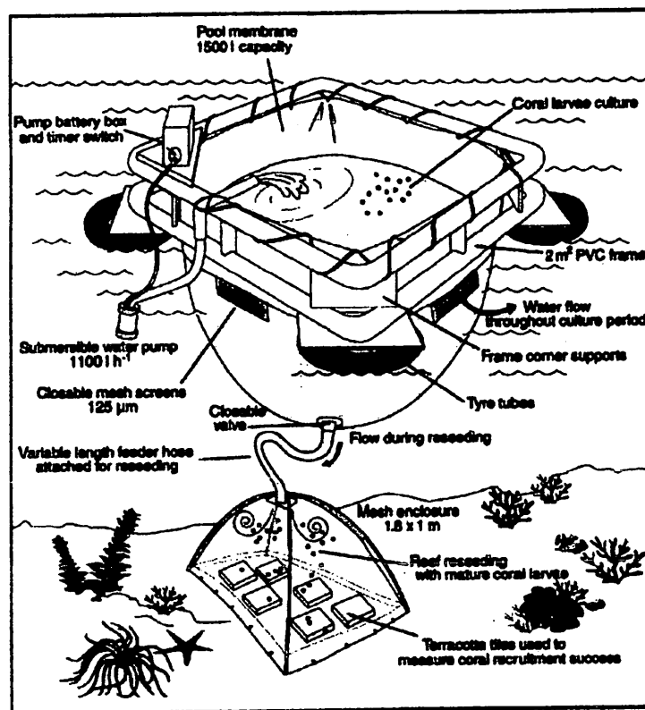
図 3-10. 生け簀から海底のテントへ幼生を導入する方法の例 (Heyward et al. 2002 より)
