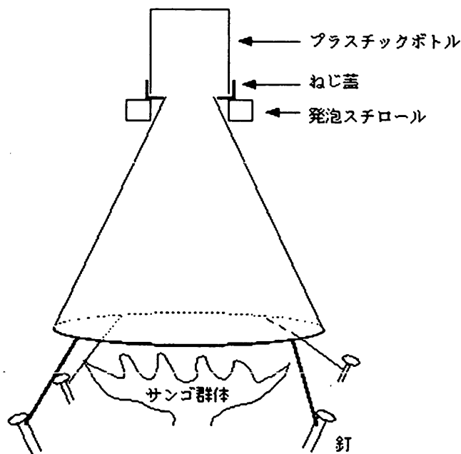
図 3-2. バンドル・コレクターの概略
