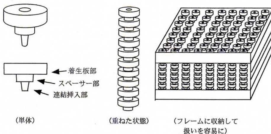
図 6-3. サング着生具と組み立て法
