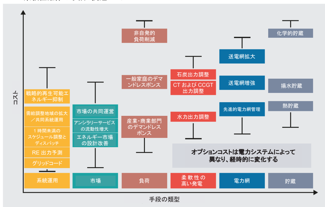
図 1.11 柔軟性確保の手段と関連コスト
