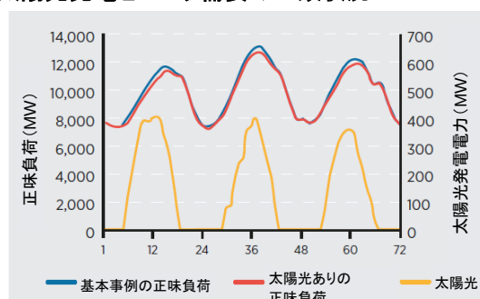
図 2.27 コロラド州における太陽光発電とピーク需要の一致状況
