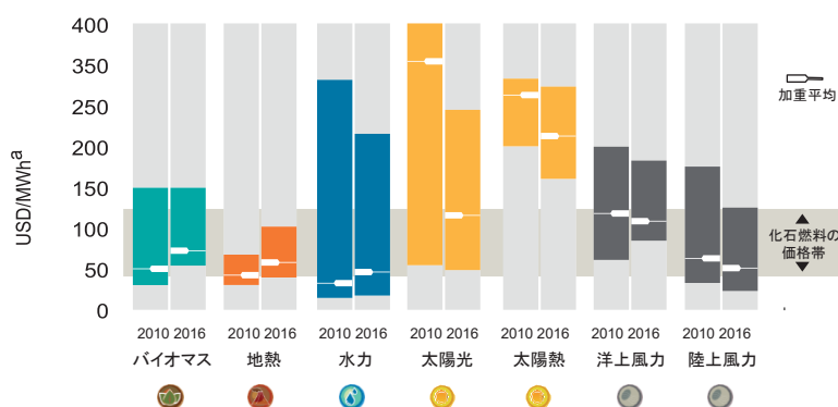
図 1.1 2010 年および 2016 年における事業用発電所の均等化発電原価(LCOE) (平均および範囲)
