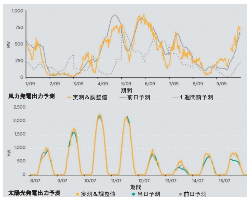
図 1.9 ベルギーにおける風力発電および太陽光発電出力予測
