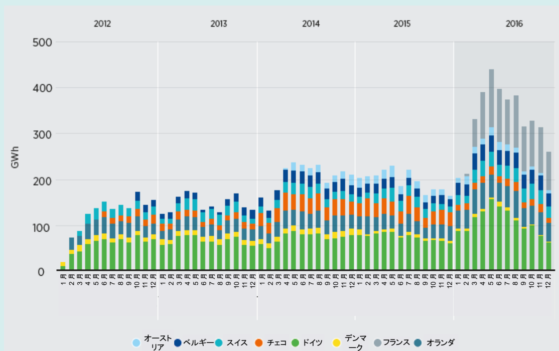
図 2.13 インバランス相殺プロセスの国際系統管理協力機構全メンバーに関する月間相殺量
