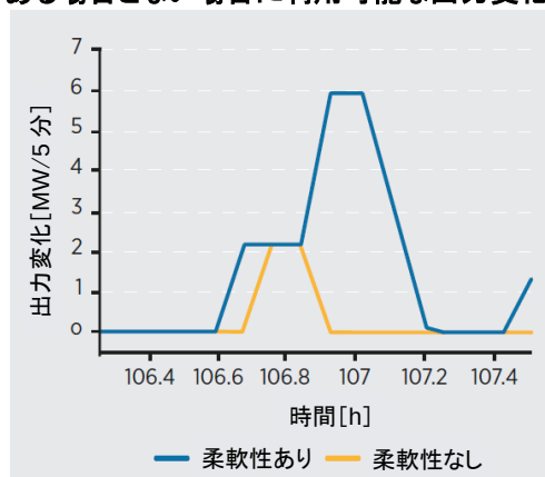
図 2.23 柔軟性予備力商品がある場合とない場合に利用可能な出力変化容量
