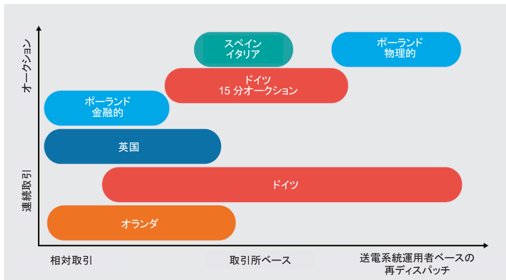
図 2.7 欧州各国における当日取引の形態
