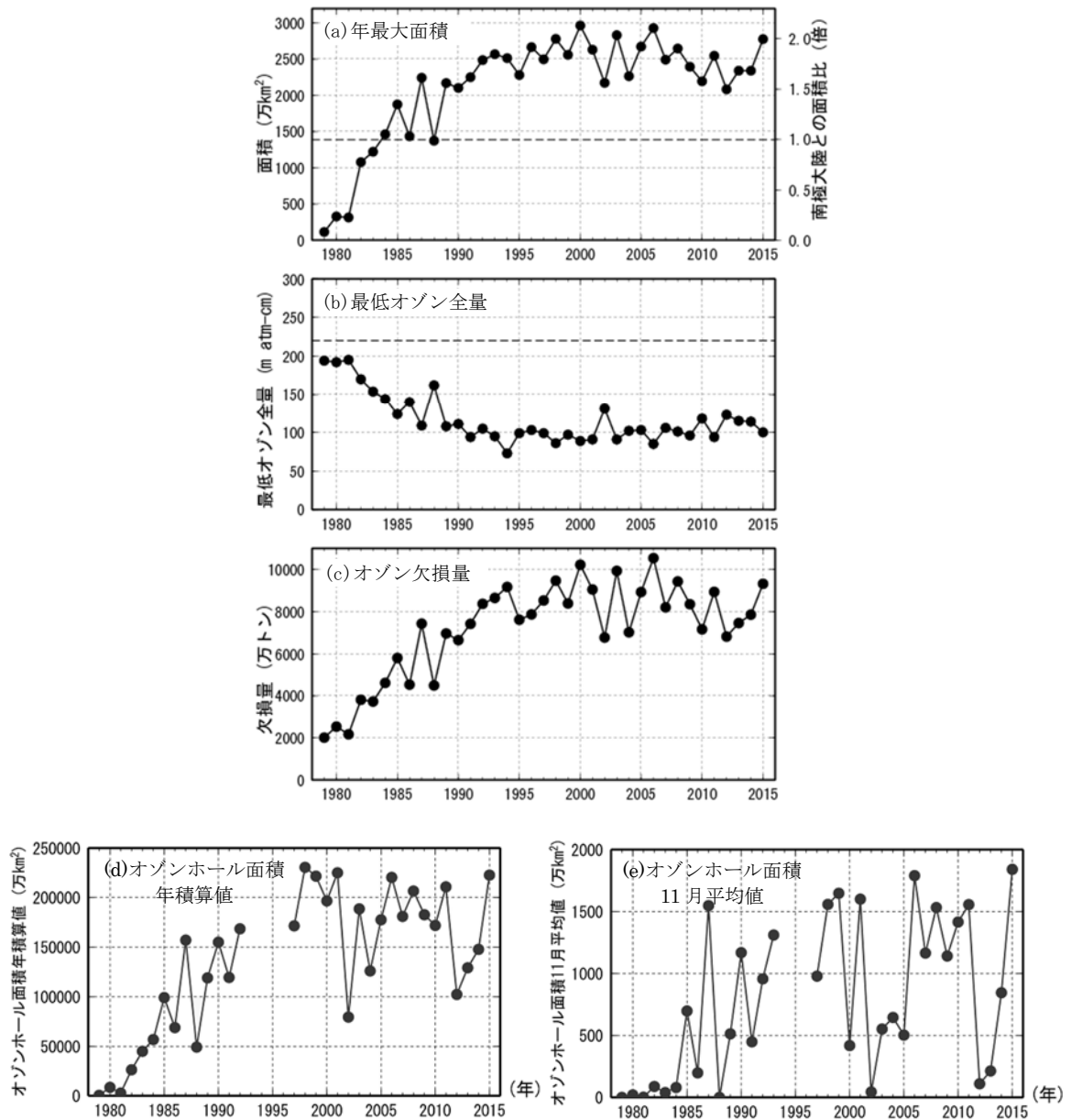
図 1-3-12 オゾンホールの規模の経年変化（1979～2015 年）
