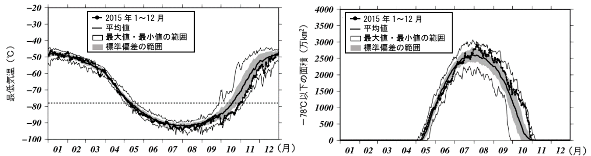
図 1-3-11 南極域上空の下部成層圏の最低気温（左）及び気温が -78^{\circ}\text{C} 以下の領域の面積（右）の推移（2015 年 1 月～2015 年 12 月）
