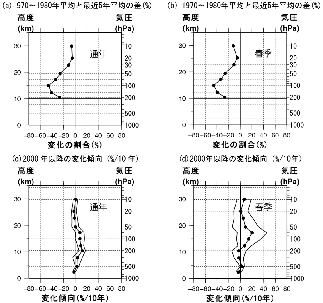
図1-3-14 南極昭和基地におけるオゾン分圧のトレンドの高度分布
