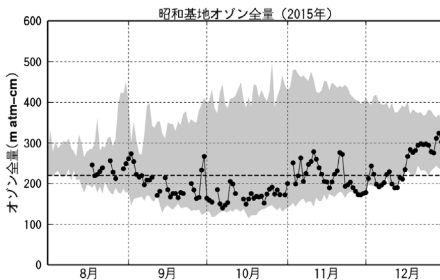
図 1-3-10 南極昭和基地における日別オゾン全量の推移（2015年8月～2015年12月）
