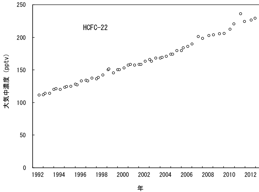
図 2-3-5 北海道における HCFC-22 の大気中のバックグラウンド濃度の経年変化 (出典) 環境省 平成 24 年度フロン等オゾン層影響微量ガス等監視調査より
