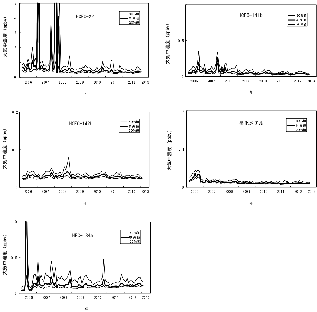
図 2-3-16 川崎市における特定物質等の月別濃度（中央値）の経年変化（続き） (出典) 環境省 平成 17 年度フロン等オゾン層影響微量ガス等監視調査 及び平成 24 年度フロン等オゾン層影響微量ガス等監視調査より
