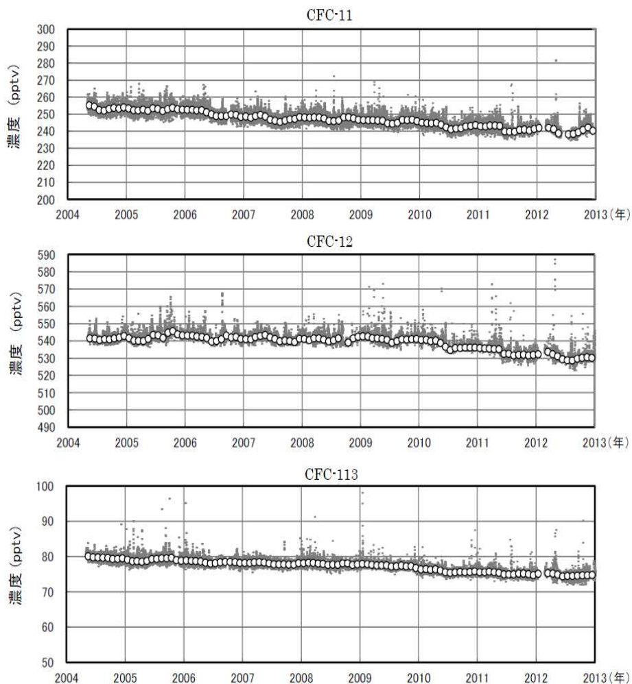
図 2-3-8 波照間島で観測された CFC-11、CFC-12 及び CFC-113 濃度の経年変化
