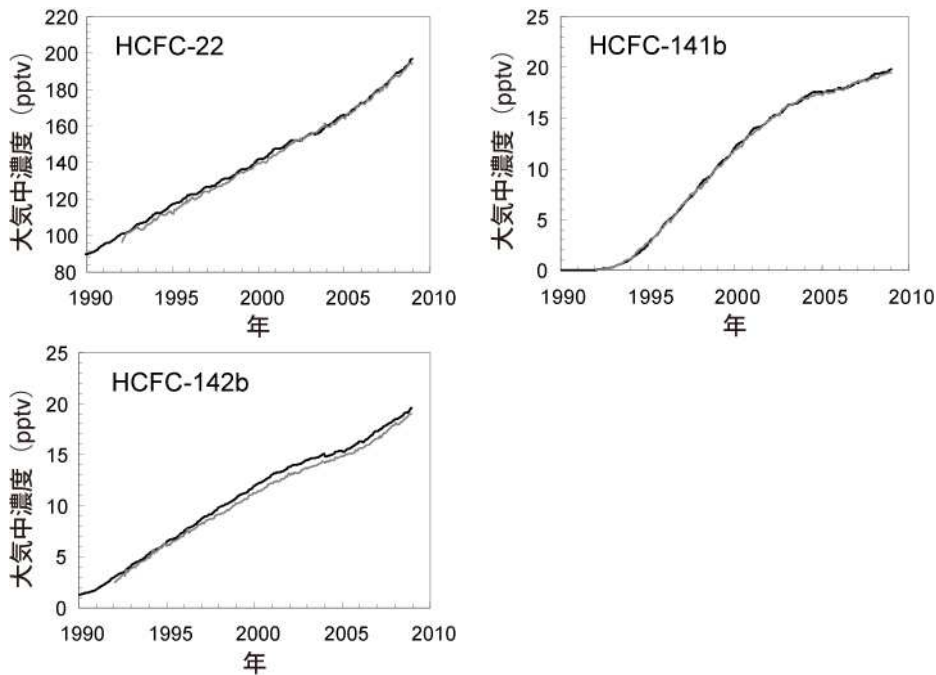
図 2-3-14 海外のネットワークで観測された HCFC-22、HCFC-141b 及び HCFC-142b の濃度変化 各観測ネットワークによる観測結果。NOAA による観測結果を薄い灰色、AGAGE による観測結果を濃い灰色で示している。 (出典) Scientific Assessment of Ozone Depletion: 2010 (WMO, 2011) より作成
