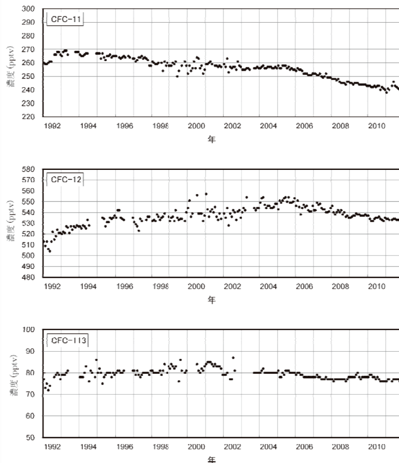
図 2-3-9 岩手県大船渡市綾里における大気中のクロロフルオロカーボン類濃度の経年変化 綾里における大気中の CFC-11（上）、CFC-12（中）、CFC-113（下）の地上での月平均濃度（測定結果を月平均したもの）の経年変化を示す。なお、データのない期間は、主に観測機器の更新や較正作業のための欠測である。また、観測精度を向上させるため、2003 年 9 月から放射線源を用いた電子捕獲型検出器（ECD）を搭載したガスクロマトグラフを導入したことにより、観測濃度データのばらつきがそれ以前と比較して少なくなっている。※口絵 IV 参照。口絵では、水色で表している。
