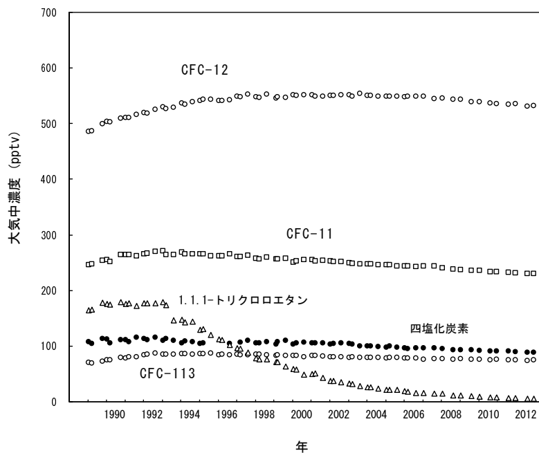
図 2-3-1 北海道における特定物質の大気中のバックグラウンド濃度の経年変化
