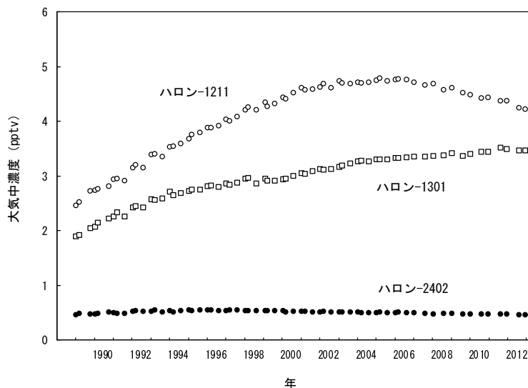
図 2-3-4 北海道におけるハロン類の大気中のバックグラウンド濃度の経年変化
