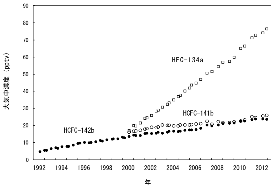
図 2-3-6 北海道における HCFC-141b、HCFC-142b 及び HFC-134a の大気中のバックグラウンド濃度の経年変化 (出典) 環境省 平成 24 年度フロン等オゾン層影響微量ガス等監視調査より
