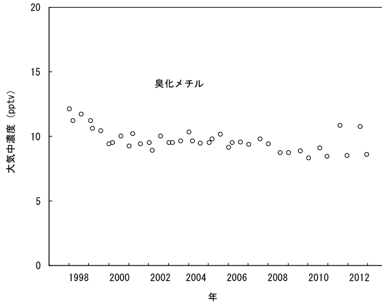
図 2-3-7 北海道における臭化メチルの大気中のバックグラウンド濃度の経年変化 (出典) 環境省 平成 24 年度フロン等オゾン層影響微量ガス等監視調査より
