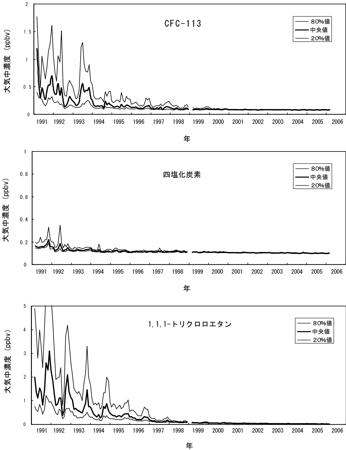
図 2-3-16 川崎市における特定物質等の月別濃度（中央値）の経年変化（続き）
