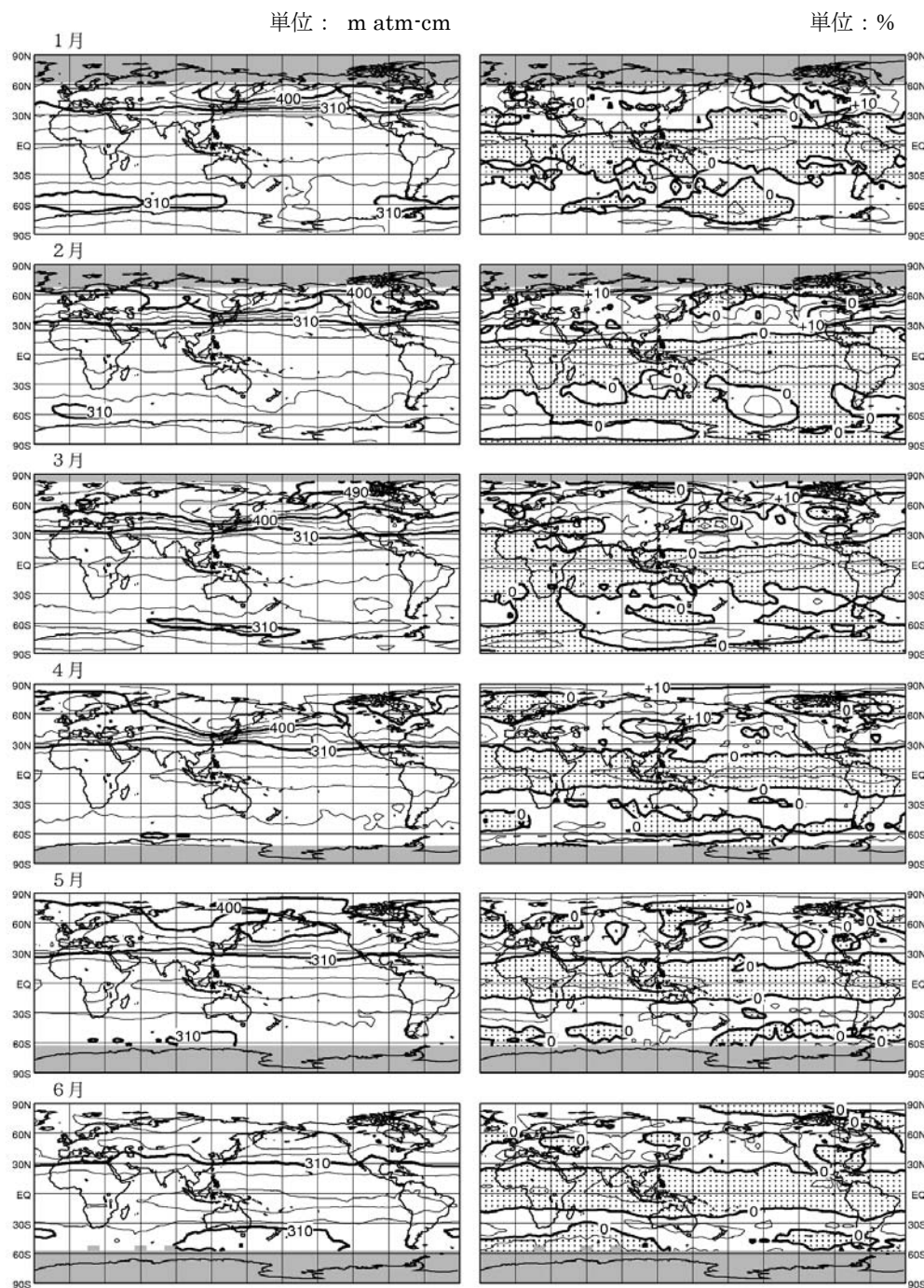
図1-資-1 月平均オゾン全量・偏差(%)の地球規模の分布図(2010年1-6月) (出典) 気象庁 オゾン層観測報告:2010
