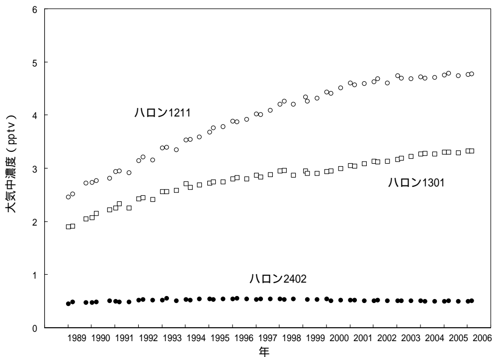
図 33 北海道におけるハロン 1211、ハロン 1301 及びハロン 2402 の大気中平均濃度の経年変化 各プロットは各月の測定結果の平均値 (n = 4~6、n は 1 プロット当たりの試料数) (出典) 環境省 平成 17 年度フロン等オゾン層影響微量ガス監視調査
