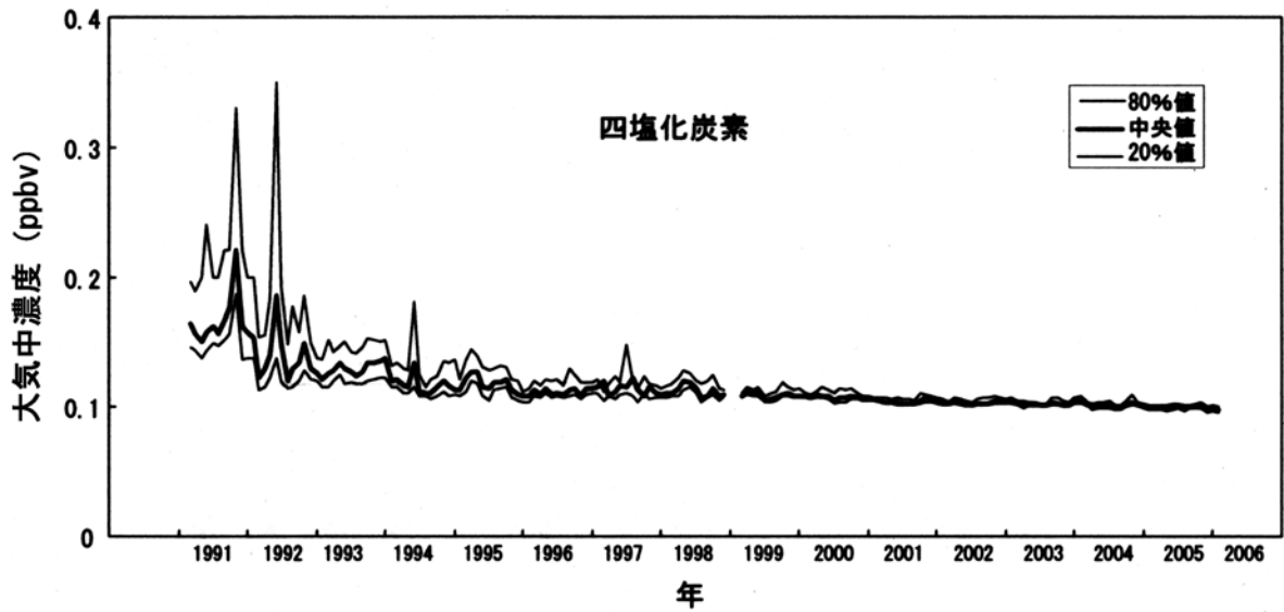
図 39-2 川崎市における特定物質の月別濃度の推移 (出典) 環境省 平成 17 年度フロン等オゾン層影響微量ガス監視調査
