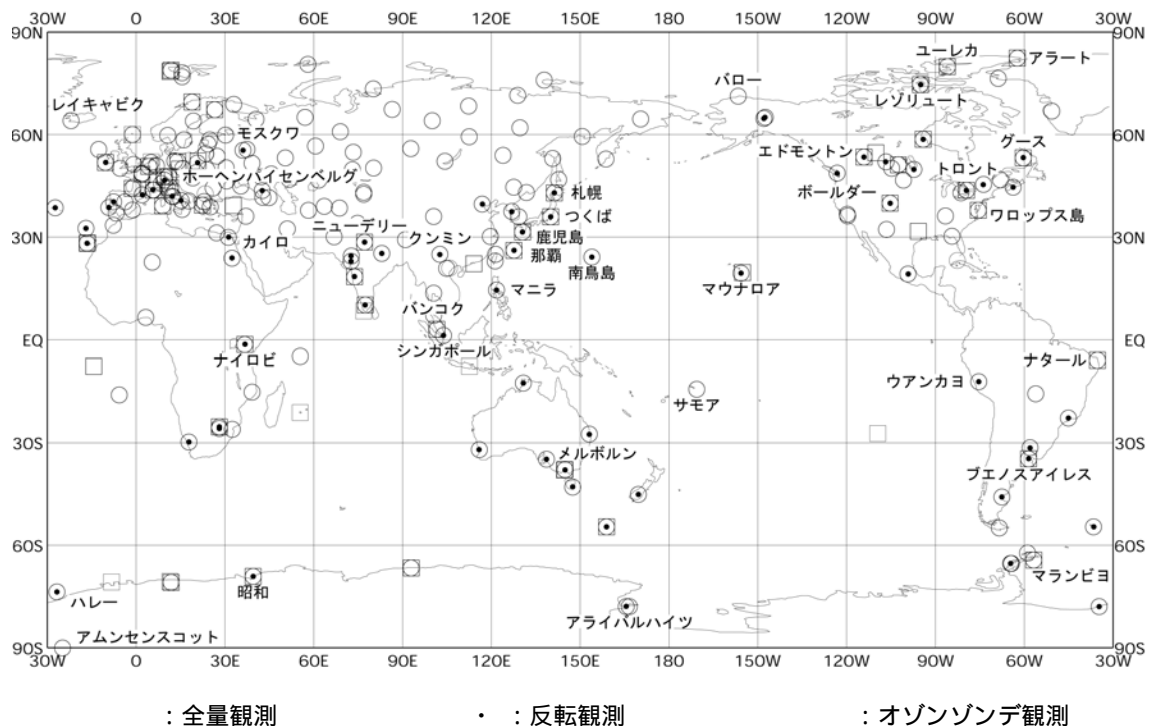
図53 世界のオゾン観測所の分布 (2004年現在)
