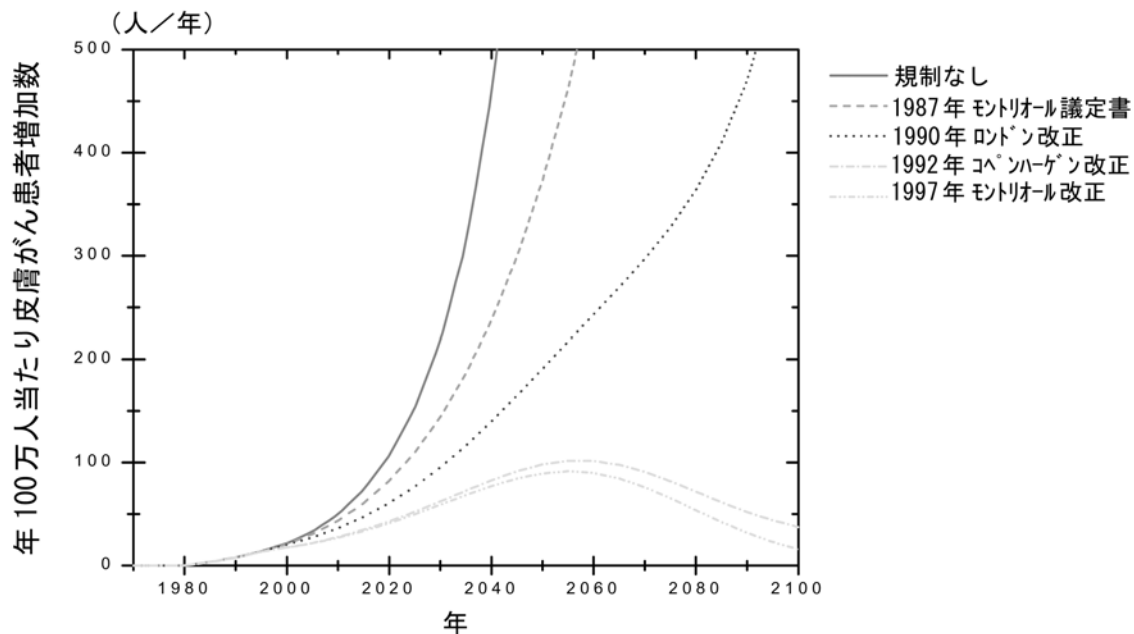
図 51 様々なシナリオに基づいた皮膚がんのリスク評価 (出典) UNEP 環境影響パネル報告書 1998
