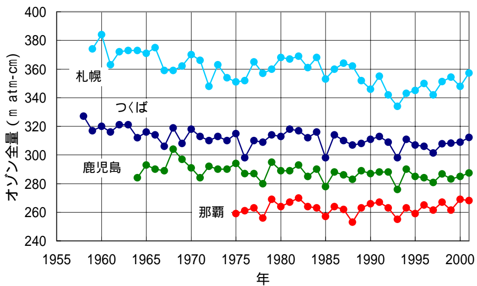
図 日本上空のオゾン全量の年平均値の変化 出典：気象庁提供データ
