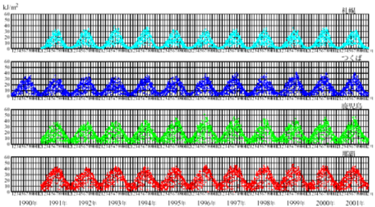
図 UV-B 量の日積算値の変化 出典：気象庁提供データ
