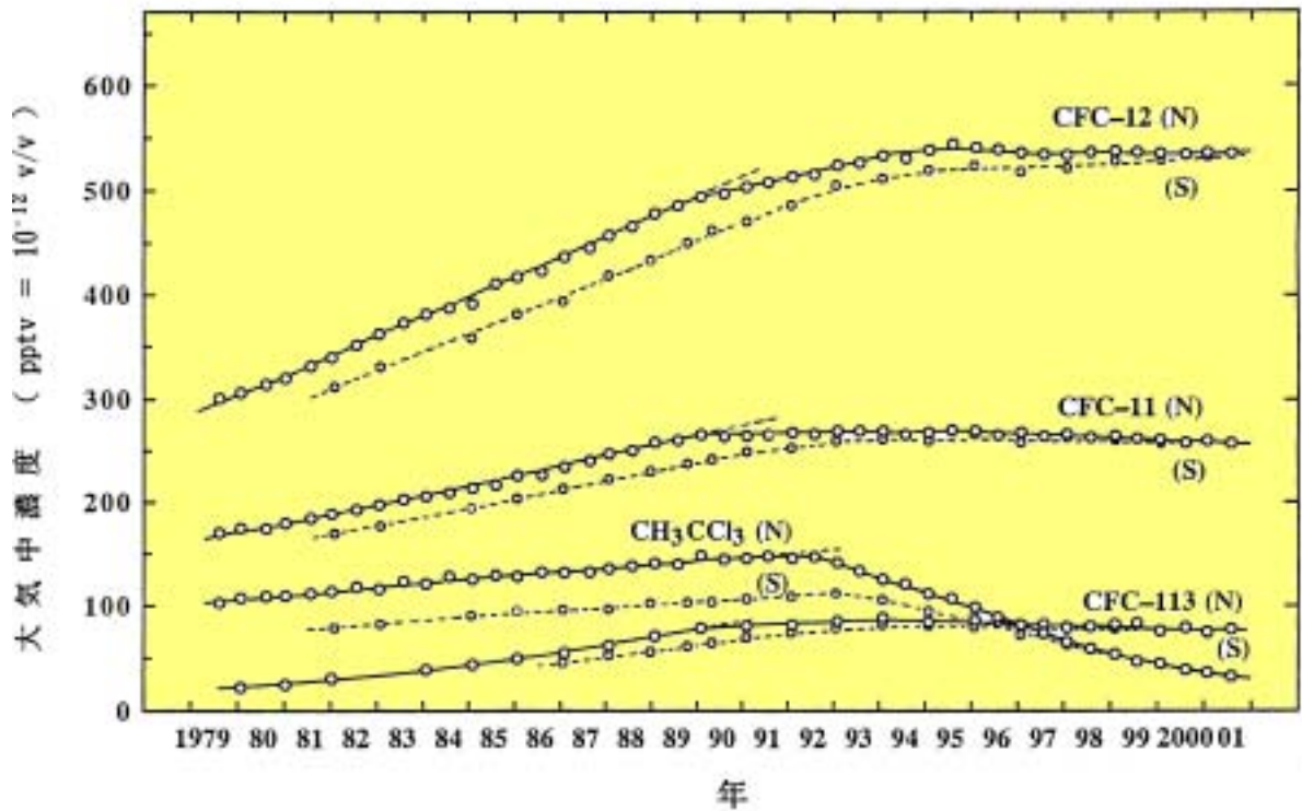
図 北半球中緯度（北海道:N）及び南半球（南極昭和基地:S）における 特定物質の大気中平均濃度の経年変化 出典：東京大学巻出教授提供データ
