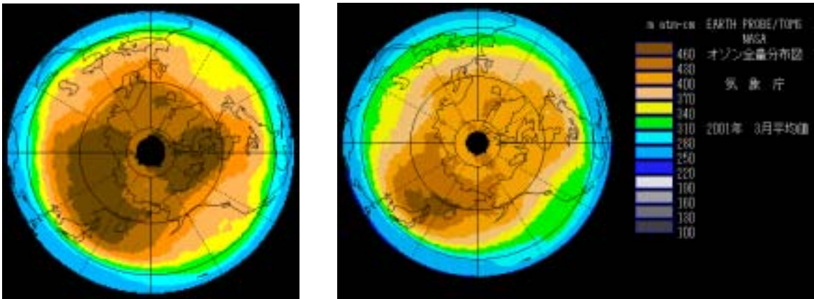
図 1979年、2001年それぞれ3月の月平均オゾン全量の北半球分布 出典：気象庁提供データ
