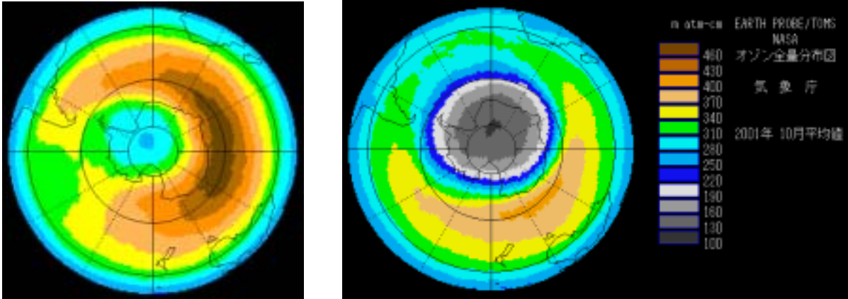
図 1979年、2001年それぞれ10月の月平均オゾン全量の南半球分布 出典：気象庁提供データ
