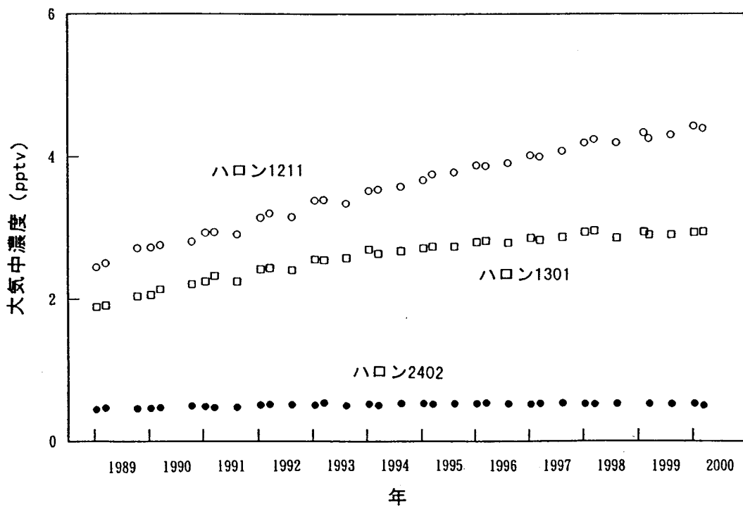
図 36 北海道におけるハロン 1211、ハロン 1301 及びハロン 2402 の大気中平均濃度の経年変化 各プロットは各月の測定結果の平均値 ( n = 4 ~ 6 ) ( 出典 ) 環境省調査
