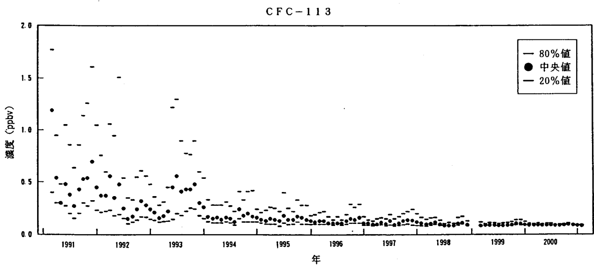
図 39 - 1 川崎市における特定物質の月別濃度の推移
