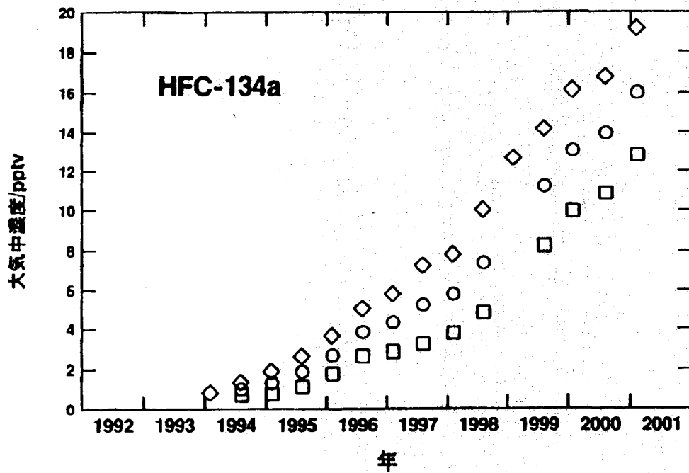
図 33 北半球中緯度 (北海道)及び南半球(南極昭和基地)における H F C -134 a の大気中平均濃度の経年変化
