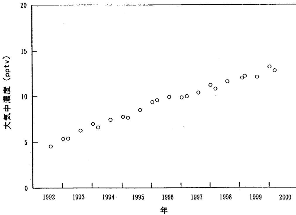
図 38 北海道におけるH C F C -142b の大気中平均濃度の経年変化
