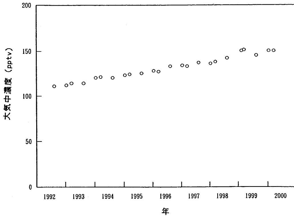
図 37 北海道におけるH C F C -22 の大気中平均濃度の経年変化
