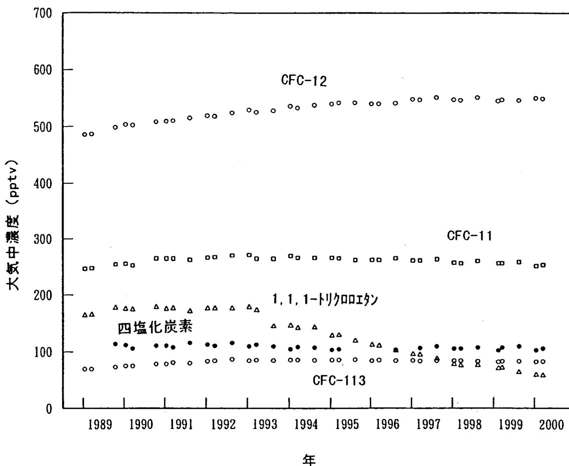
図34 北海道における特定物質の大気中平均濃度の経年変化
