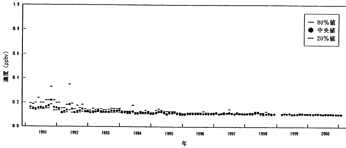
図 39 - 2 川崎市における特定物質の月別濃度の推移
