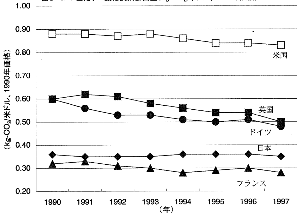
図3 GDP当たり二酸化炭素排出量(kg-CO 2 /米ドル、1990年価格)
