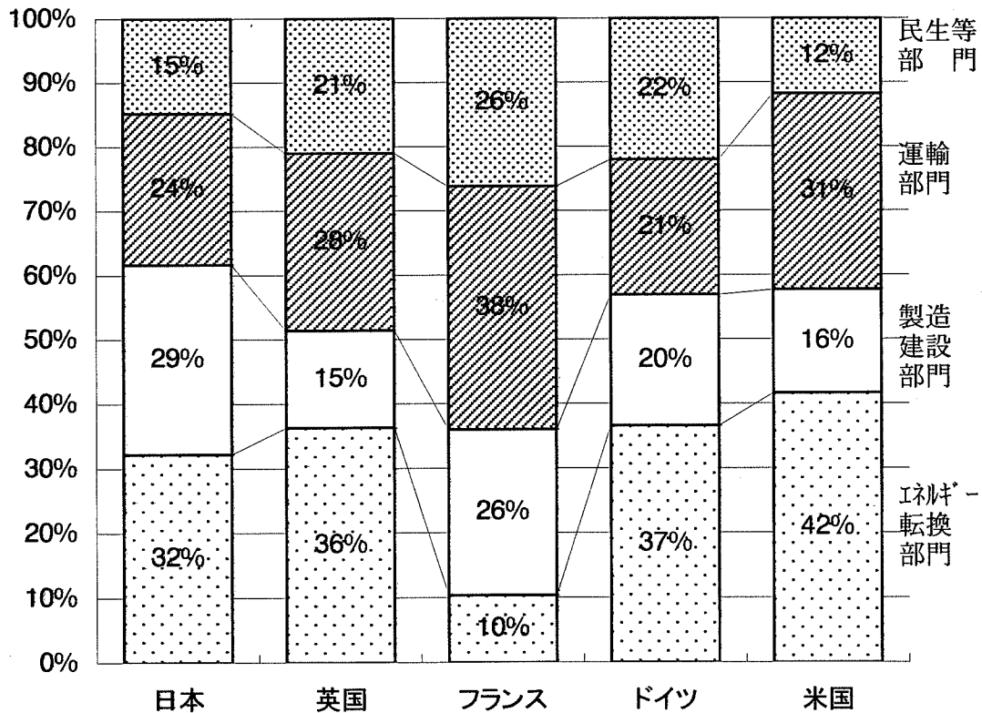
図6 各国の部門別二酸化炭素排出量 (1997年)
