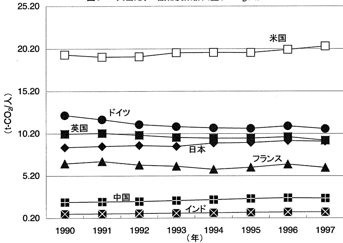
図5 一人当たり二酸化炭素排出量(t-CO 2 /人)
