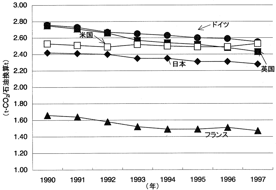
図4 一次エネルギー供給当たり二酸化炭素排出量(t-CO 2 /石油換算t)
