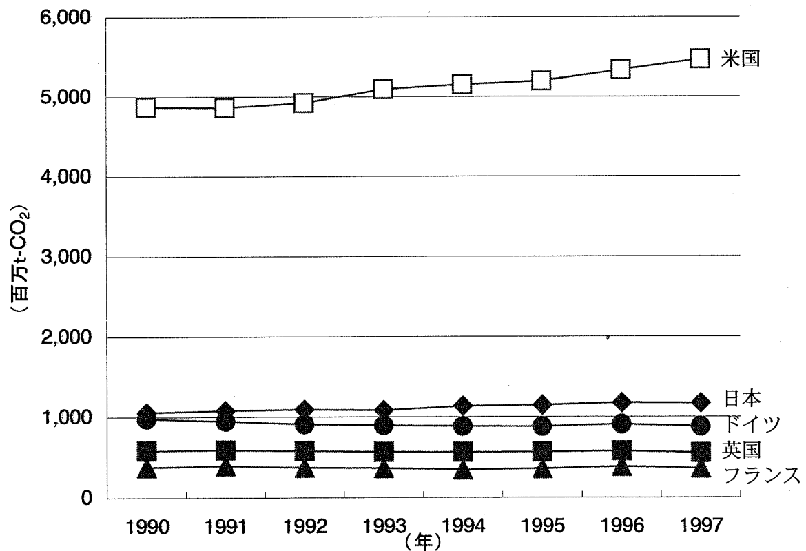
図2 各国の二酸化炭素排出量の推移
