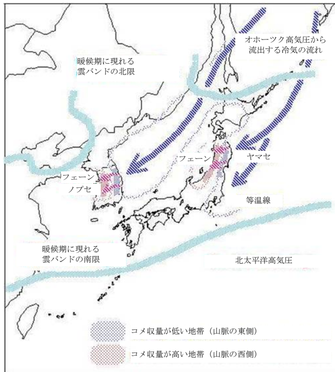
図 2-13 日本と韓半島における寒冷気流の同時流入 (林ほか, 2000a ; 林ほか, 2000b)
