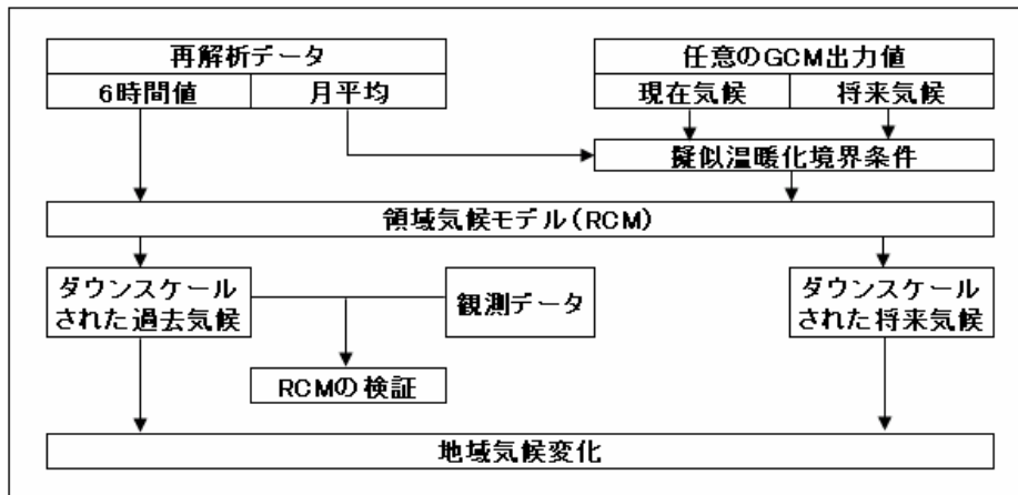
図 2-9 擬似温暖化法によるダウンスケーリングのフローチャート (Kimura and Kitoh, 2007 より改変)
