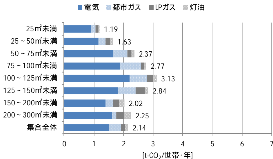
図 1-32 建て方別延べ床面積別世帯当たり年間エネルギー種別 CO 2 排出量（集合） （注 1）125 m 2 以上の区分の集計世帯数は 10 件以上 20 件未満である。 （注 2）300 m 2 以上は集計世帯数が 10 未満のため表示していない。
