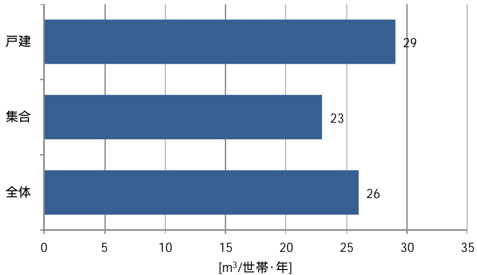
図 1-53 建て方別世帯当たり年間LPガス消費量(固有単位)
