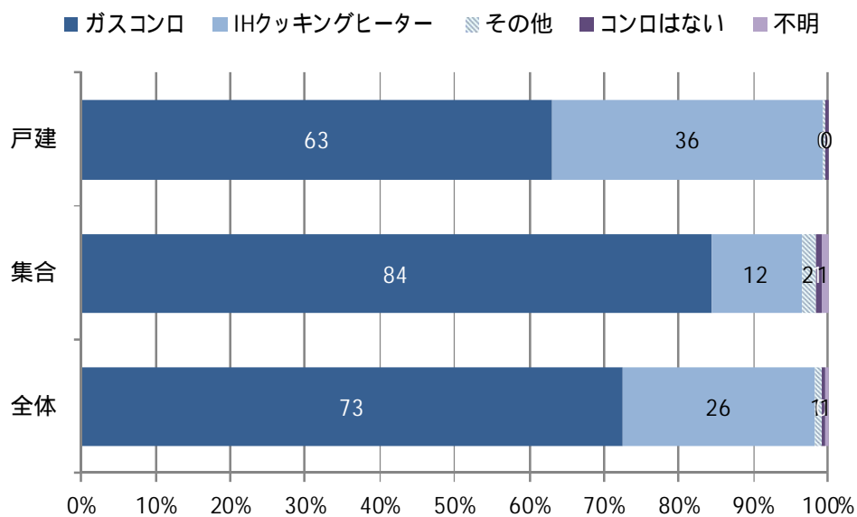
図 1-64 建て方別台所用コンロ
