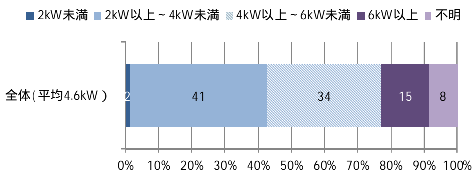
図 1-66 太陽電池の総容量
