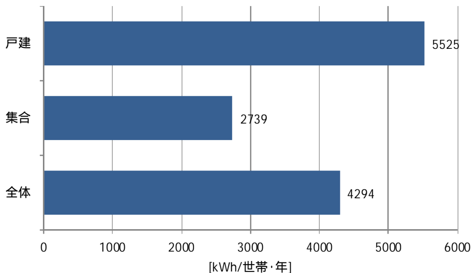
図 1-51 建て方別世帯当たり年間電気消費量（固有単位）
