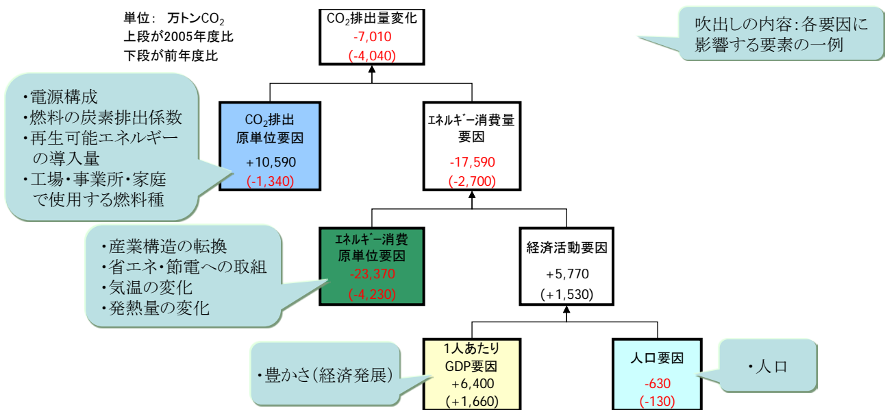
図 2-20 エネルギー起源 CO 2 排出量の増減要因 (2015 年度)
