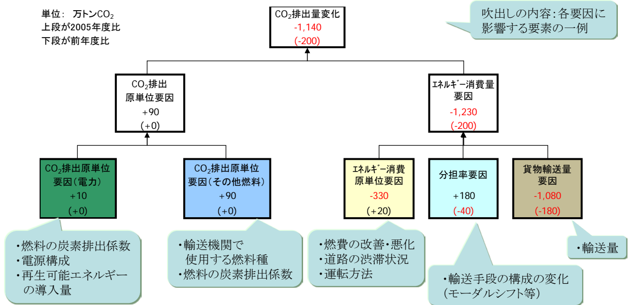
図 2-26 貨物部門のCO 2 排出量増減要因(電気・熱配分後)(2015年度)
