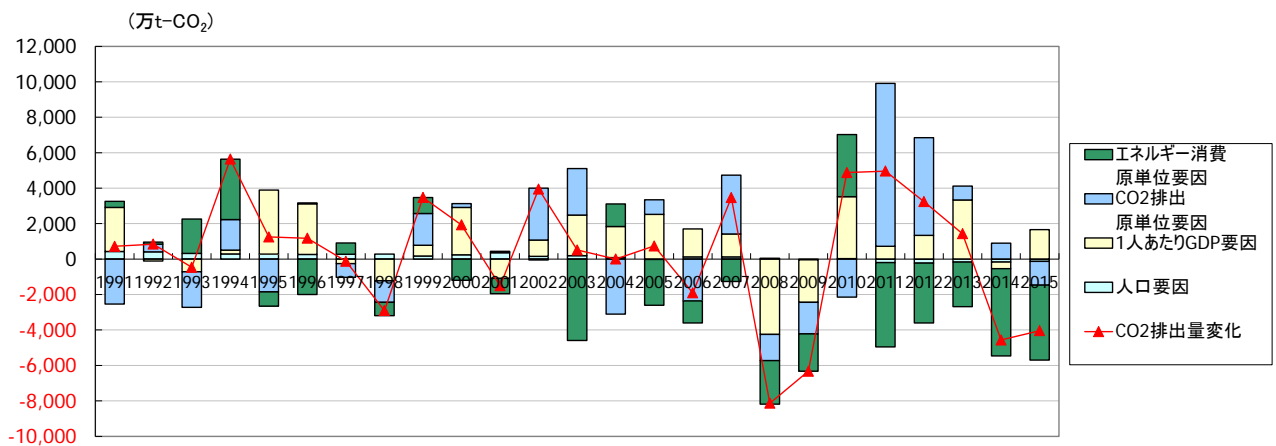
図 2-21 エネルギー起源 CO 2 排出量の増減要因の推移
