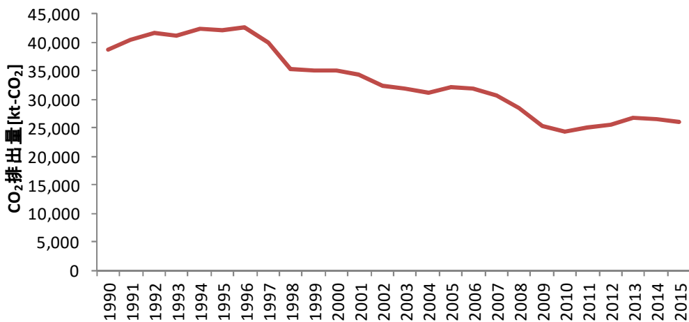
図 1 セメント製造からのCO 2 排出量の推移
