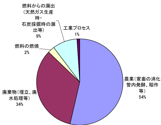
CH 4 総排出量 1990年度 (平成2年度) 3,340万トン (CO 2 換算)
