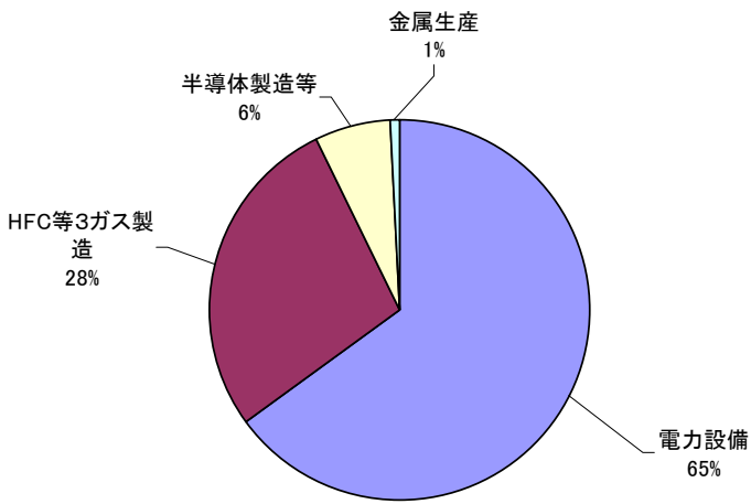
SF 6 総排出量 1995年 (平成7年) 1,690万トン (CO 2 換算)
