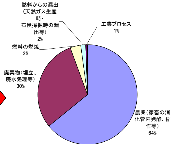
CH 4 総排出量 (速報) 2005年度 (平成17年度) 2,420万トン (CO 2 換算)
