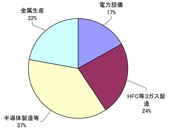
SF 6 総排出量 (速報) 2005年 (平成17年) 410万トン (CO 2 換算)
