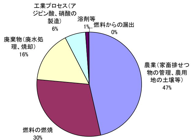
N 2 O総排出量 (速報) 2005年度 (平成17年度) 2,580万トン (CO 2 換算)
