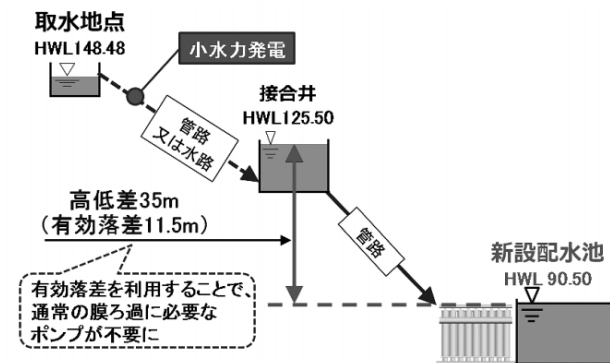
図 有効落差を利用するイメージ
