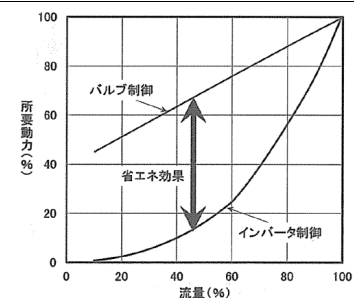
図 インバーターによる省エネ効果のイメージ
