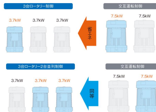
台数制御のイメージ 小水量時（上）と大水量時（下） [3]
